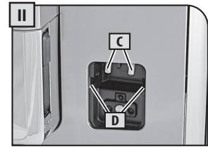
C = Embrayages machine D = Glissières pour les pivots de la carafe
