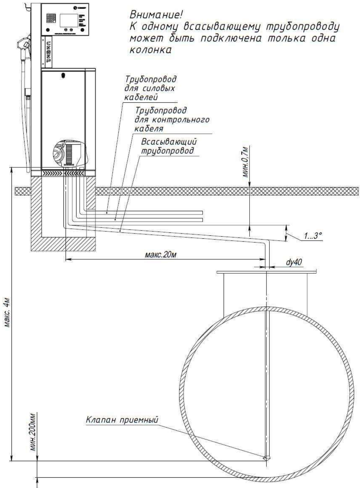
Пример устройства коммуникаций для колонки «СЕВЕР-211-50 ЖКИ» Рисунок Б.1
