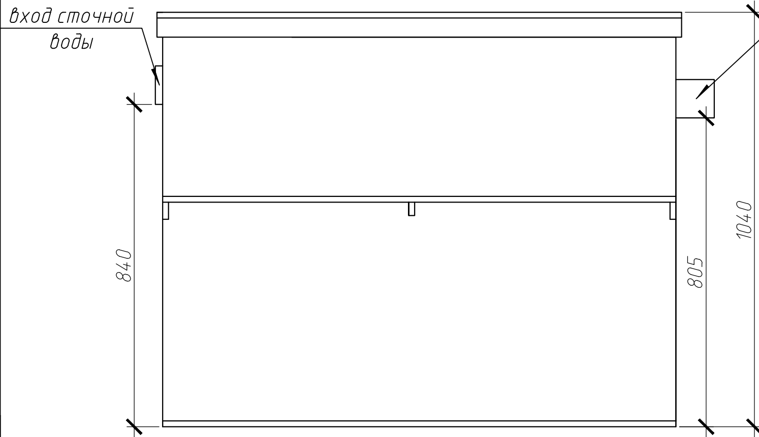
Вид сбоку
