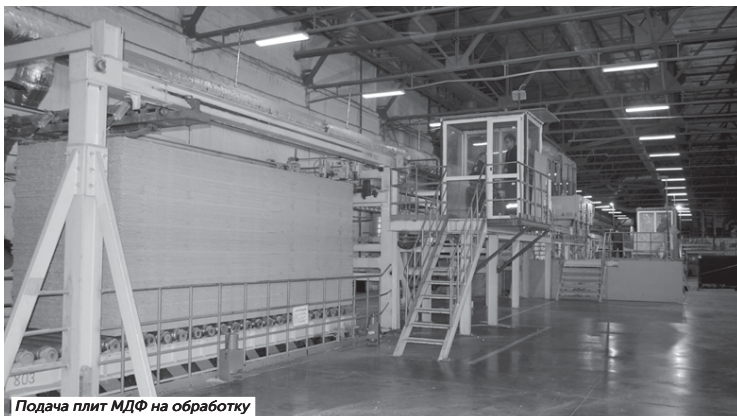
Подача плит МДФ на обработку
