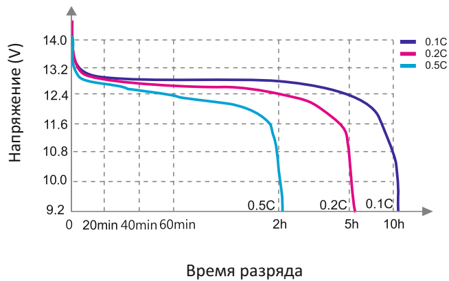
Кривая разряда с разной скоростью (25 °C)
