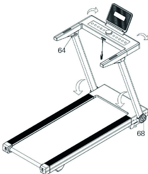
Рисунок 5 — Складывание беговой дорожки
