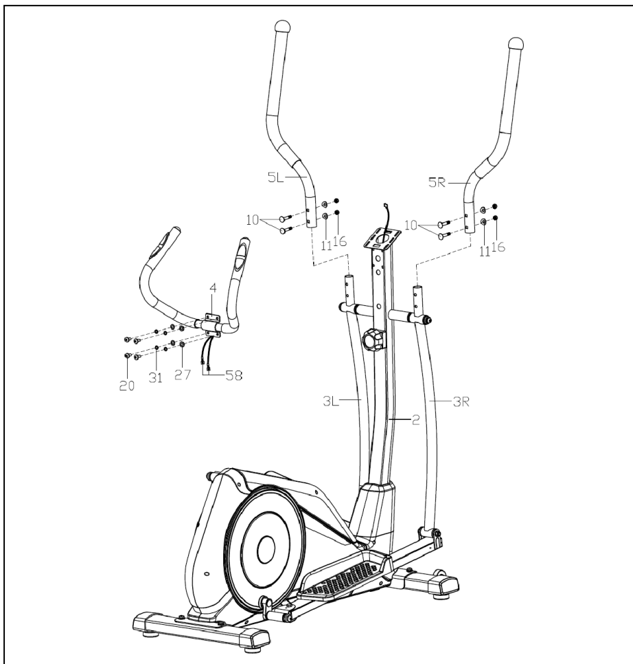
Рисунок 6 – Установка ручек
