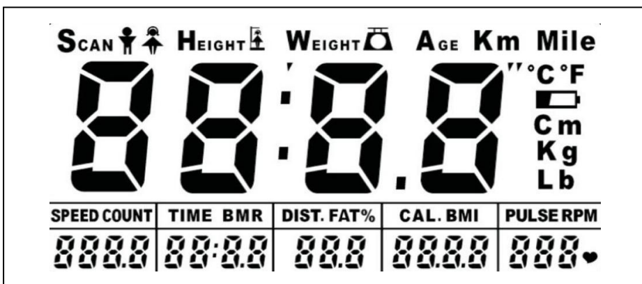
Рисунок 10 – Экран консоли
