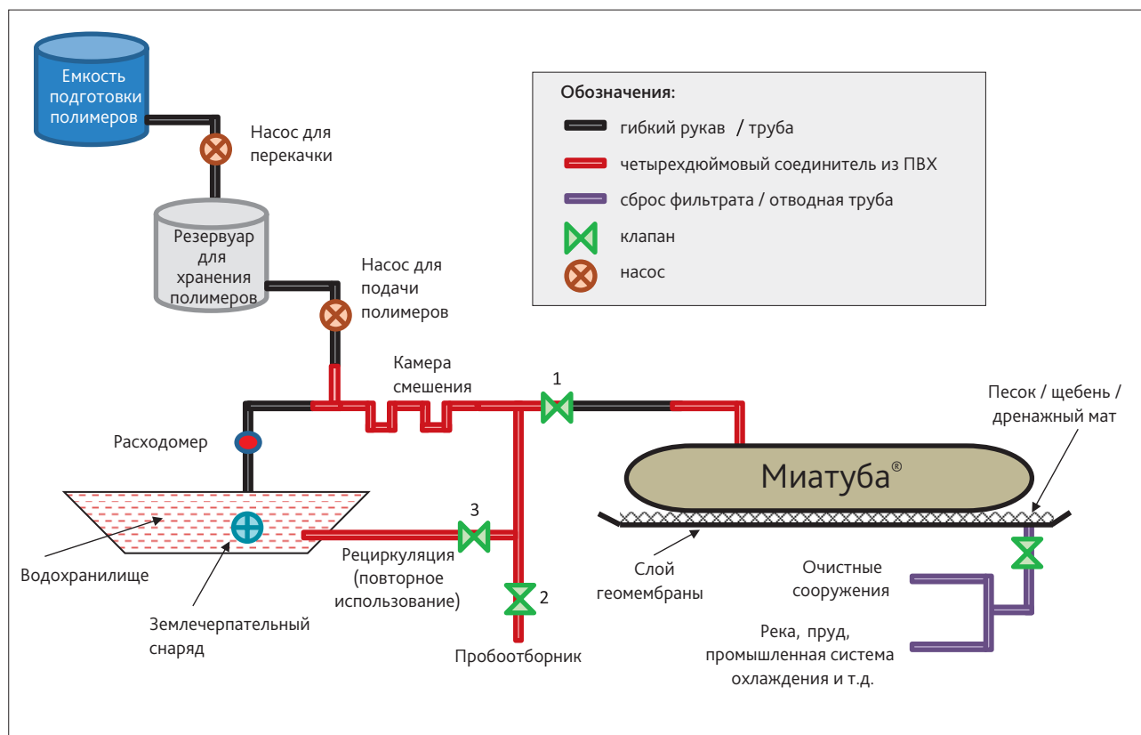
Схема процесса обезвоживания донного осадка
