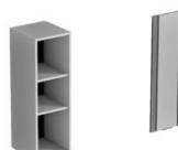
ВСФ 300 корпус В 300: 300x900x350 мм фасад ВСФ 300: 296x896 мм
