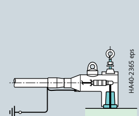
Прокладка кабеля назад с угловым кабельным адаптером
