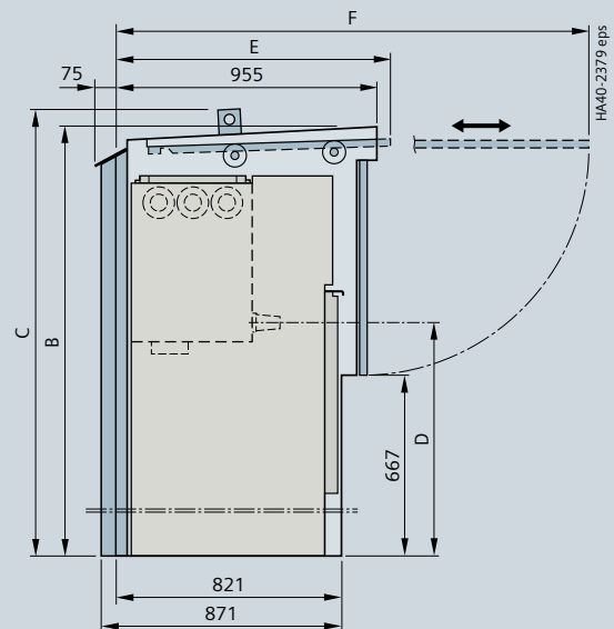
Корпус для наружной установки со сбросом давления вверх
