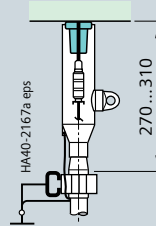
Прокладка кабеля вниз с прямым адаптером
