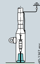
Прокладка кабеля вверх с прямым адаптером
