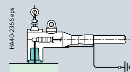
Прокладка кабеля вправо с угловым кабельным адаптером
