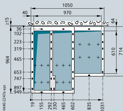
Тип RRT с углублением на 250 мм
