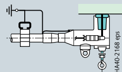
Прокладка кабеля назад с угловым кабельным адаптером
