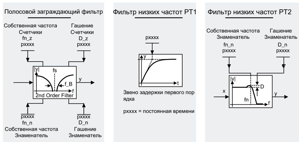
Рисунок 4-2 Обзор фильтров – Фильтры заданного значения частоты вращения
