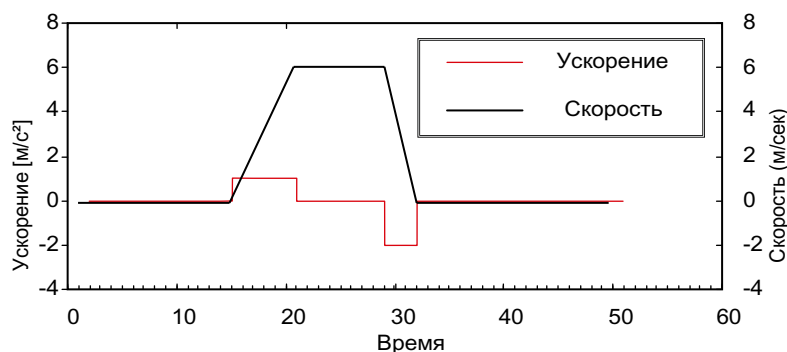
Рисунок 8-16 Без ограничения рывка
