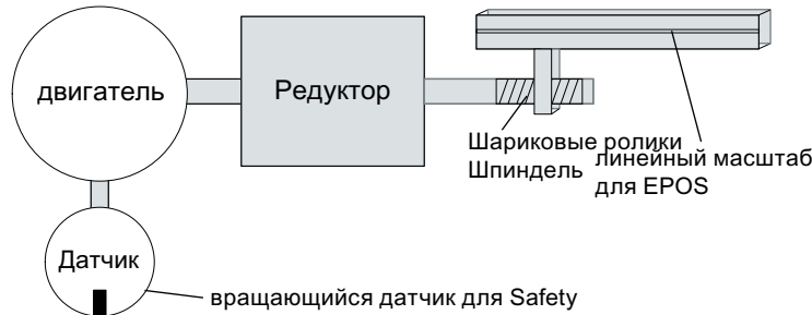
Рисунок 8-22 Пример 2: EPOS и безопасное реферирование_линейное
