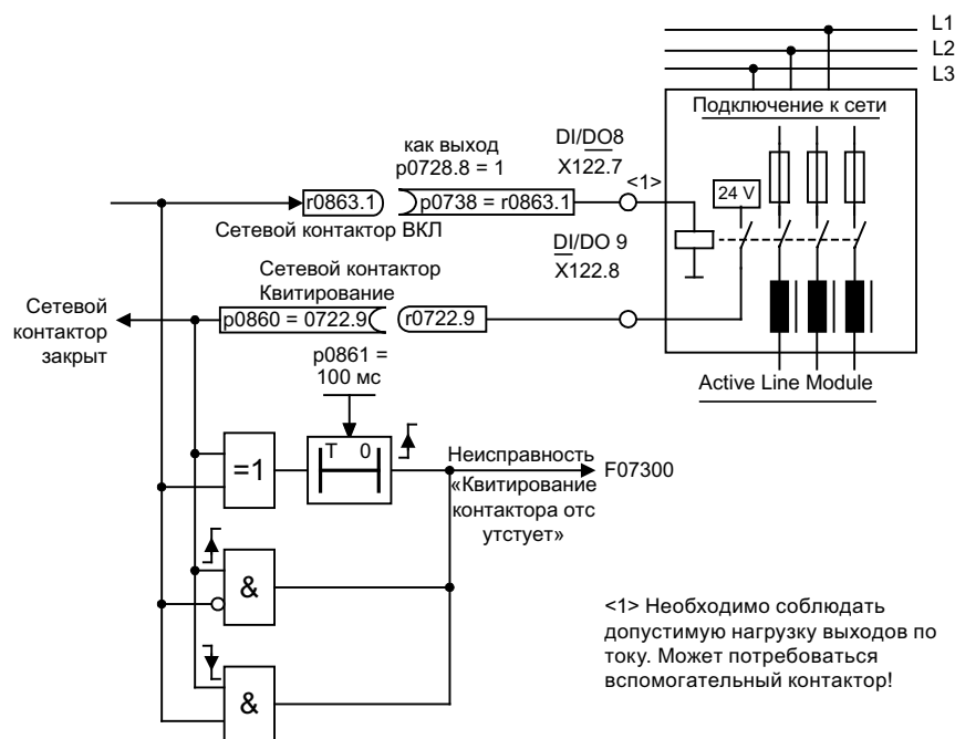
Рисунок 2-10 Управление сетевым контактором
