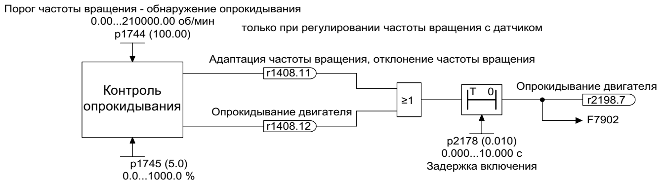
Рисунок 9-3 Защита от опрокидывания
