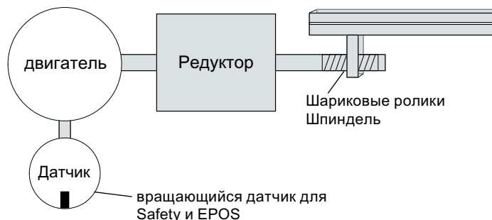
Рисунок 8-23 Пример 3: EPOS и безопасное реферирование_линейное
