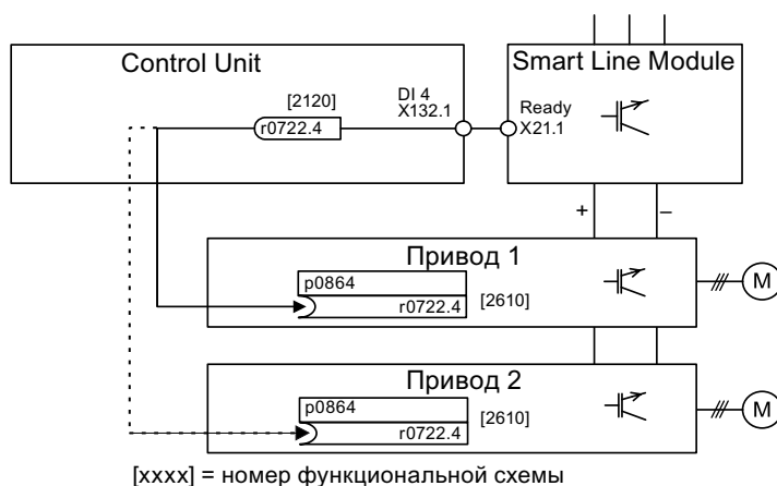
Рисунок 11-3 Иллюстративное соединение модуля питания Smart без DRIVE-CLiQ
