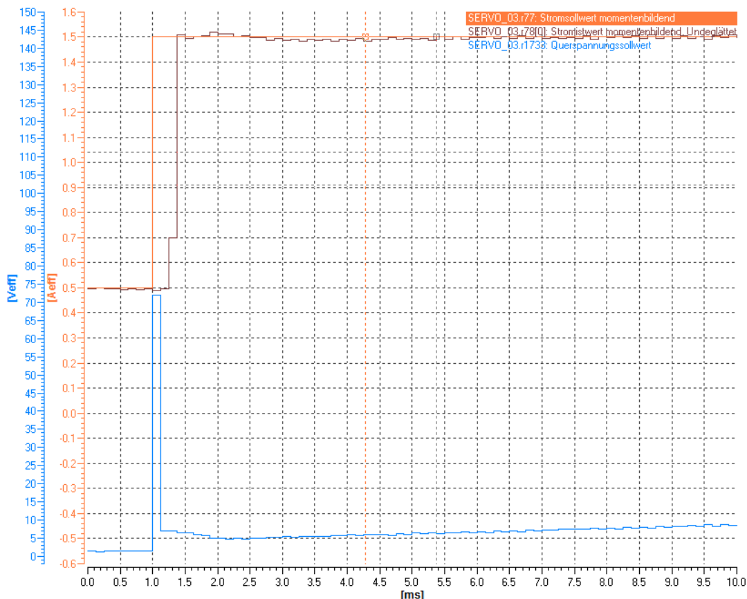
Рисунок 4-42 Пример: после оптимизации
