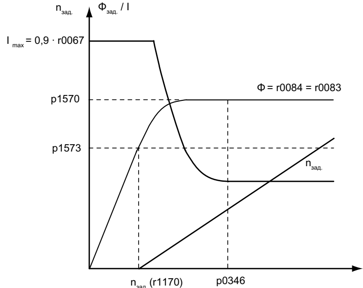
Рисунок 5-23 Характеристики для быстрого намагничивания
