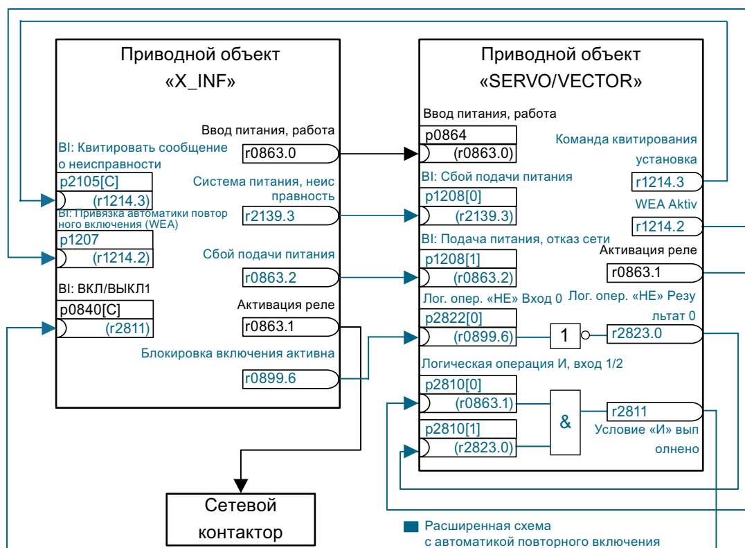
Рисунок 11-2 Схема BICO: Включение устройства питания через привод дополнительно с автоматикой повторного включения
