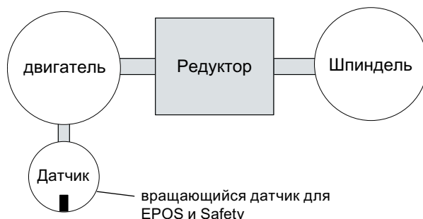
Рисунок 8-21 Пример 1: EPOS и безопасное реферирование_круговое
