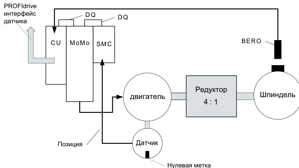
Рисунок 8-19 Конструкция с редуктором между двигателем и шпинделем
