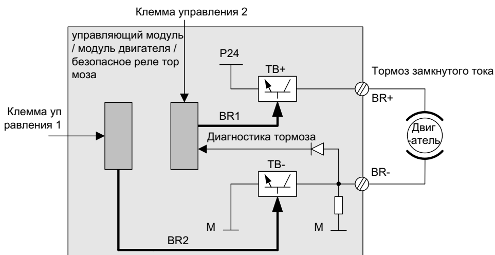
Рисунок 10-1 Двухканальное управление торможением блочного формата (пример)
