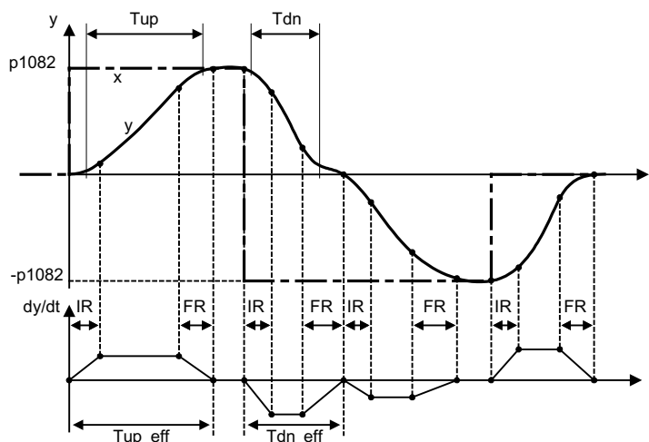
Рисунок 3-9 Расширенный задатчик интенсивности
