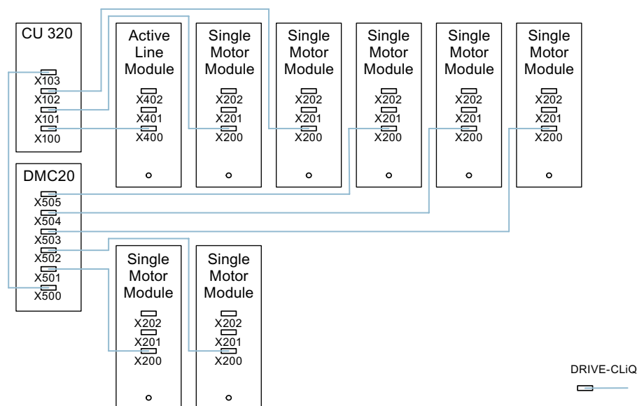
Рисунок 11-9 Иллюстративная топология Hot-Plugging для векторного управления U/f
