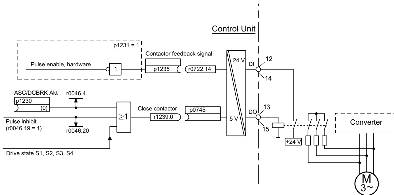
Рисунок 7-4 Пример внешнего торможения закорачиванием якоря
