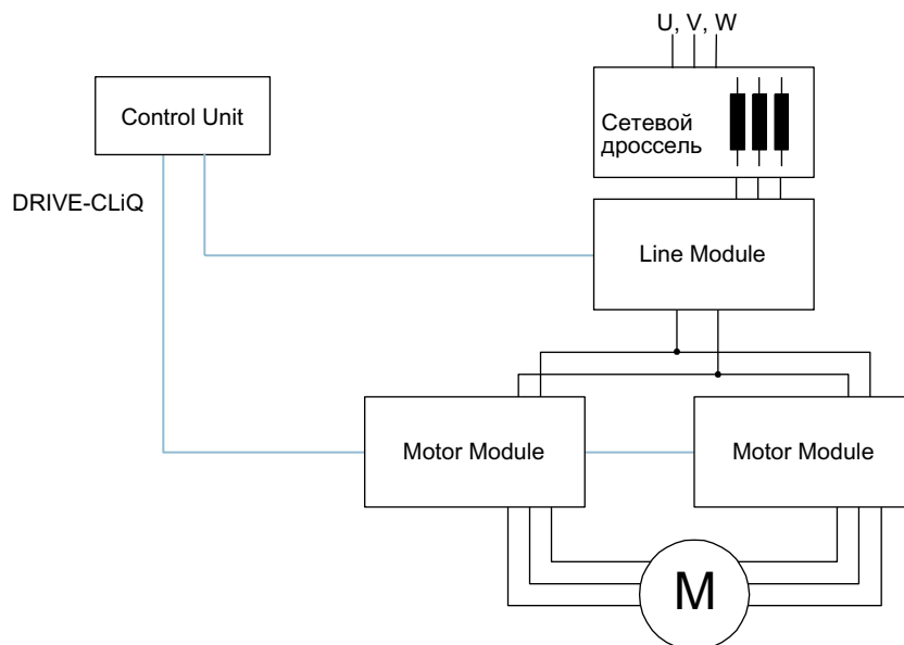
Рисунок 8-27 Параллельное включение двух модулей двигателя на один двигатель с двухобмоточной системой
