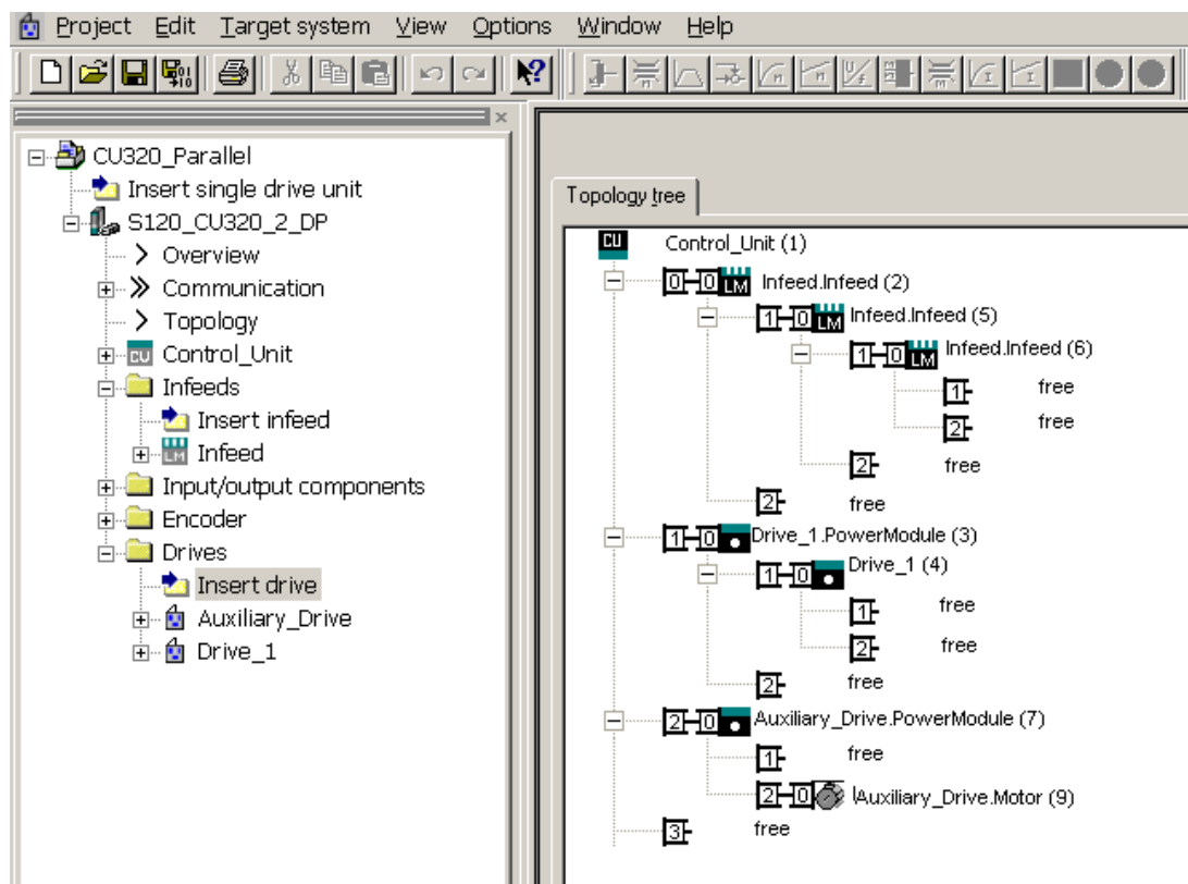
Рисунок 8-28 Топология с 3 модулями питания Basic, 2 модулями двигателей и 1 вспомогательным приводом
