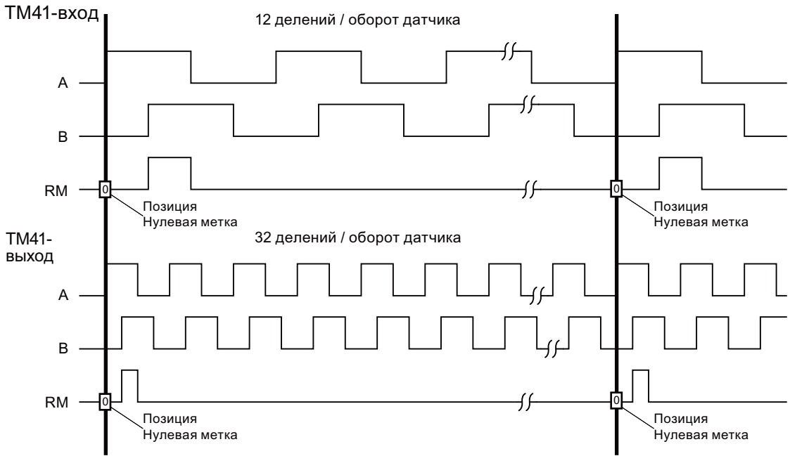
Рисунок 7-20 Пересчет числа делений датчика
