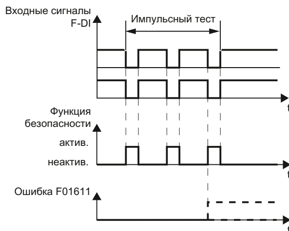
Рисунок 10-5 Реакция преобразователя на импульсный тест
