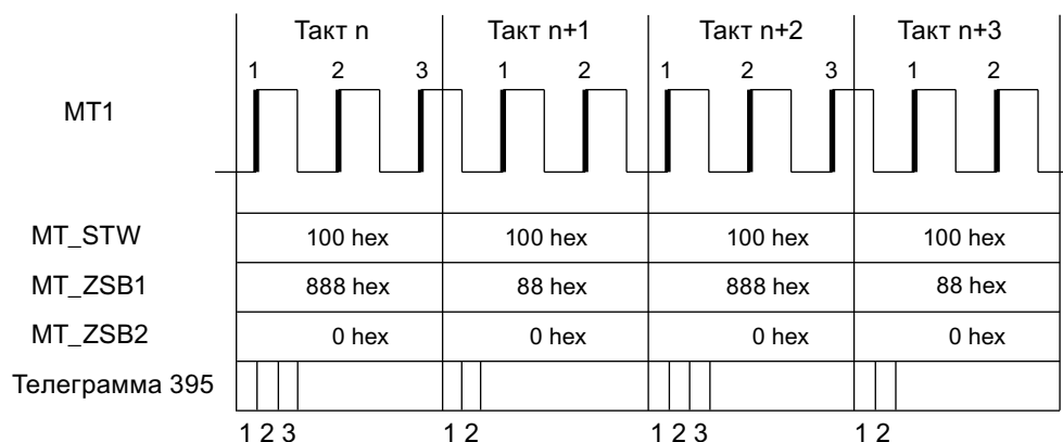
Рисунок 4-32 поиск передних фронтов для щупа 1
