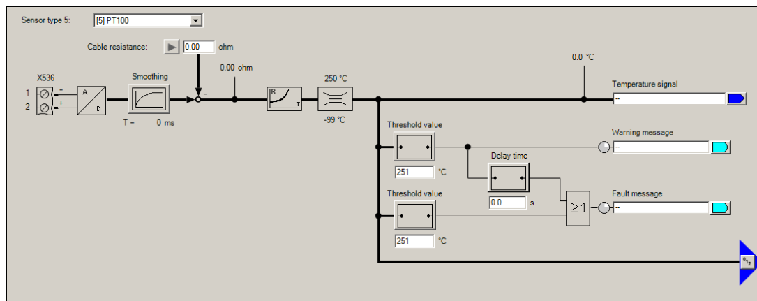
Рисунок 9-1 Время сглаживания датчика/канала температуры
