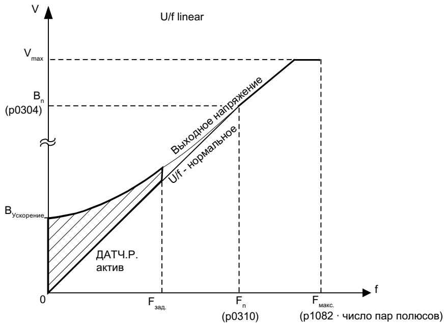
Рисунок 6-4 Вольтодобавка при разгоне (пример: p1300 = 0 и p1311 > 0)
