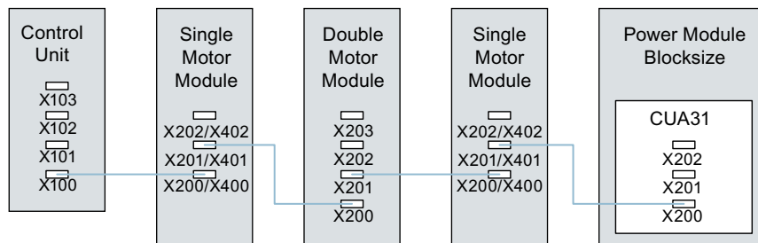
Рисунок 13-22 Пример линии DRIVE-CLiQ
