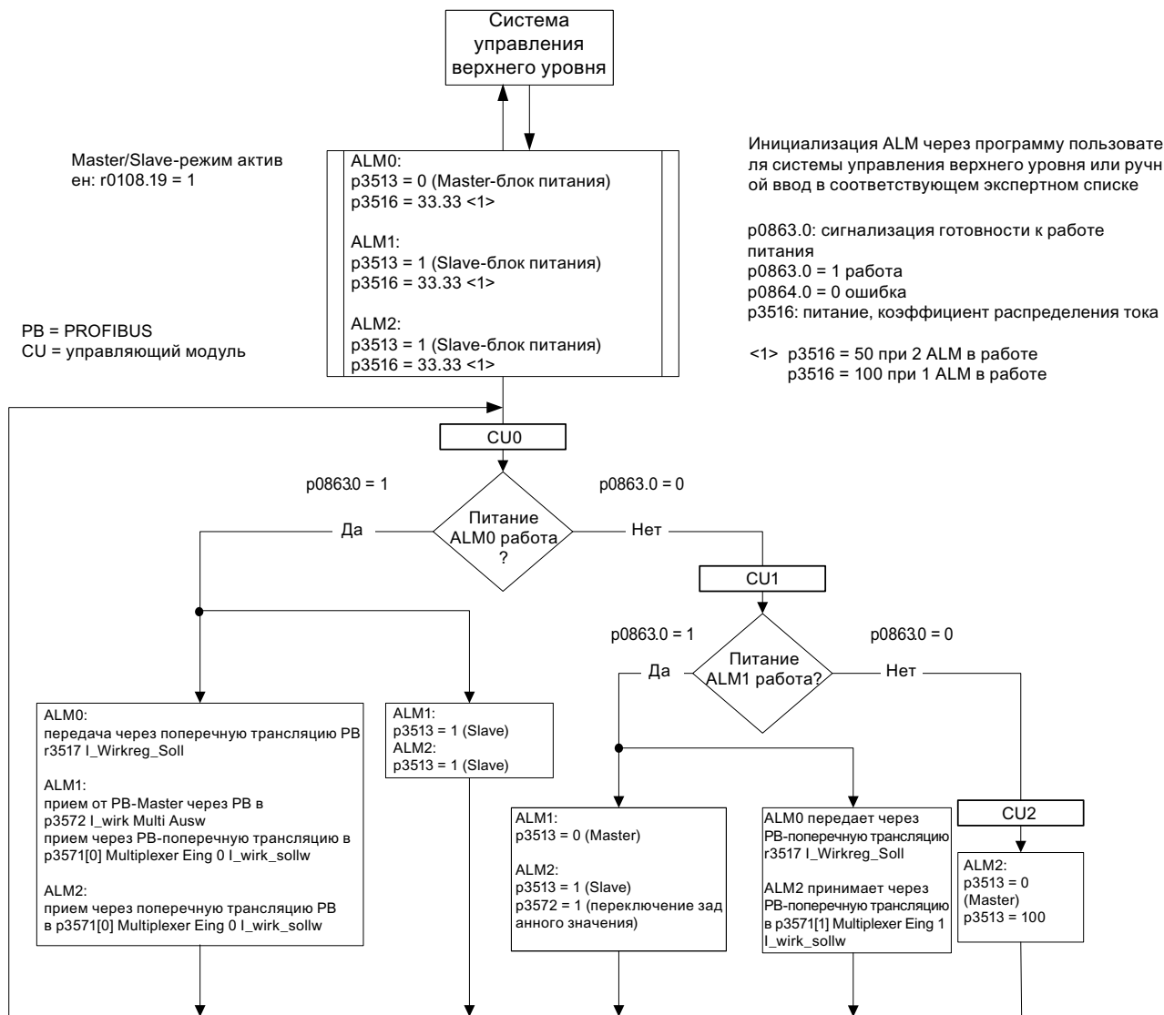
Рисунок 8-25 Структурограмма режима Master/Slave, 3 идентичных активных модуля питания (ALM) одной мощности, вариант коммуникации PROFIBUS
