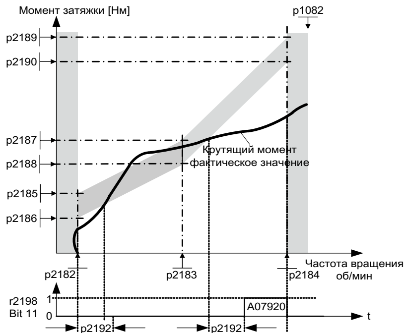
Рисунок 8-3 Контроль нагрузки
