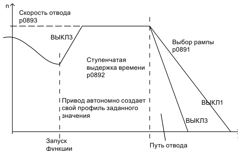
Рисунок 8-30 Рампа ВЫКЛ с «Расширенным отводом»
