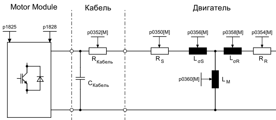
Рисунок 4-19 Эквивалентная схема - Асинхронный двигатель и кабель
