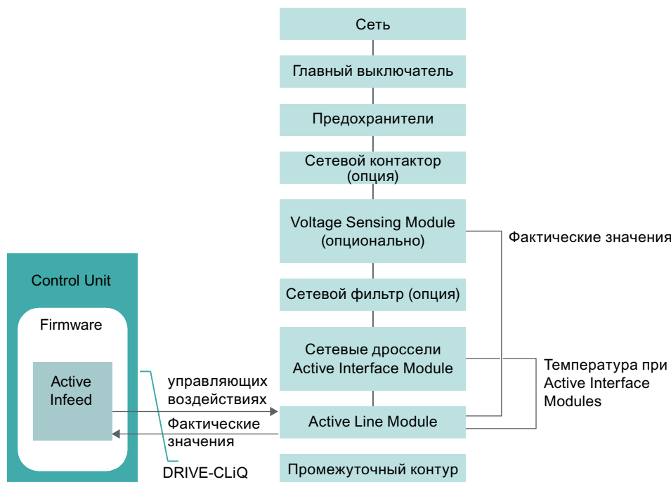
Рисунок 2-1 Схематическая структура активного питания книжного формата
