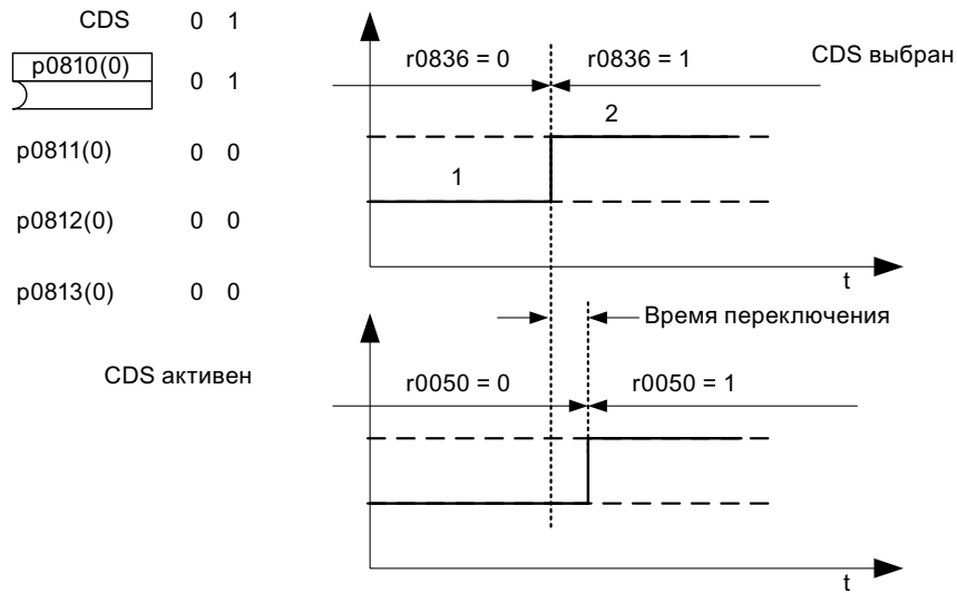
Рисунок 13-12 Переключение командного блока данных (пример)
