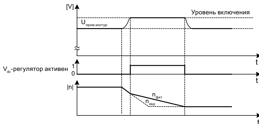
Рисунок 6-9 Включение/выключение V_{dc\_max} -регулирования
