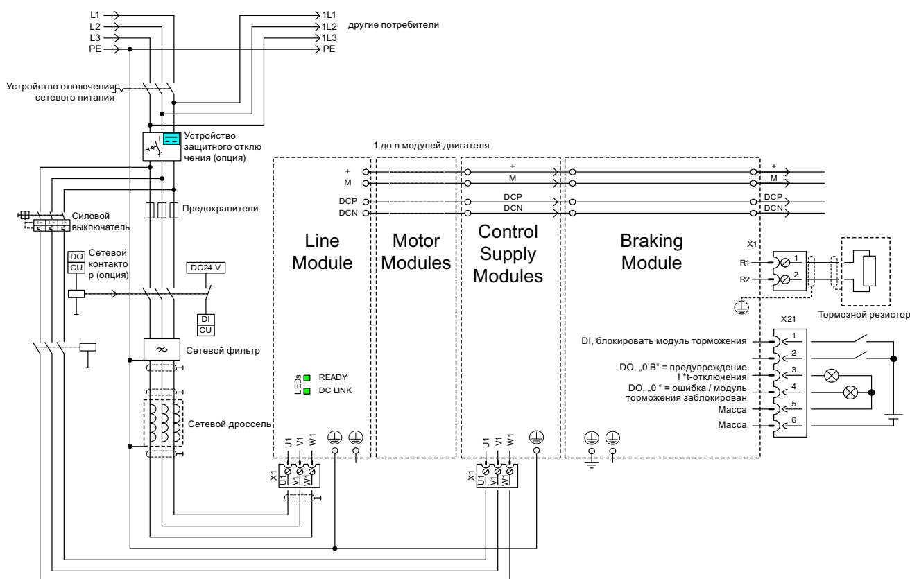
Рисунок 11-5 Иллюстративное соединение быстрого останова при выпадении сети или аварийном выключении
