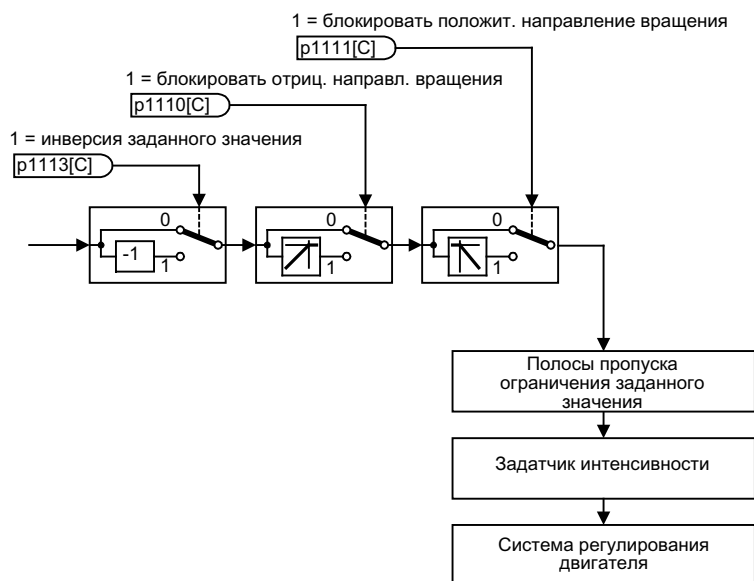
Рисунок 3-6 Ограничение направления вращения, реверсирование
