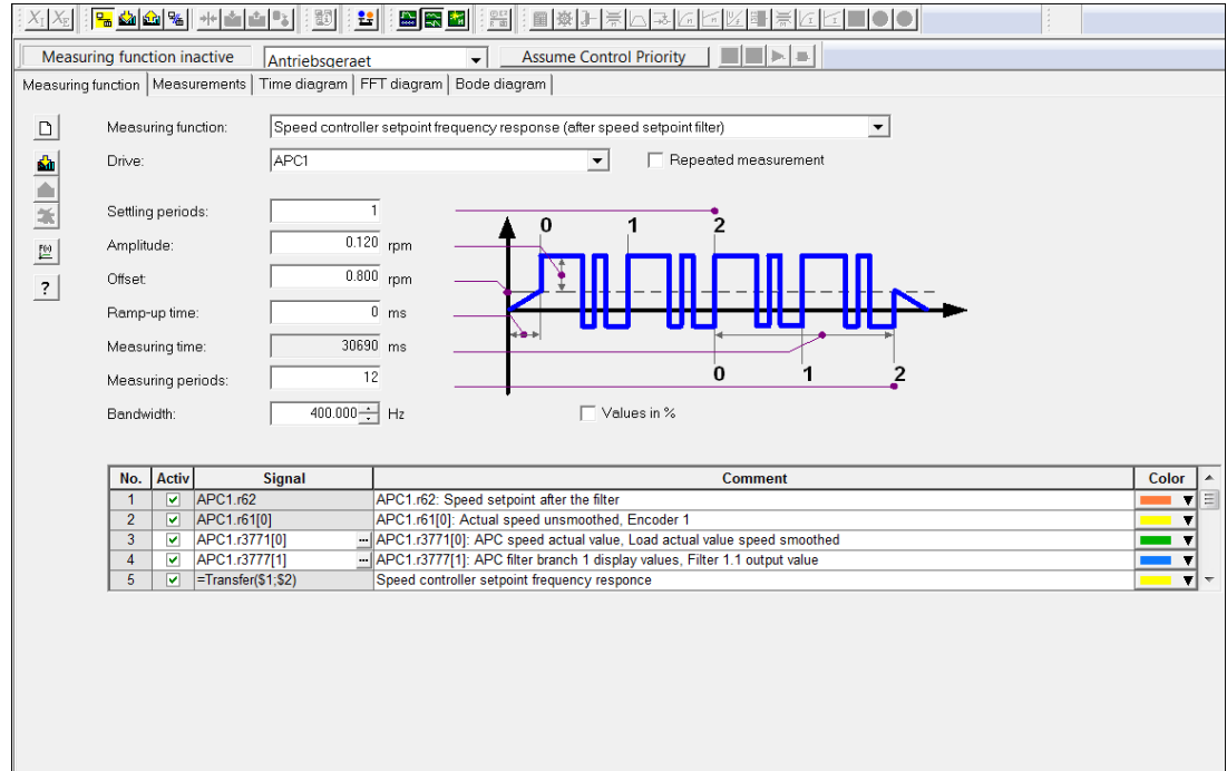
Рисунок 8-51 Измерительная функция и сигналы
