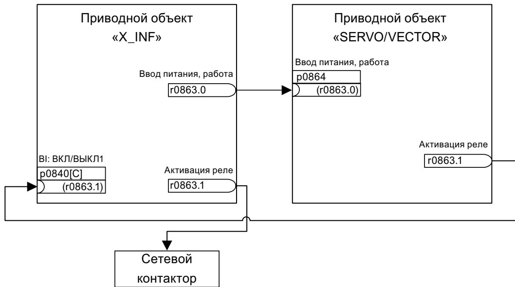
Рисунок 11-1 Схема BICO: Включение устройства питания через привод
