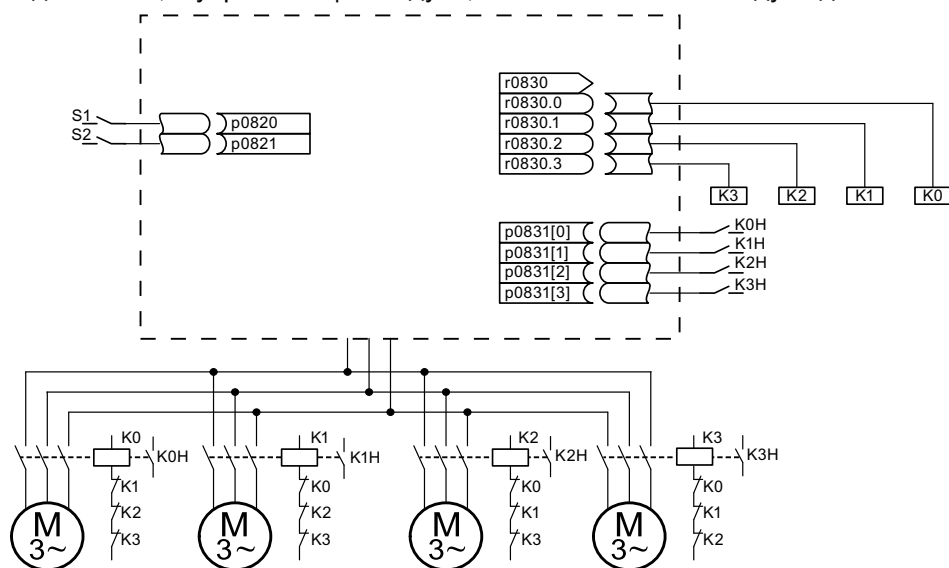
Рисунок 11-6 Пример переключения двигателей
