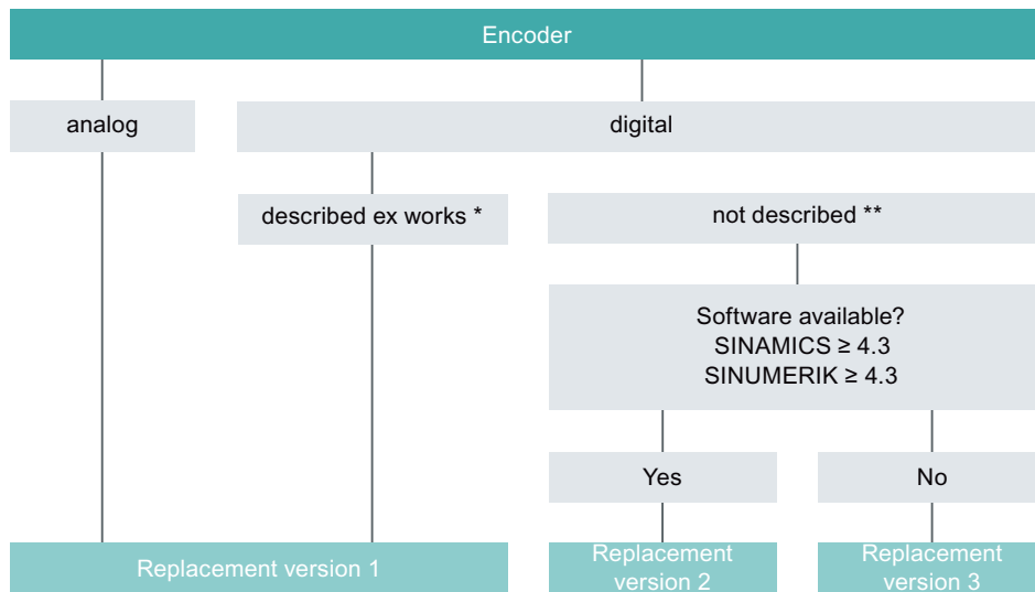
Рисунок A-16 Варианты замены датчика
