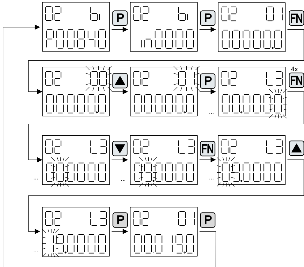
Рисунок А-13 Пример: Изменение отображенного параметра бинектора
