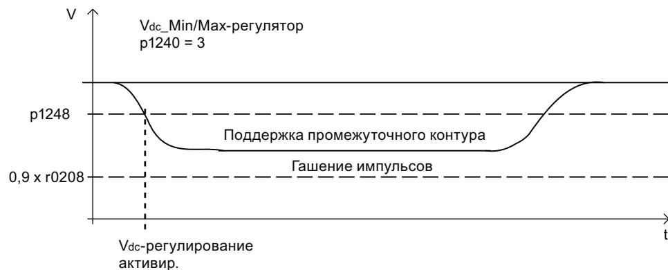
Рисунок 8-32 Заданное значение напряжения промежуточного контура
