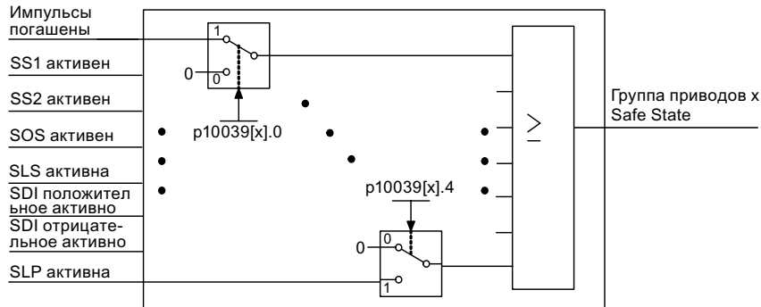
Рисунок 10-7 Выбор Safe State (пример Extended Functions)
