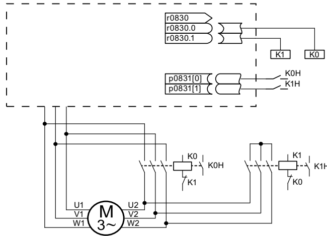
Рисунок 11-7 Пример переключения звезда / треугольник
