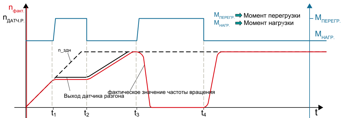
Рисунок 3-11 Стандартное слежение за задатчиком интенсивности
