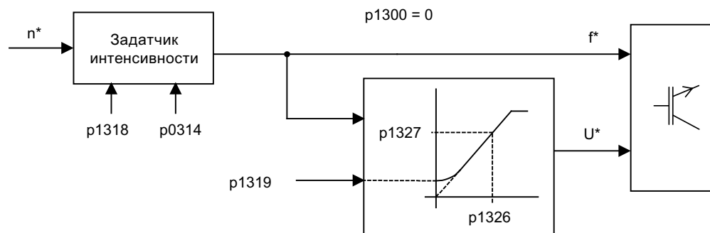
Рисунок 4-15 Структура управления U/f
