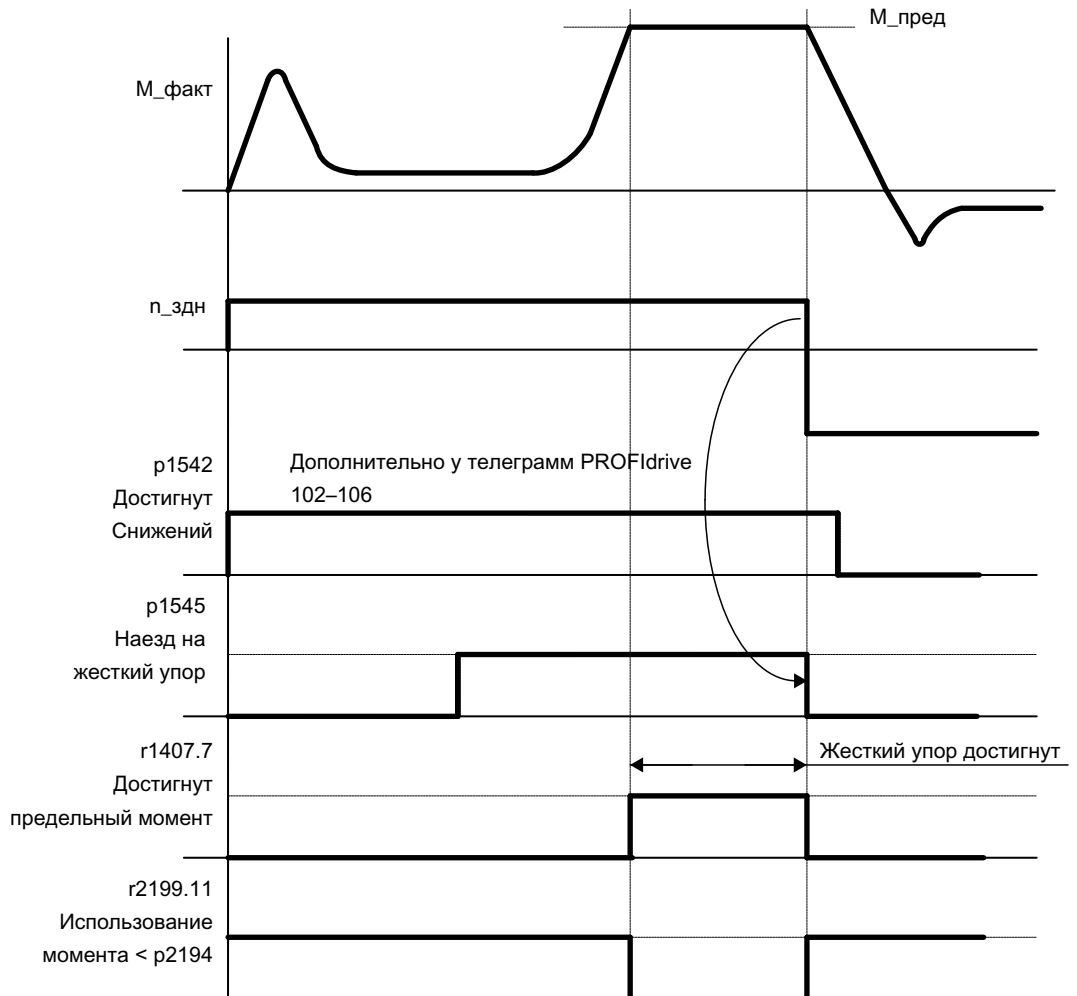
Рисунок 4-30 Характеристика сигнала при «Наезде на жесткий упор»
