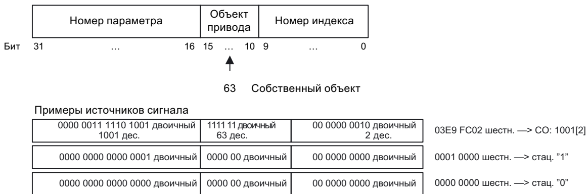
Рисунок 13-9 Внутренняя кодировка выходных параметров бинекторов/коннекторов
