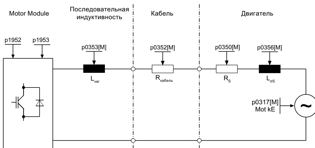
Рисунок 4-20 Эквивалентная схема - Синхронный двигатель и кабель
