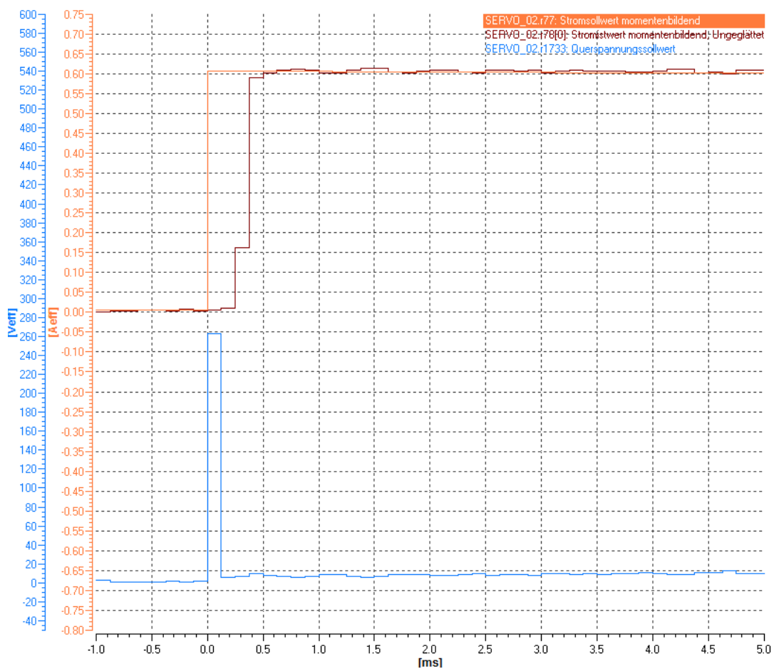
Рисунок 4-38 Предусиление регулирования напряжения р1703 в норме
