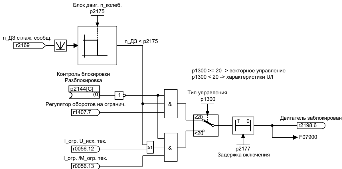
Рисунок 9-2 Защита от блокировки
