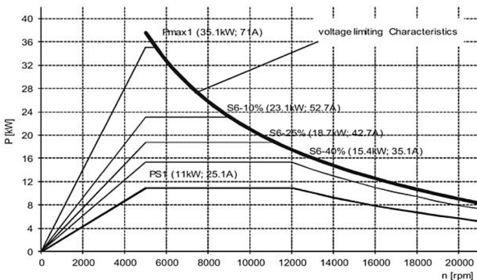
Рисунок 4-13 Асинхронный двигатель: Характеристика мощность-вращающий момент
