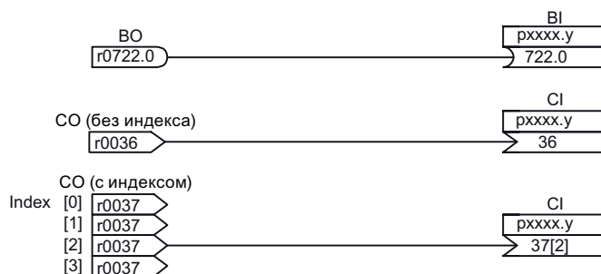
Рисунок 13-8 Соединение сигналов при помощи техники BICO
