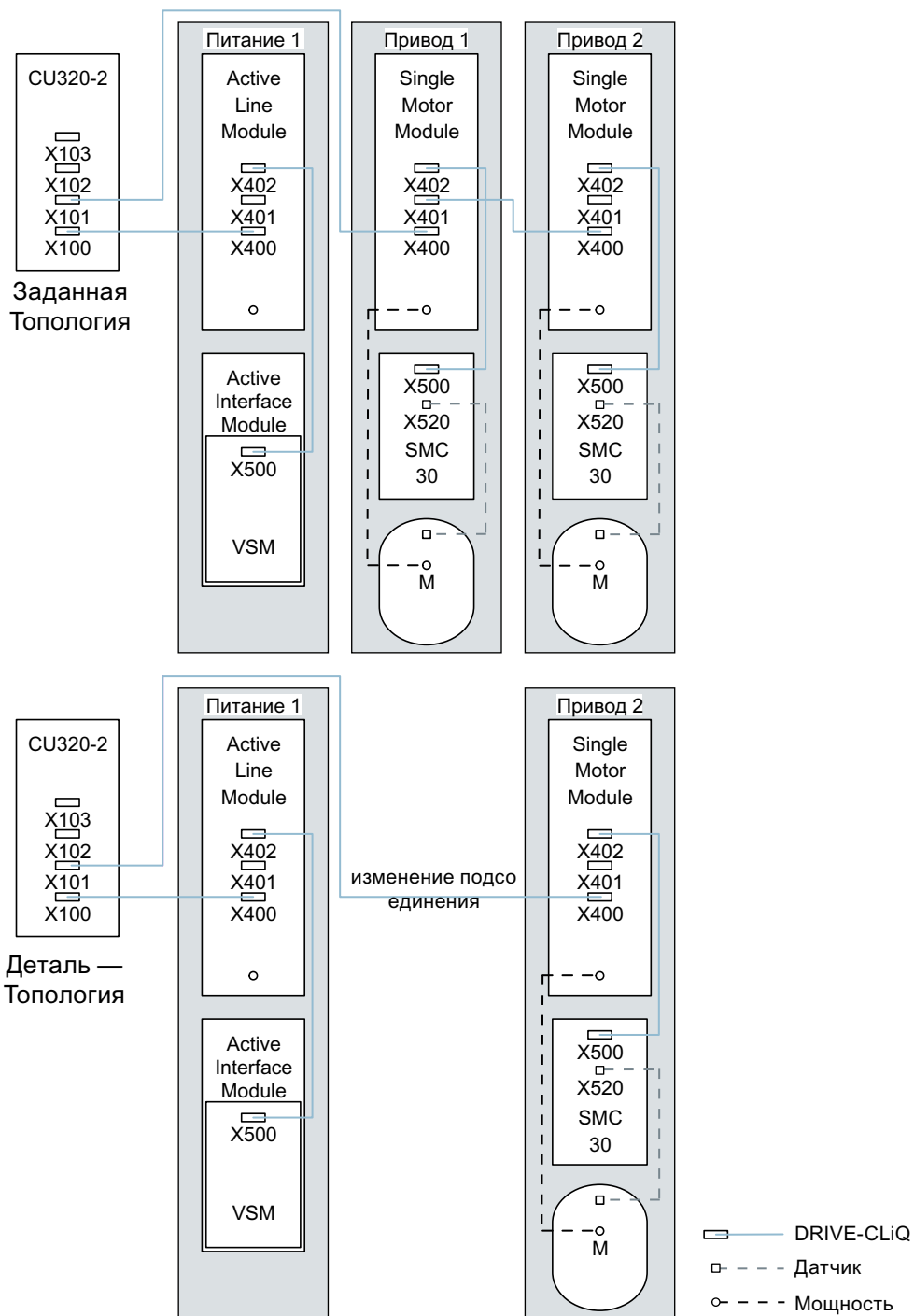
Рисунок 13-24 Пример частичной топологии
