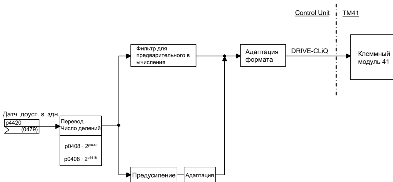
Рисунок 7-19 Эмуляция инкрементального датчика
