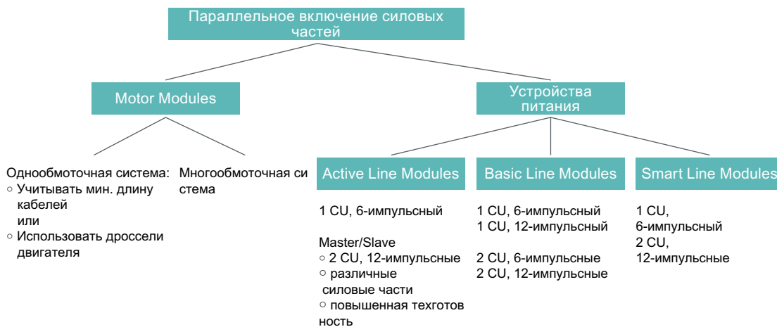
Рисунок 8-26 Обзор: Параллельное включение силовых частей
