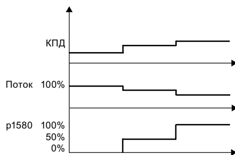
Рисунок 5-22 Простая оптимизация КПД
