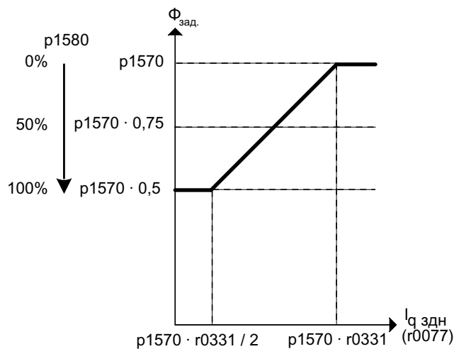
Рисунок 5-21 Оптимизация КПД
