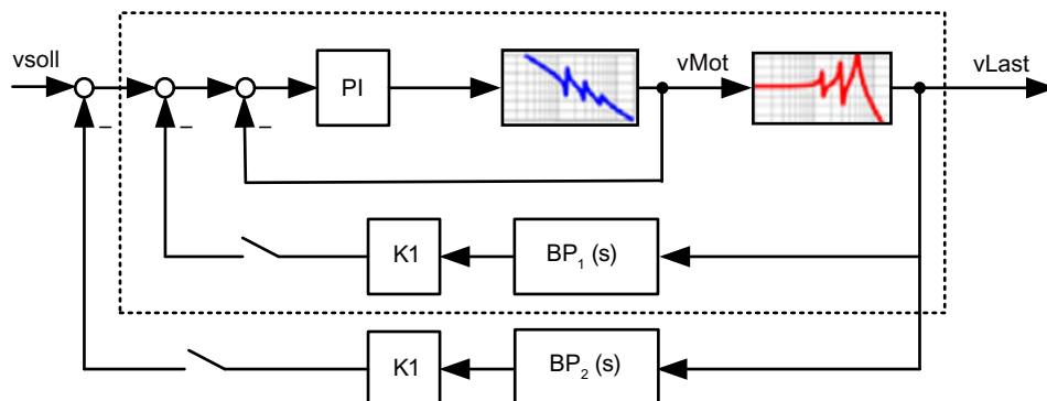
Рисунок 8-47 Регулирующий контур с 2 обратными связями APC
