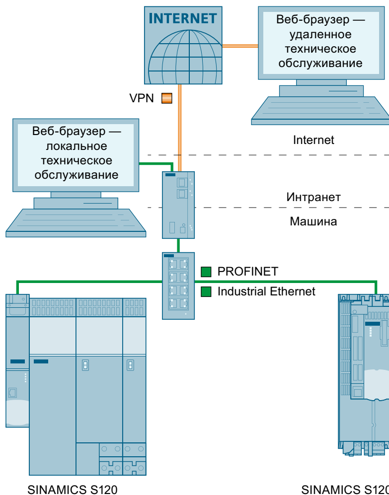
Рисунок 12-1 Структура веб-сервера
