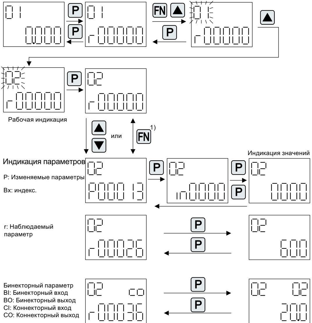
Рисунок А-10 Индикация параметров
