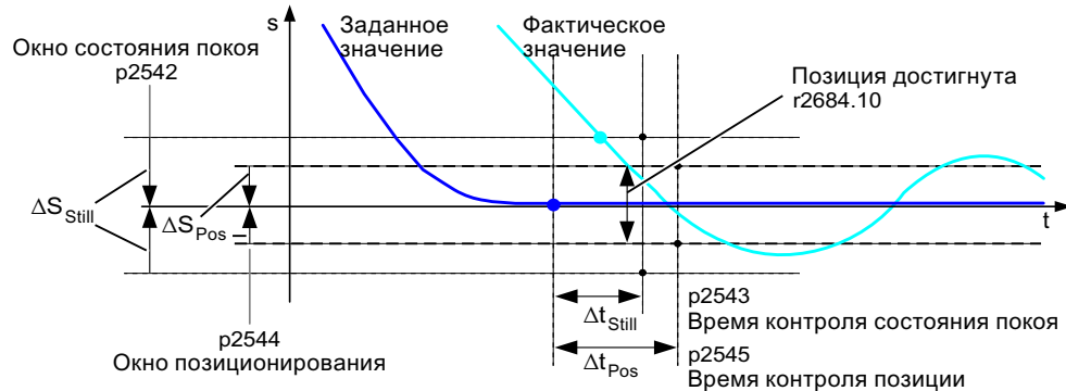
Рисунок 8-10 Контроль состояния покоя, окно позиционирования
