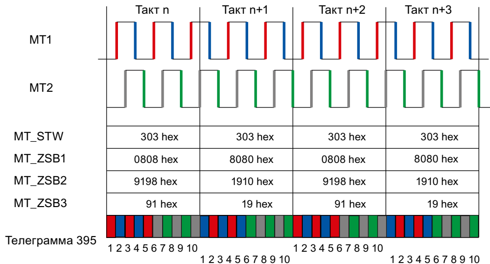
Рисунок 4-34 поиск передних и задних фронтов для щупа 1 и 2
