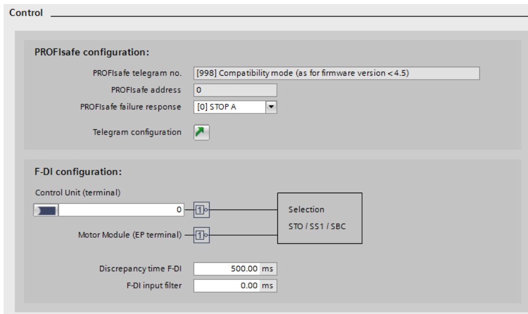
Рисунок 10-9 Пример: Управление STO
