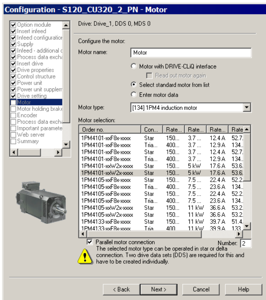
Рисунок 7-24 Выбор параллельного включения двигателей при векторном управлении
