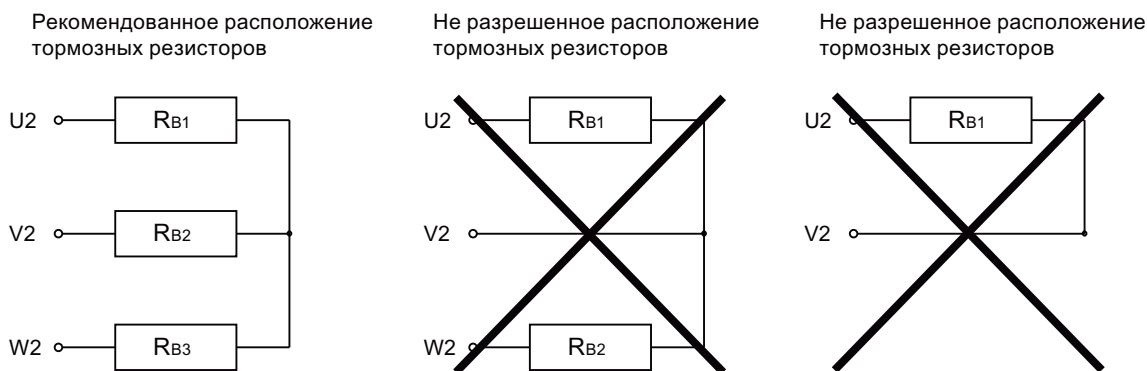
Рисунок 7-5 Тормозные резисторы
