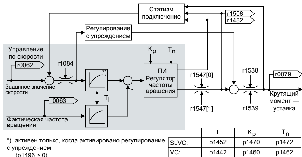
Рисунок 5-6 Регулятор частоты вращения
