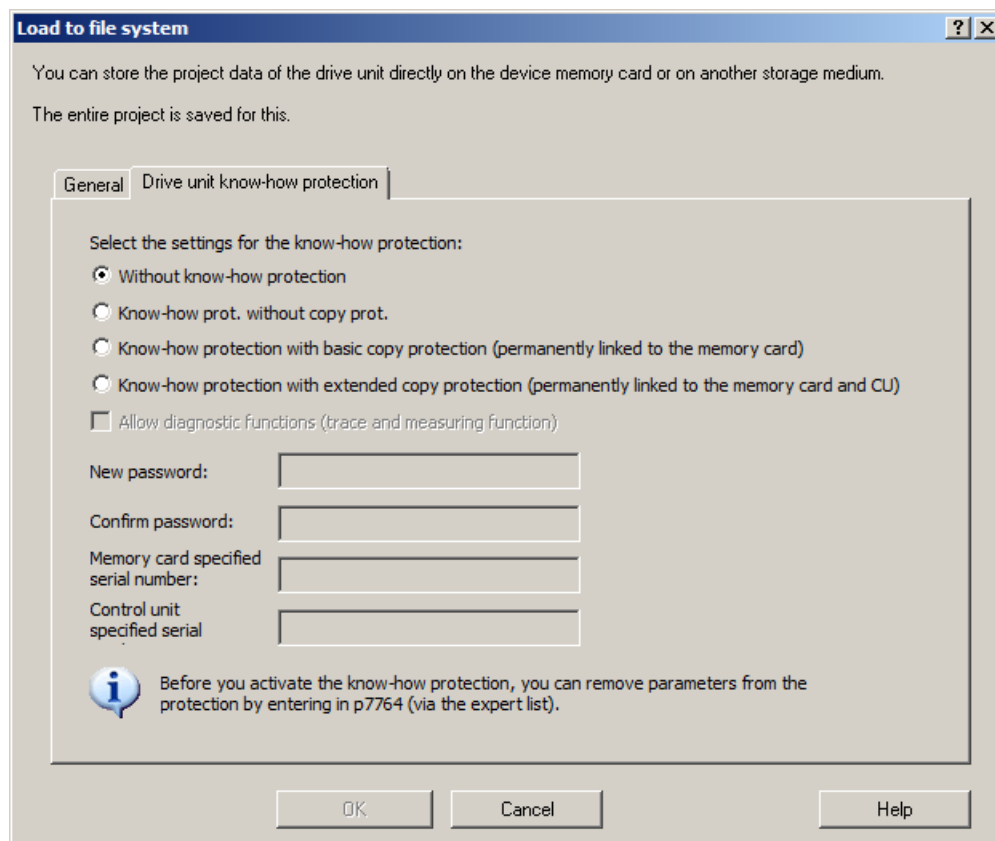
Рисунок 13-20 Загрузка в файловую систему, защита ноу-хау
