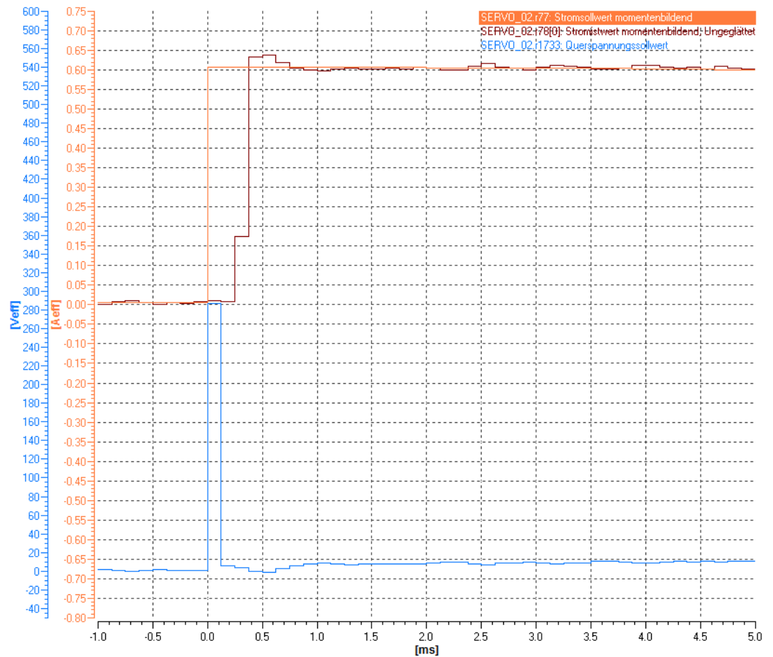
Рисунок 4-39 Предусиление регулирования напряжения p1703 слишком велико
