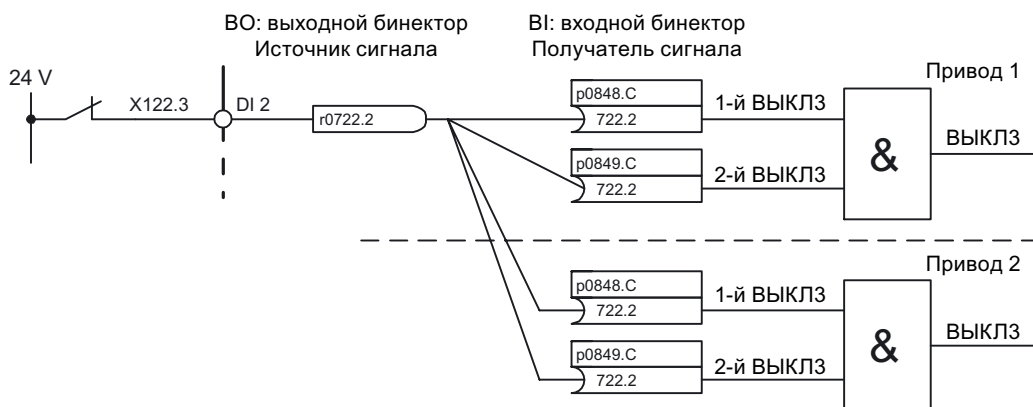
Рисунок 13-11 Соединить ВЫКЛЗ с несколькими приводами (пример)
