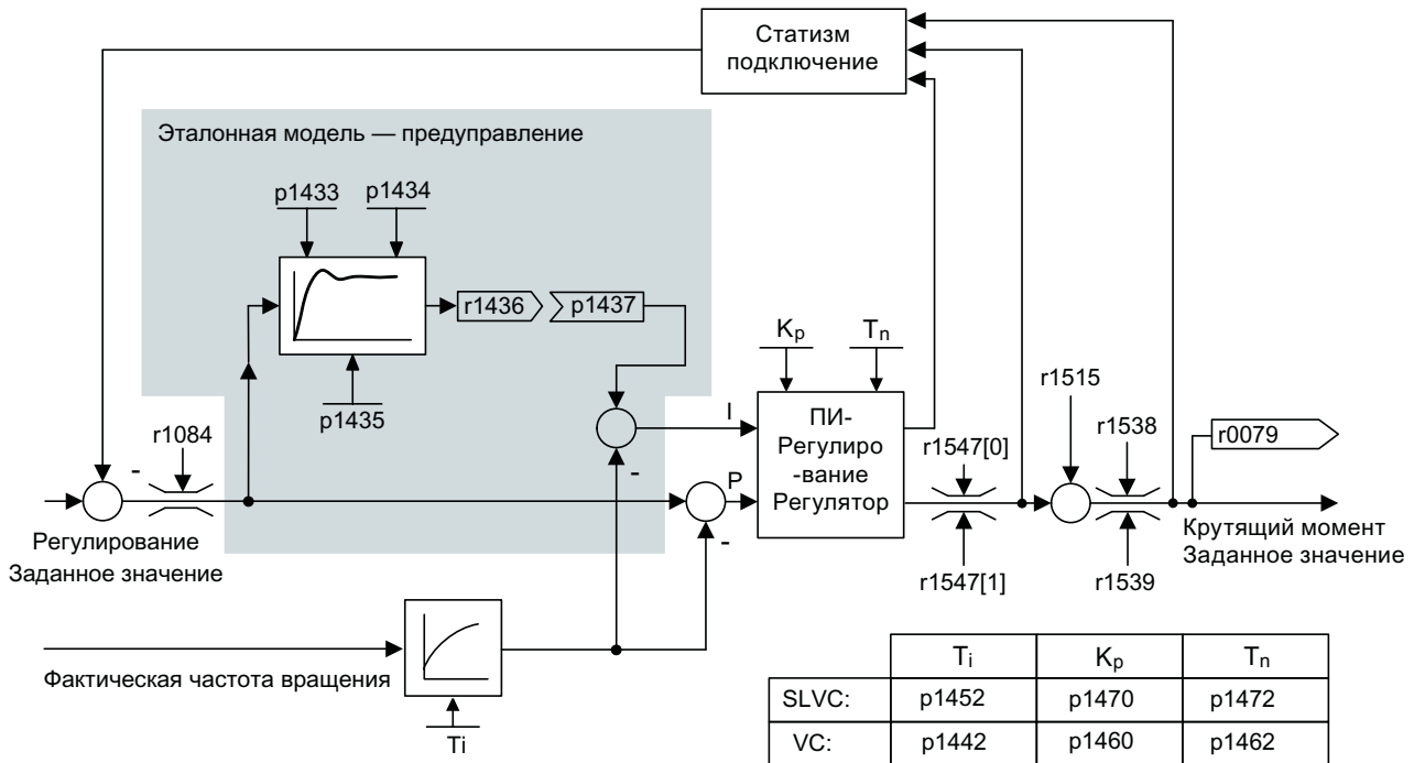
Рисунок 5-10 Эталонная модель
