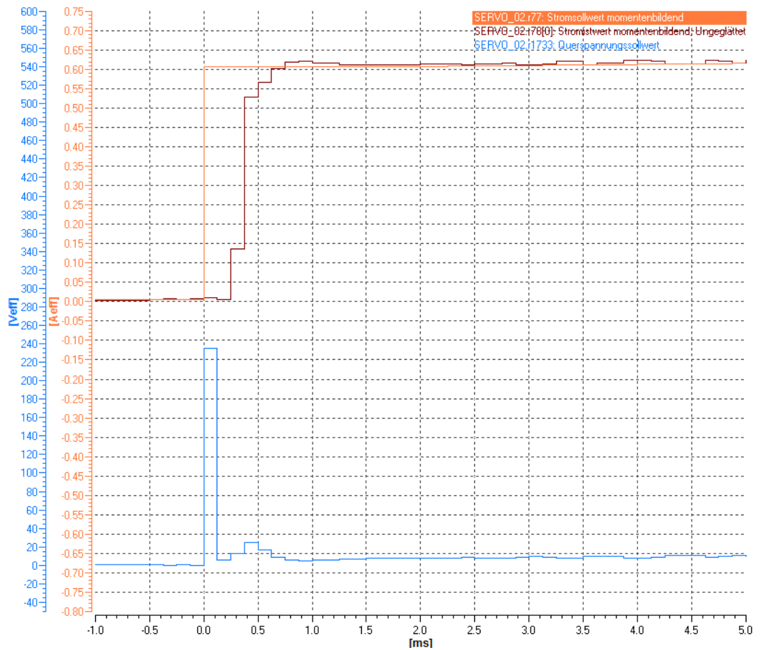
Рисунок 4-37 Предусиление регулирования напряжения p1703 слишком мало
