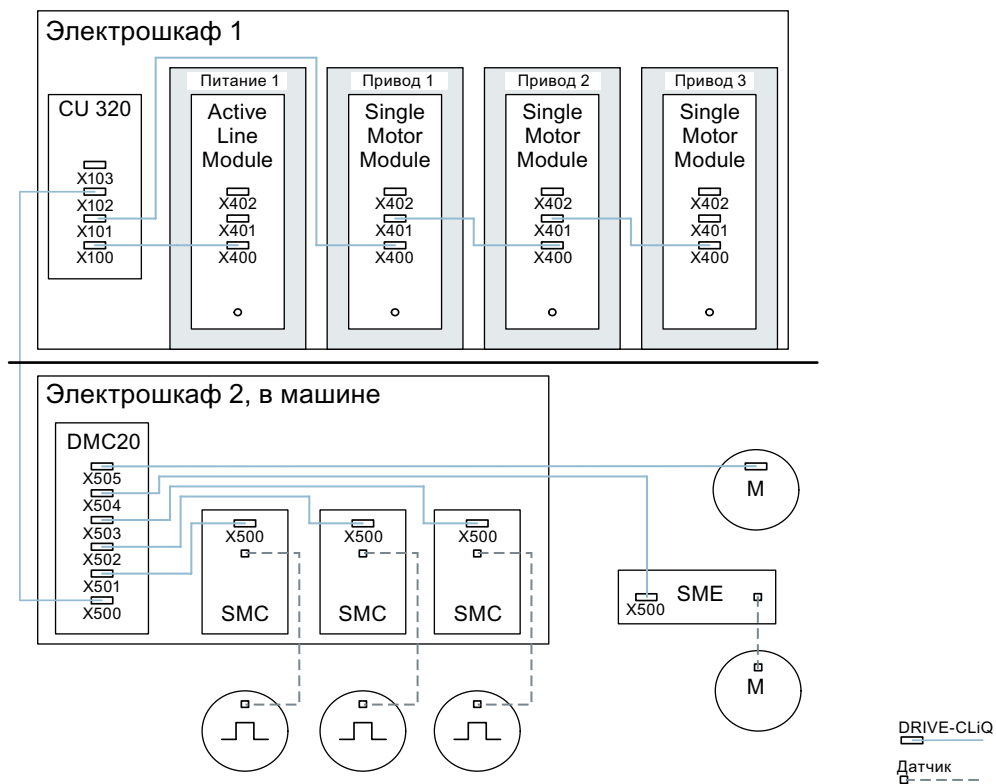
Рисунок 11-8 Пример децентрализованной конструкции с DMC20
