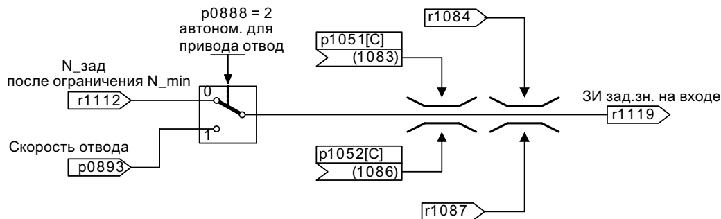
Рисунок 8-31 Интерфейс канала заданного значения на задатчике интенсивности
