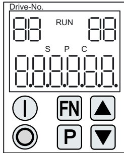
Рисунок А-9 Обзор индикаторов и кнопок
