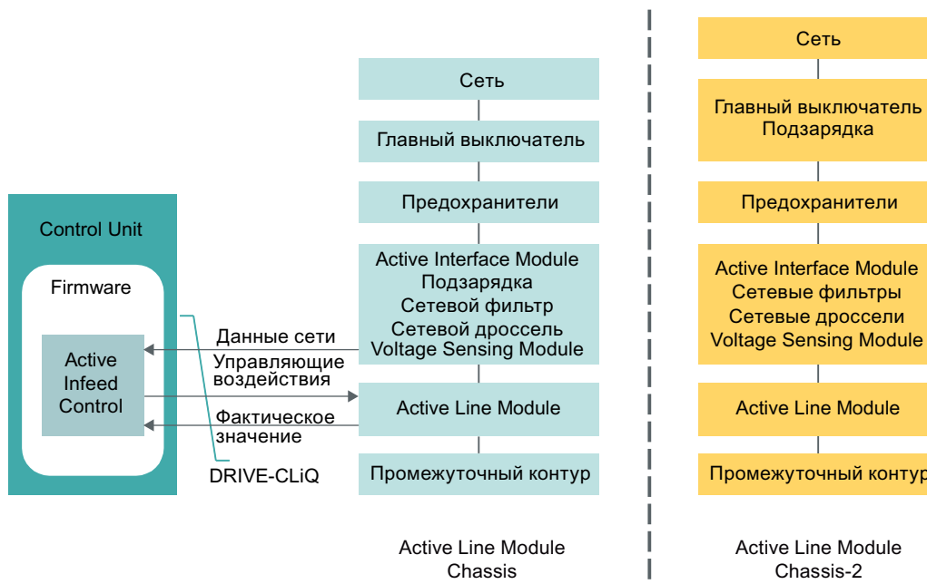
Рисунок 2-2 Схематическая структура управления Active Infeed Chassis и Chassis-2
