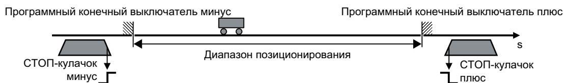
Рисунок 8-15 Программные и аппаратные конечные выключатели в качестве ограничений
