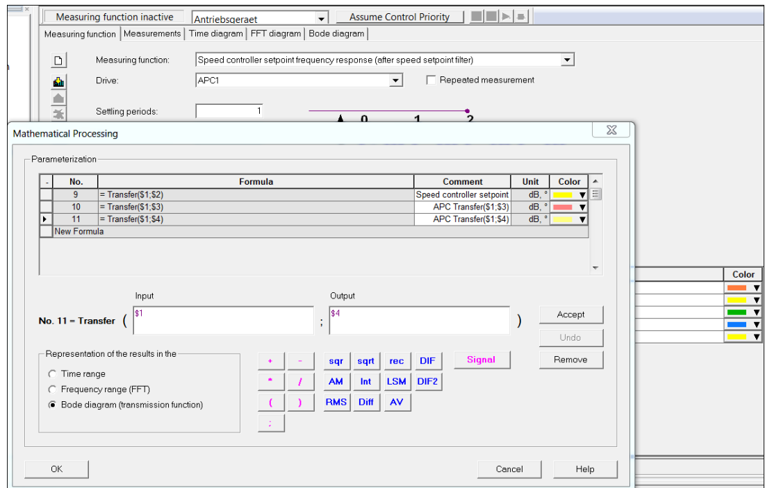
Рисунок 8-52 Передаточные функции
