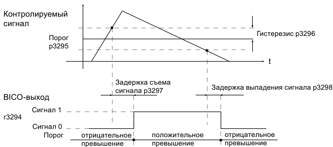
Рисунок 4-31 Переменная сигнальная функция
