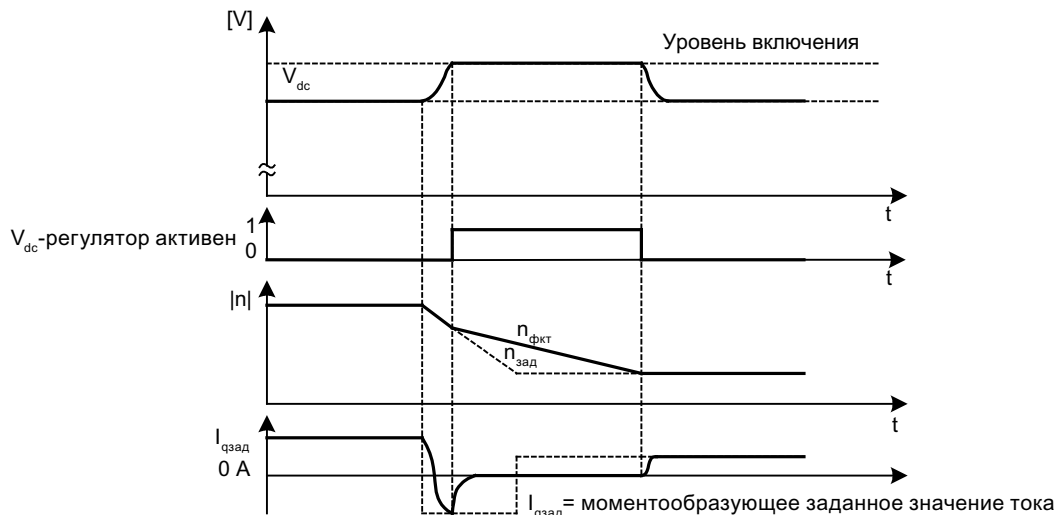
Рисунок 5-16 Включение/выключение V_{dc\_max} -регулирования
