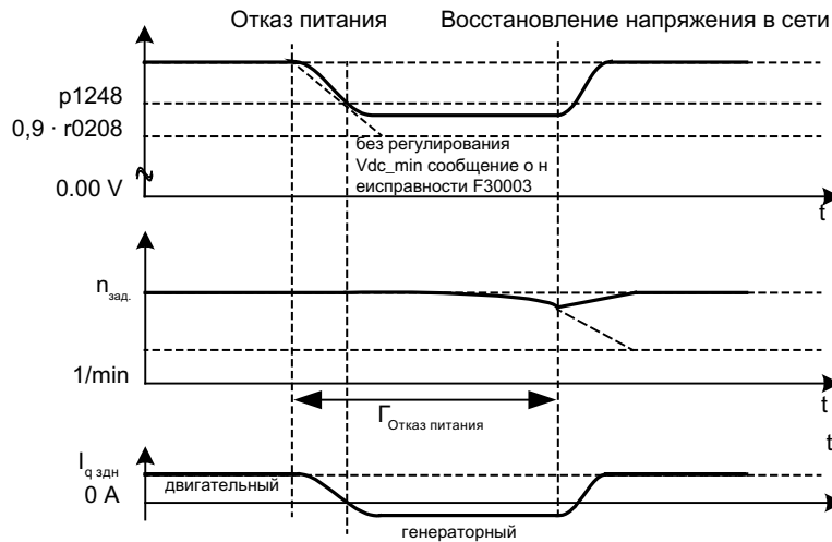
Рисунок 4-27 Включение/выключение V_{dc\_min} -регулирования (кинетическая буферизация)
