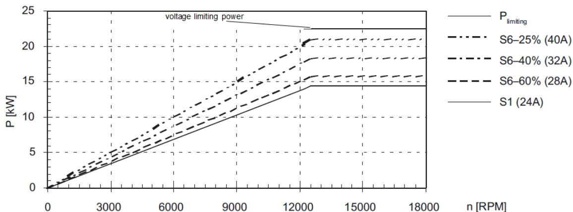
Рисунок 4-14 Синхронный двигатель: Характеристика мощность-вращающий момент
