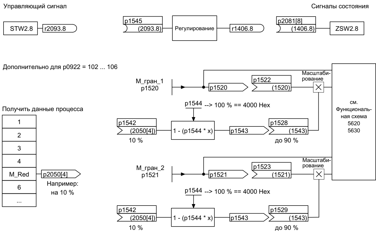
Рисунок 4-29 Сигналы при «Наезде на жесткий упор»
