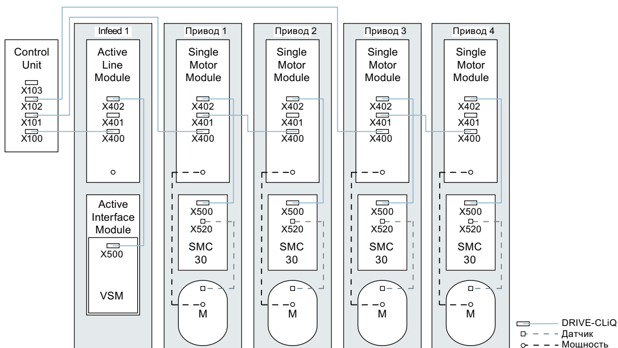
Рисунок А-2 Приводная группа формата «шасси» с разными частотами импульсов
