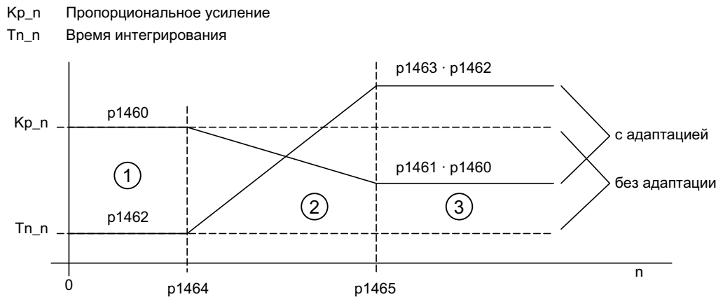
Рисунок 4-5 Адаптация регулятора частоты вращения- K_{p\_n}/T_{n\_n}
