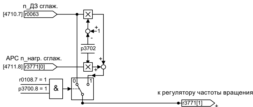
Рисунок 8-39 APC с функцией смешивания датчиков
