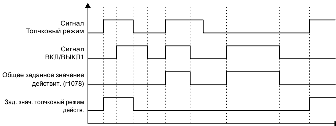
Рисунок 3-3 Блок-схема Толчковая подача и ВКЛ1
