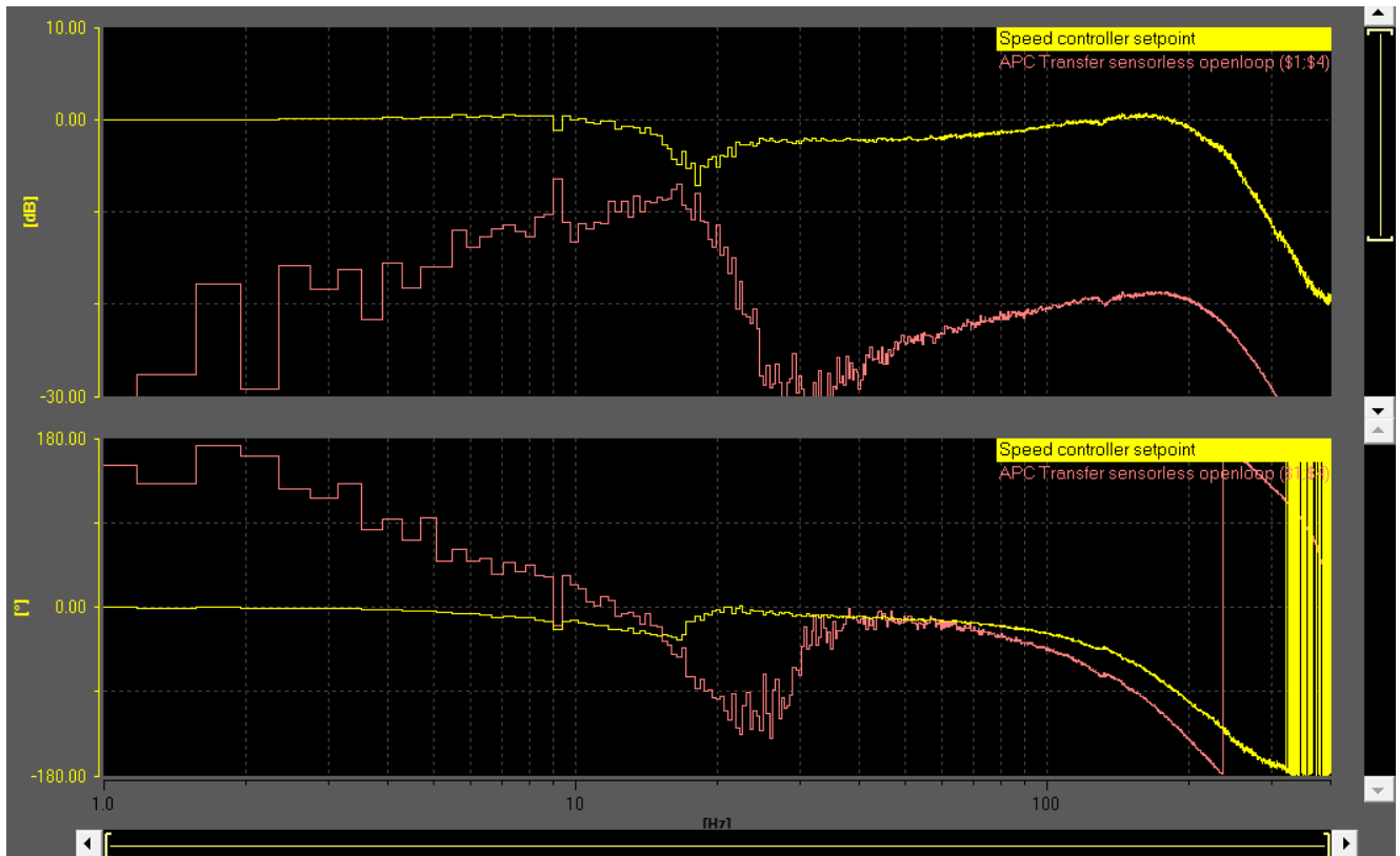
Рисунок 8-35 APC без датчика на стороне нагрузки ( p3700 = 4 ) — разомкнутый контур
