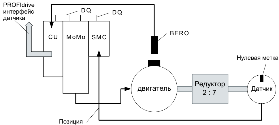
Рисунок 8-20 Измерительный редуктор между двигателем и датчиком
