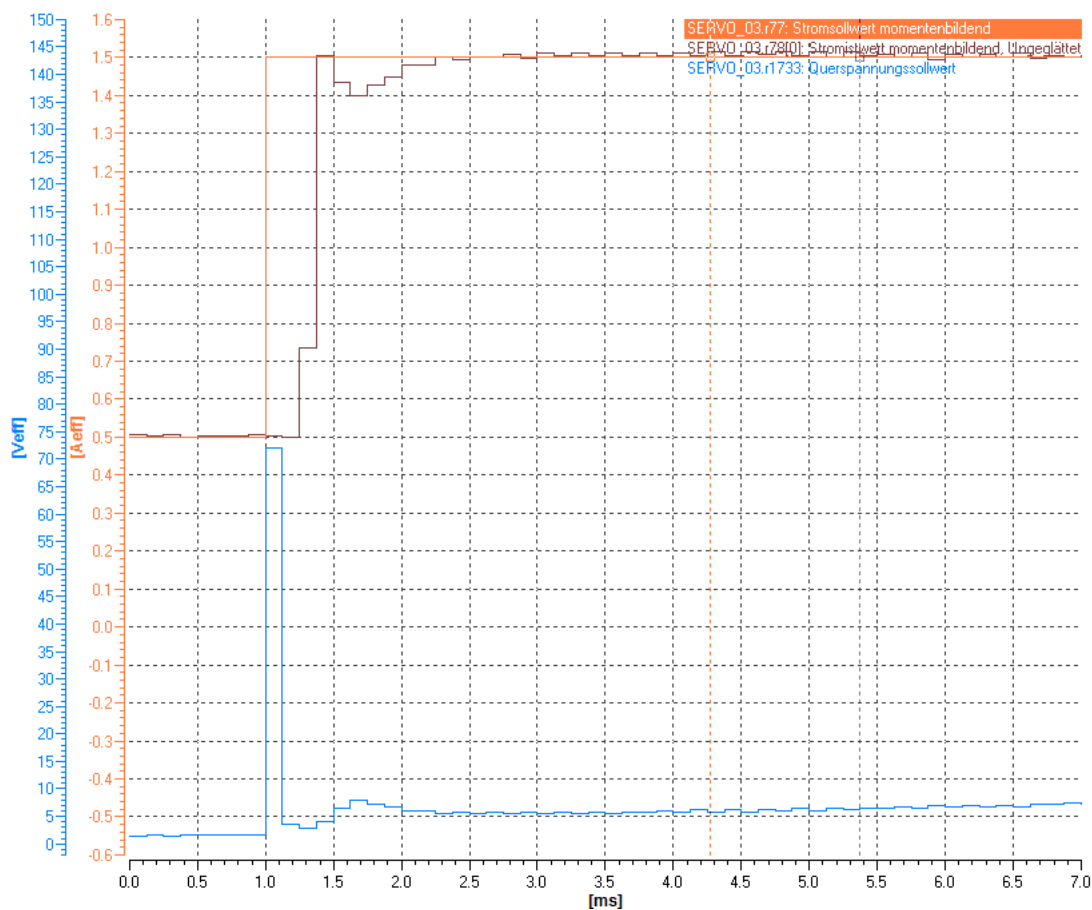
Рисунок 4-40 Пример: Предусиление регулирования напряжения перед оптимизацией (с выходом за пределы)
