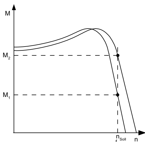
Рисунок 6-5 Компенсация скольжения
