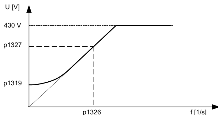
Рисунок 4-16 Характеристика U/f
