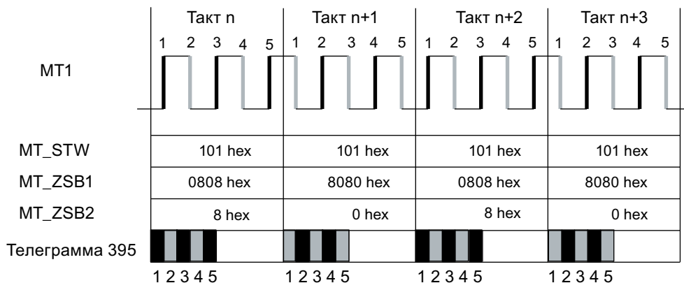
Рисунок 4-33 поиск передних и задних фронтов для щупа 1
