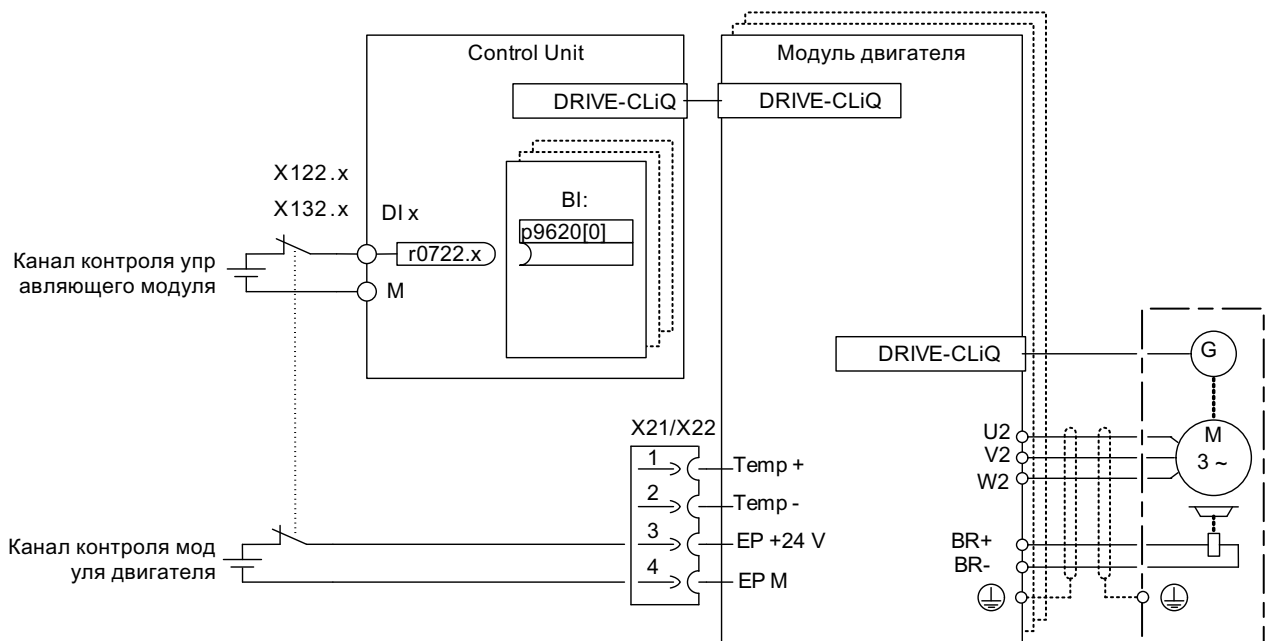
Рисунок 10-2 Пример: Клеммы для «Safe Torque Off», пример модулей двигателей книжного формата и CU320-2
