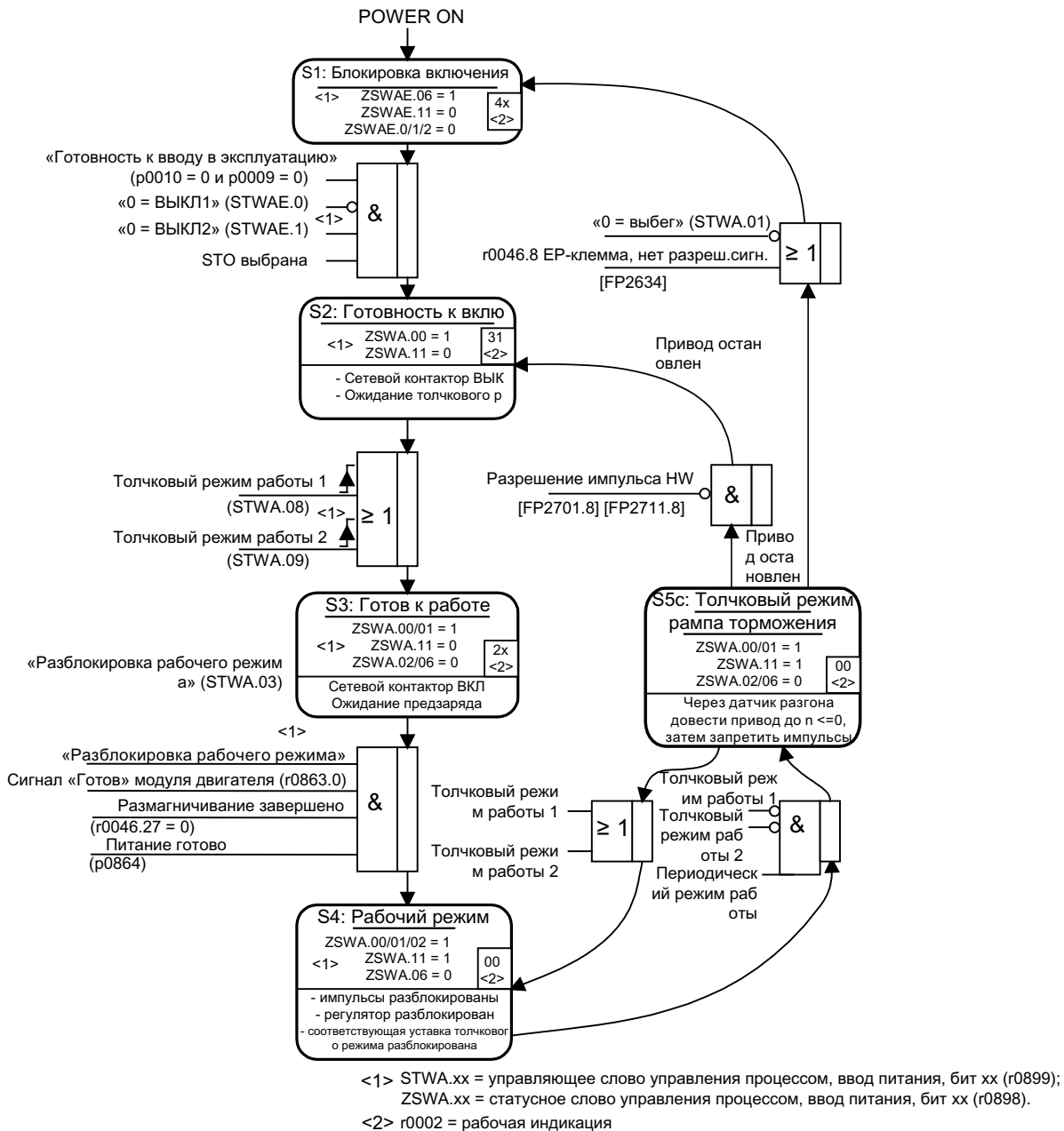
Рисунок 3-5 Процесс толковой подачи
