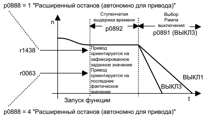
Рисунок 8-29 Рампа ВЫКЛ со ступенчатой выдержкой времени
