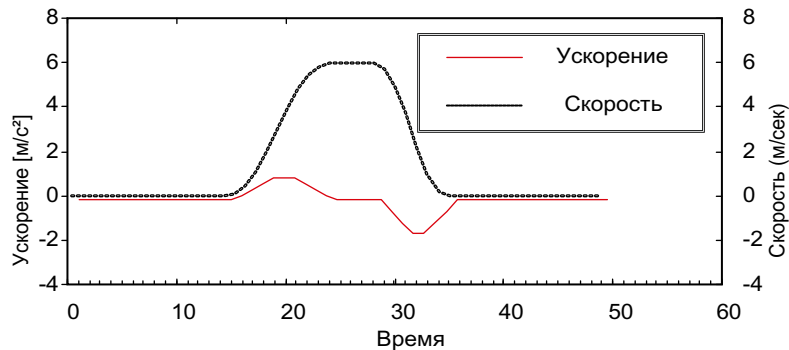
Рисунок 8-17 Активированное ограничение рывка
