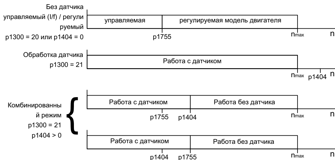
Рисунок 4-18 Переключение диапазона
