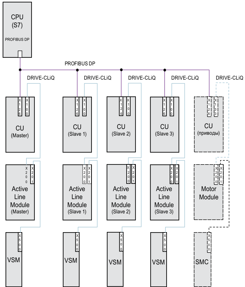
Рисунок 8-24 Топологическая структура и коммуникационная сеть через PROFIBUS для Master/ Slave-Betrieb для дублирующих блоков питания (4 структуры питания)
