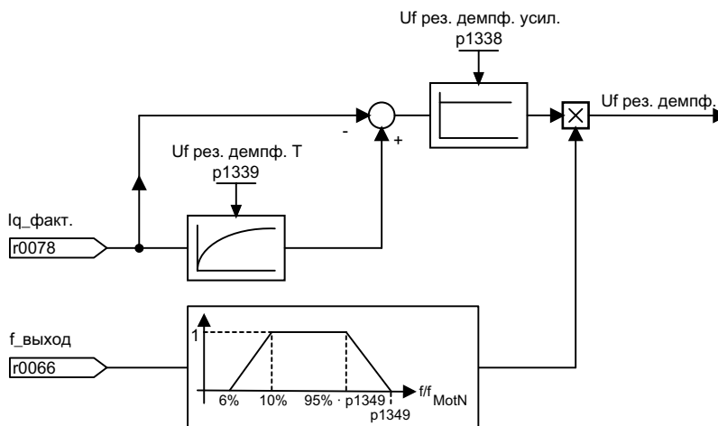
Рисунок 6-6 Поглощение резонанса
