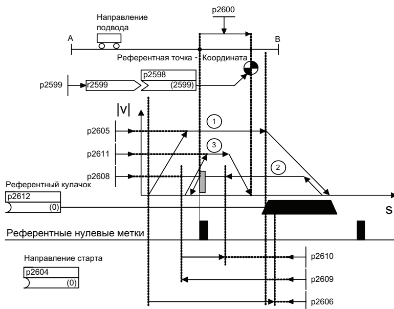
Рисунок 8-18 Пример реферирования с референтными кулачками
