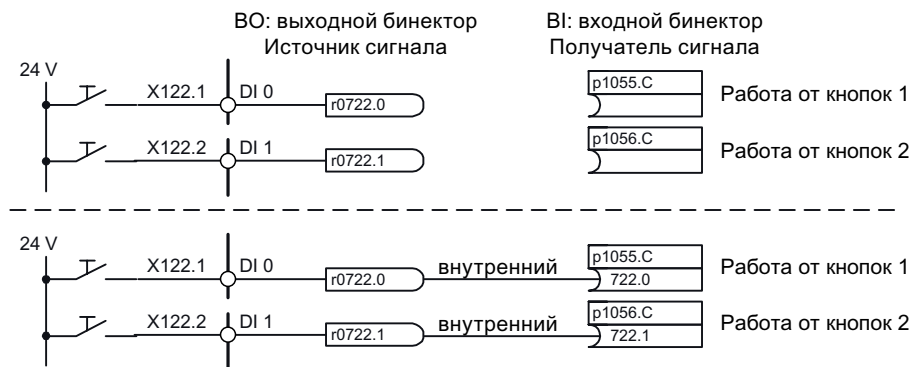
Рисунок 13-10 Соединение цифровых сигналов (пример)
