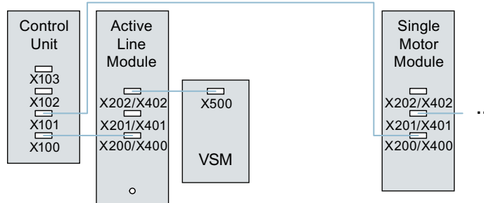
Рисунок 13-23 Пример топологии с VSM с компонентами книжного формата и формата «шасси»
