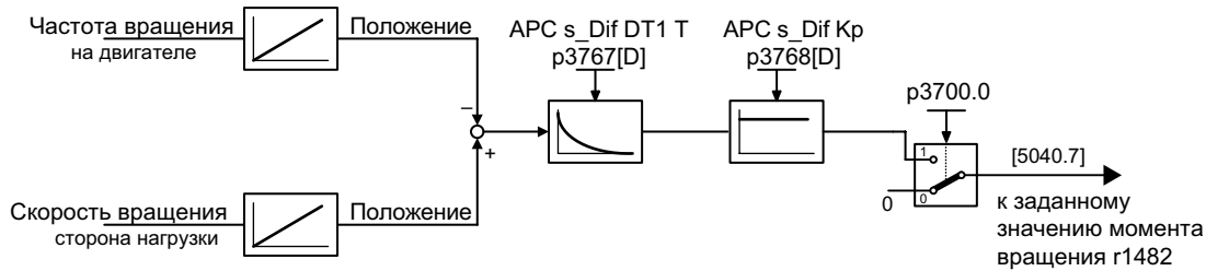
Рисунок 8-40 APC с обратной связью по разности положений
