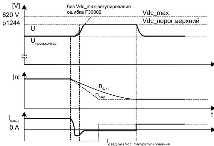
Рисунок 4-28 Включение/выключение V_{dc\_max} -регулирования
