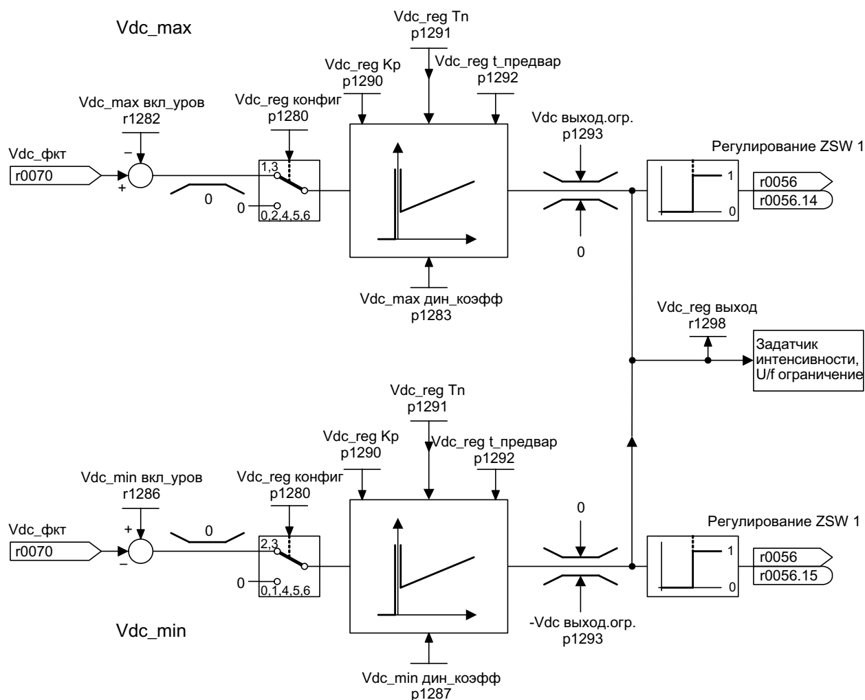
Рисунок 6-7 V dc -регулирование U/f
