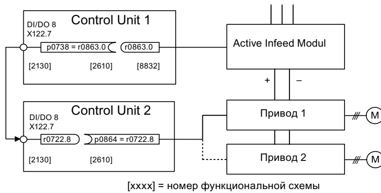
Рисунок 11-4 Иллюстративное соединение с несколькими управляющими модулями
