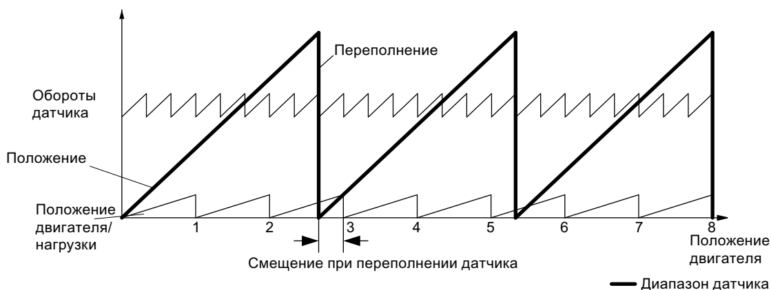
Рисунок 7-15 Привод с нечетным редуктором без отслеживания положения
