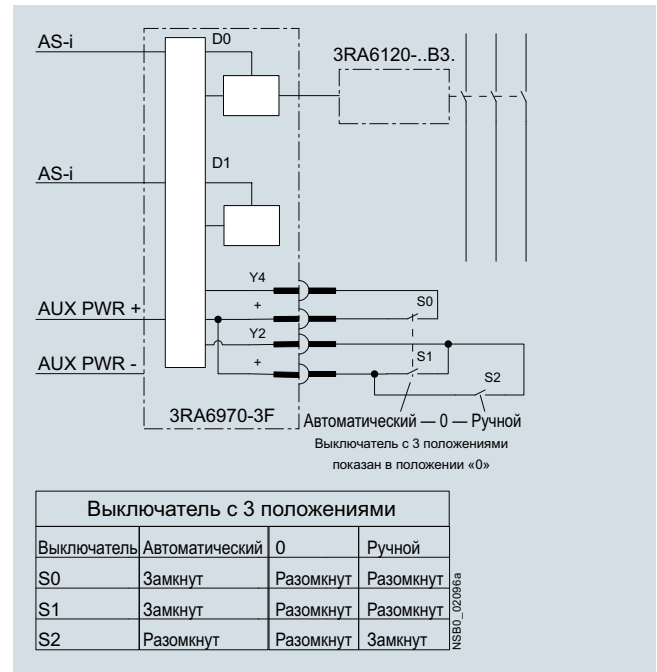
Пример принципиальной схемы для местного управления пускателем прямого пуска 3RA6120 при помощи навесного модуля AS-i
