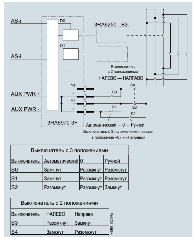
Пример принципиальной схемы для местного управления реверсивным пускателем 3RA6250 при помощи навесного модуля AS-i
