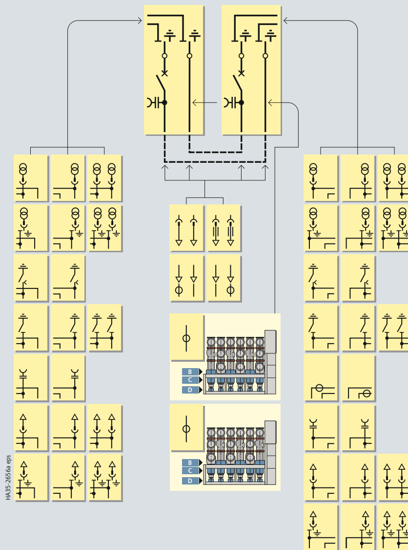
Секционный выключатель (система сборных шин 1 и 2)
