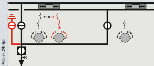
Фидер системы сборных шин 2 ВКЛ
