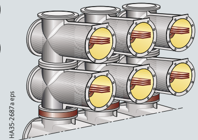
Исполнение сборной шины 5000 А (танDEMная сборная шина) Пример 8DA10
