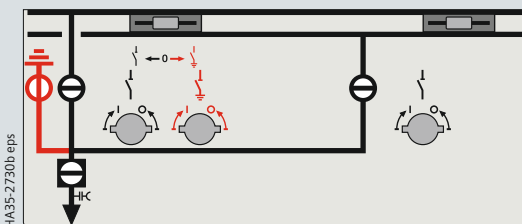
Фидер ЗАЗЕМЛЕНИЕ ПОДГОТОВЛЕНО
