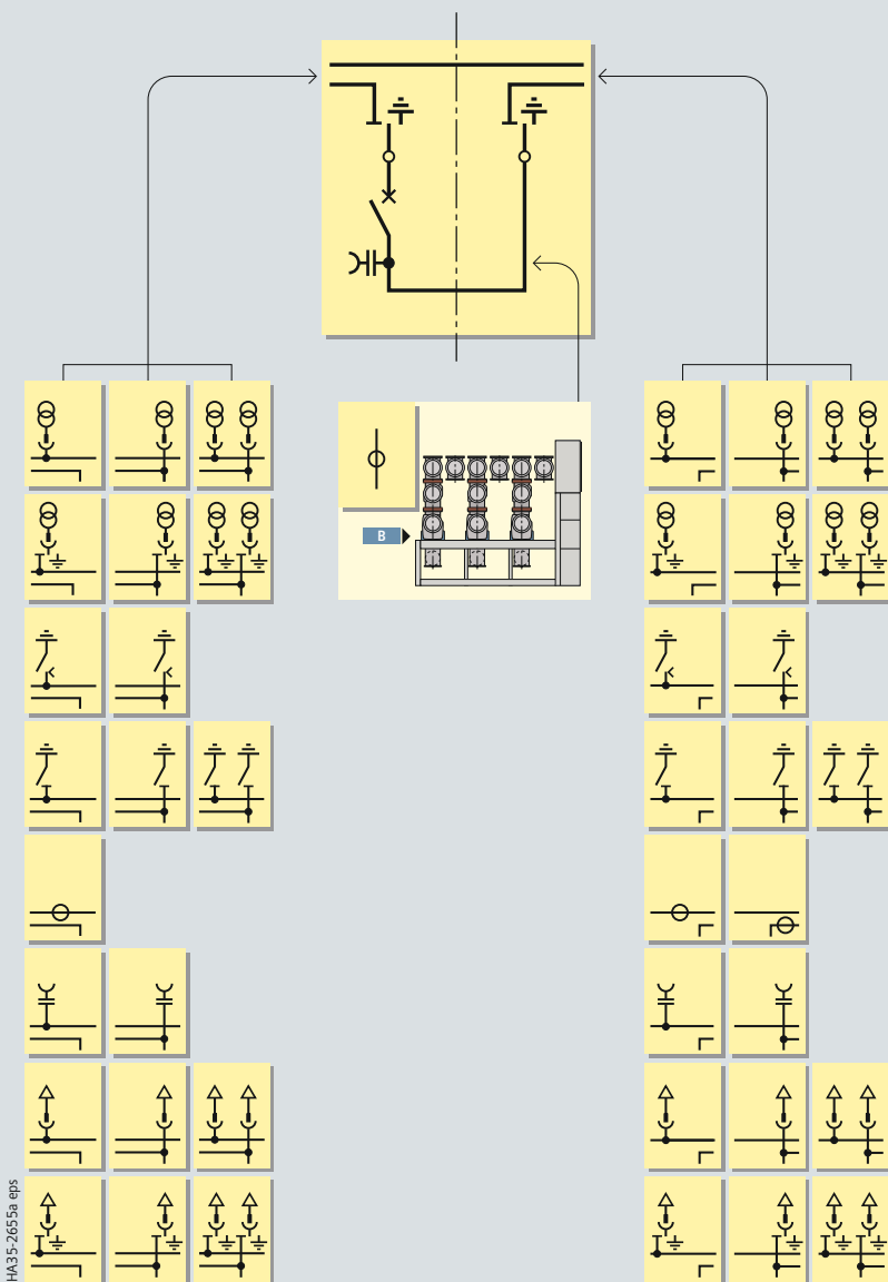
Секционный выключатель (система сборных шин 2)
