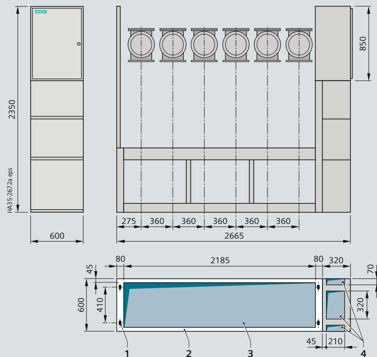
Пустая ячейка
