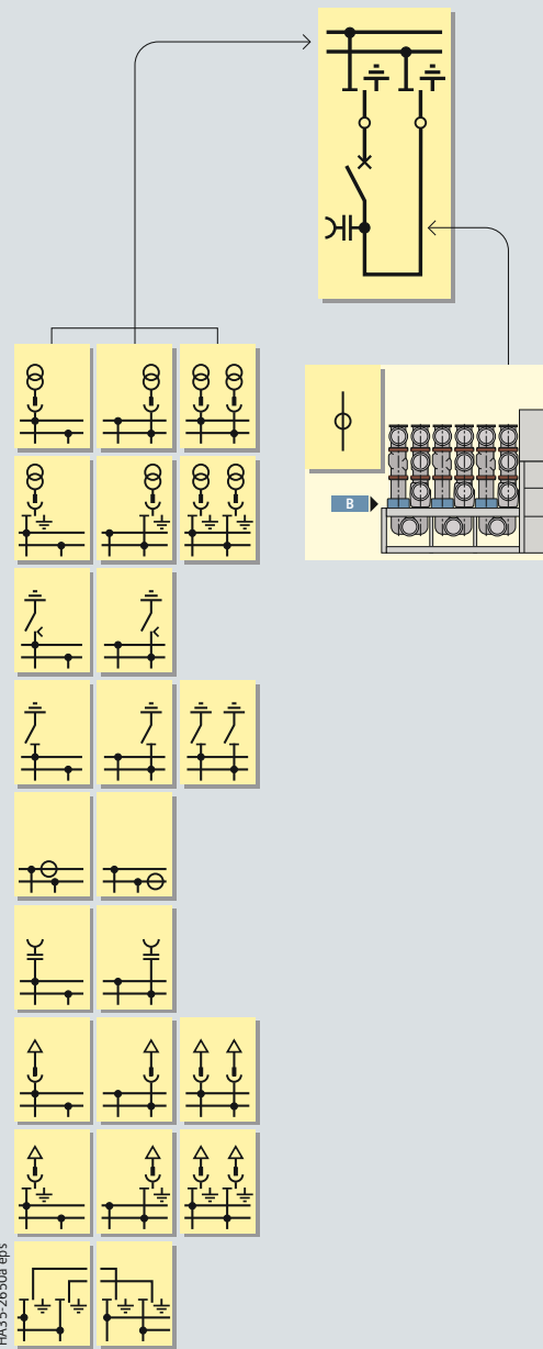
Ячейка секционного выключателя
