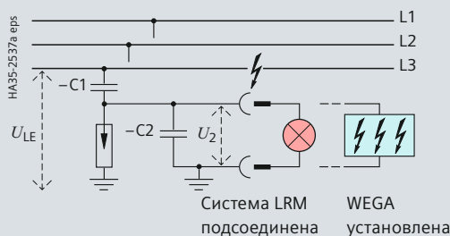
Интегрированная система проверки наличия напряжения WEGA 2.2
