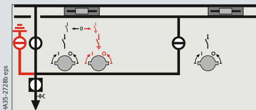
Фидер системы сборных шин 1 ВКЛ
