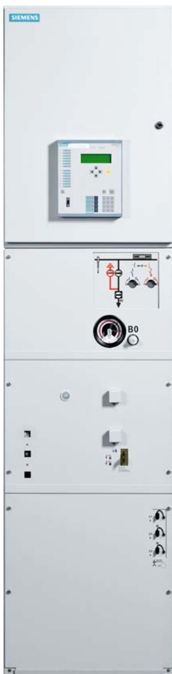
КРУЭ с силовым выключателем 8DA10
