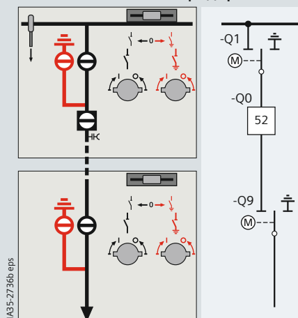
Фидер ОТКЛ
