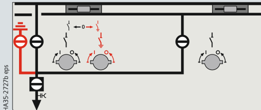
Фидер ОТКЛ
