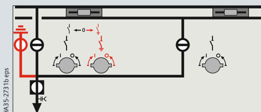
Фидер ЗАЗЕМЛЕН
