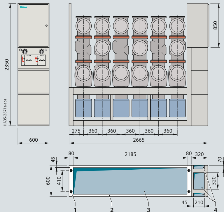
Измерительная ячейка
