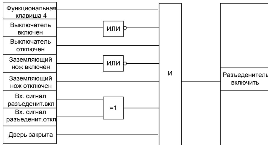
Рисунок 5-39 Блокировка разъединителя. Пример определенной пользователем блокировки.
