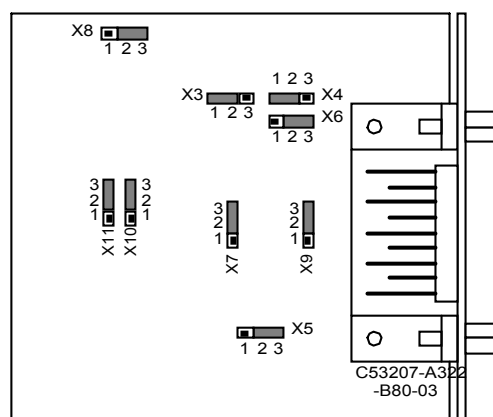
Рисунок 8-7 Расположение переключателей для установки согласующего сопротивления интерфейса версии C53207-A322-B80.
