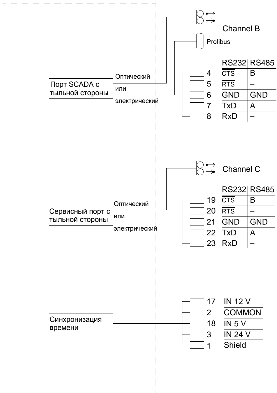
Рисунок А-7 Общая схема 7SJ60/1/2*-*B (Установка на панели)
