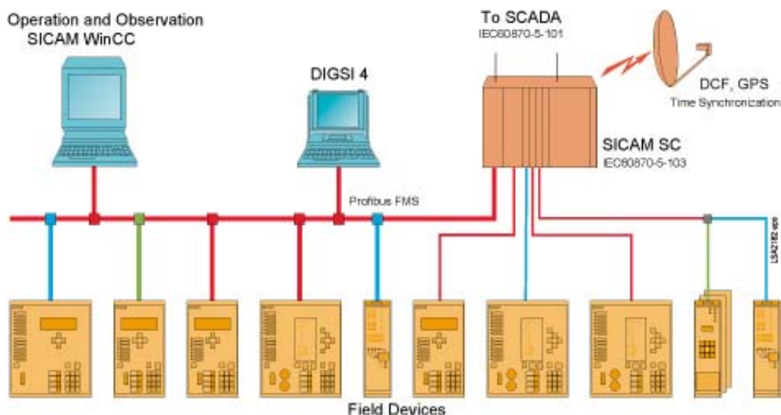
Рисунок 4-1 Пример интеграции полевых устройств в SICAM систему управления станцией
