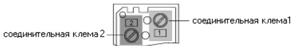
Рисунок 2-4 Соотношение (взаимосвязь) между винтовыми клеммами и номерами подключения (пример)
