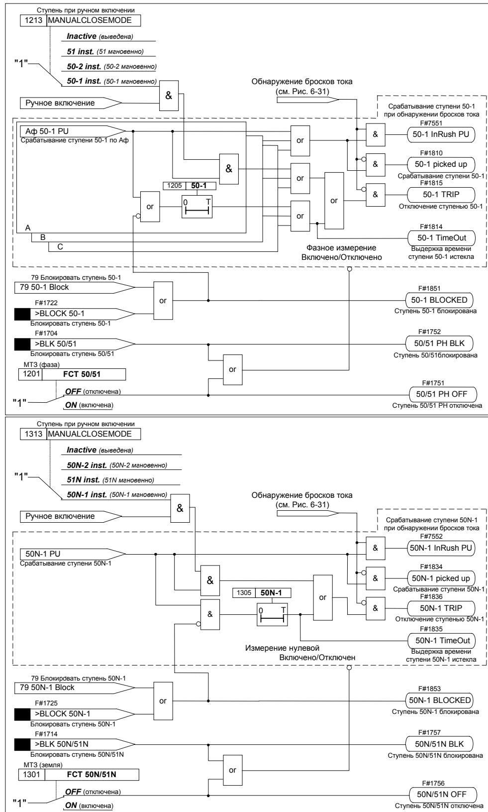
Рисунок 6-12 Схема логики защитных ступеней 50-1 и 50N-1
