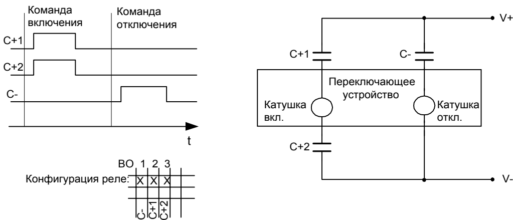
Рисунок 5-9 Двойная команда с двойными и одиночными контактами (3 реле)
