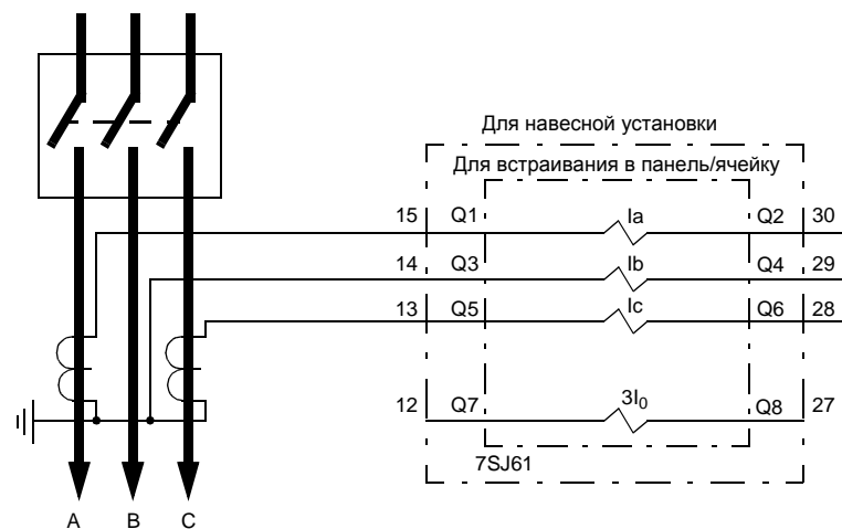
Рисунок А-9 Токовые цепи с двумя трансформаторами тока для незаземленных или компенсированных сетей
