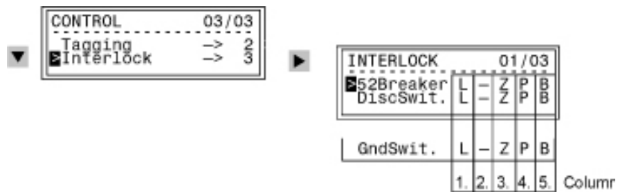
Рисунок 7-52 Пример Условий Блокировки Коммутационного Оборудования, Передняя Панель
