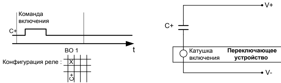
Рисунок 5-4 Одиночная команда с одним выходом
