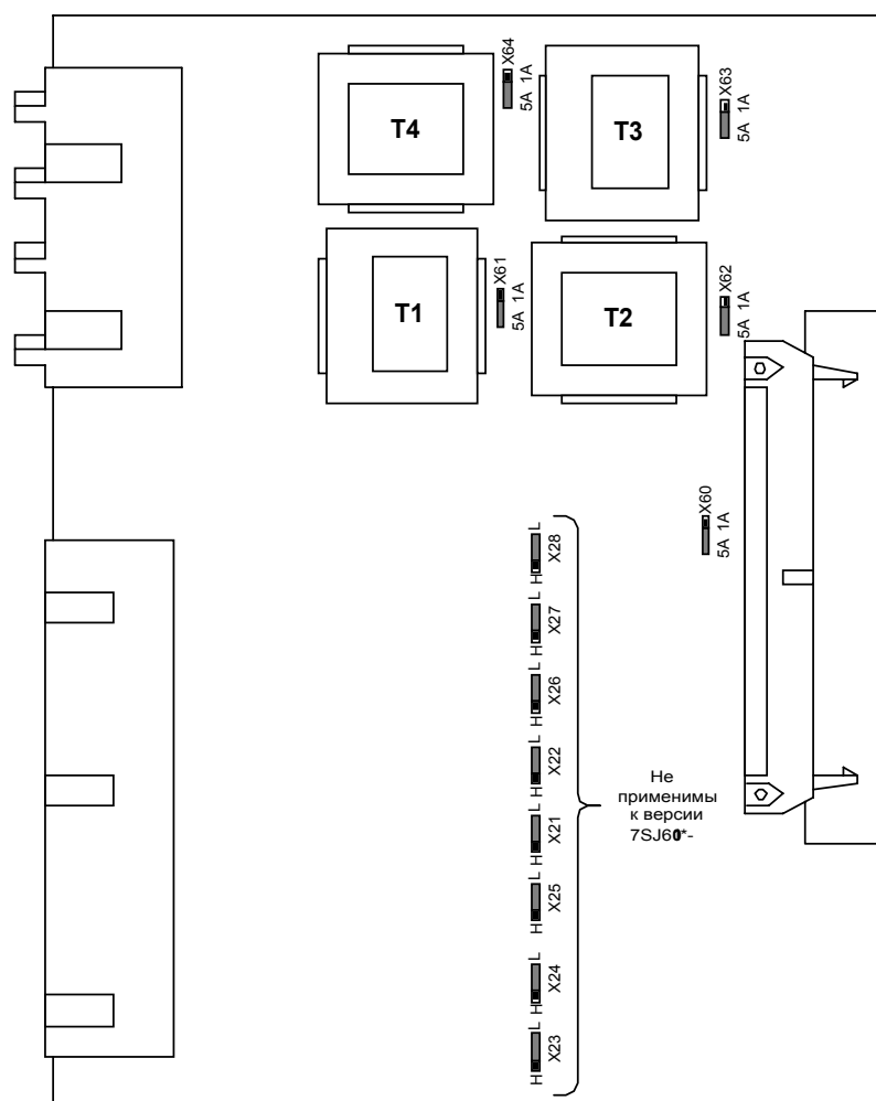
Рисунок 8-6 Переключатели на плате ввода/вывода для трансформаторов тока и бинарных входов от BI4 до BI11 (упрощено).
