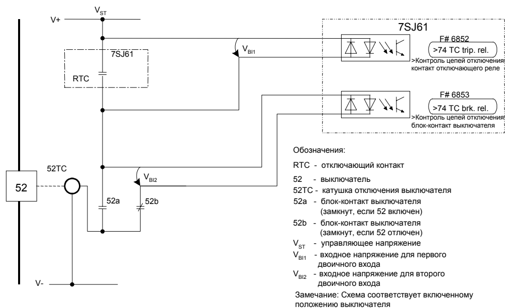
Рисунок 6-43 Контроль цепей отключения с помощью двух двоичных входов
