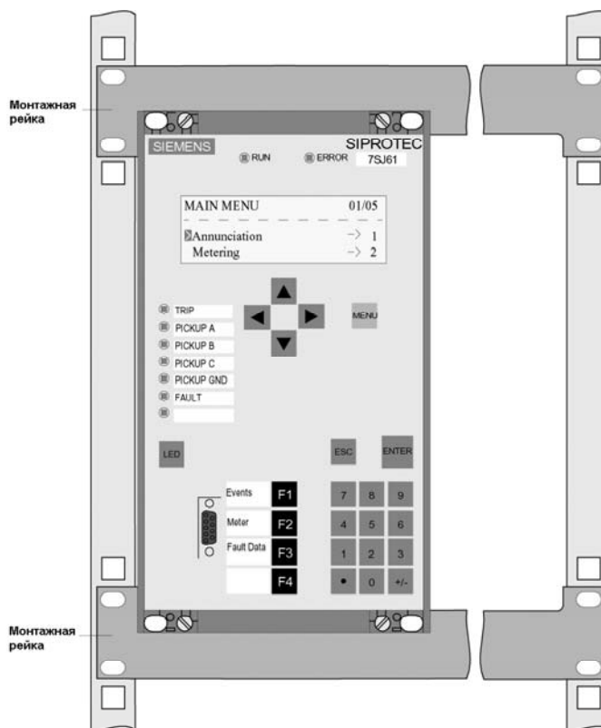
Рисунок 8-2 Установка на стойку 7SJ61.
