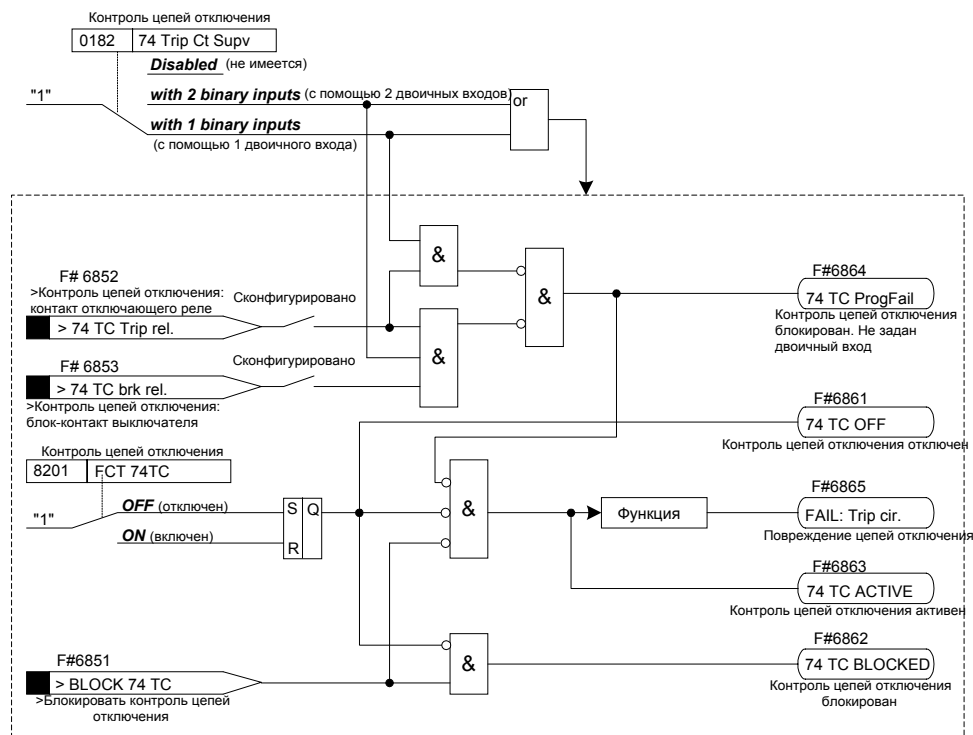
Рисунок 6-47 Схема логики формирования сообщений функции контроля цепей отключения
