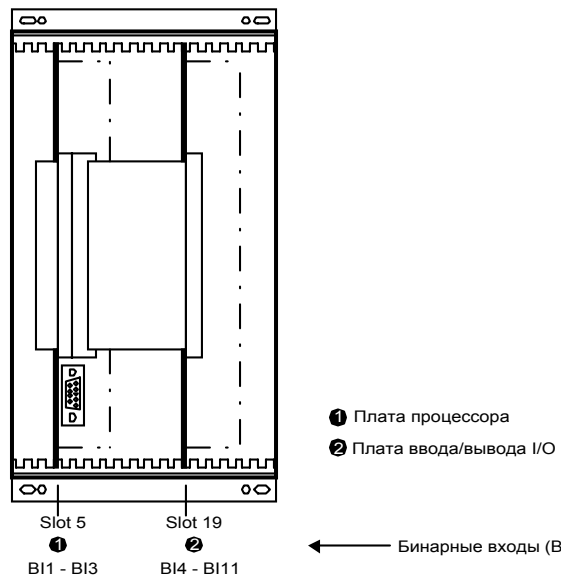
Рисунок 8-4 Вид спереди. Передняя панель снята. (Упрощено и уменьшено).
