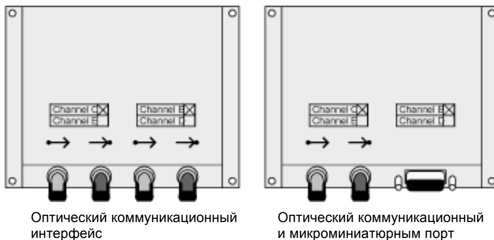
Рисунок 2-16 Панель корпуса с оптическими коммуникационными интерфейсами
