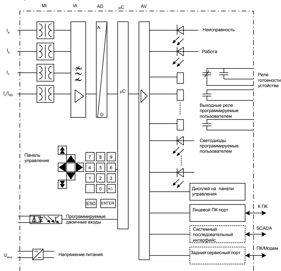
Рисунок 1-1 Структурная схема аппаратного обеспечения цифрового устройства 7SJ61 (Максимальная конфигурация)
