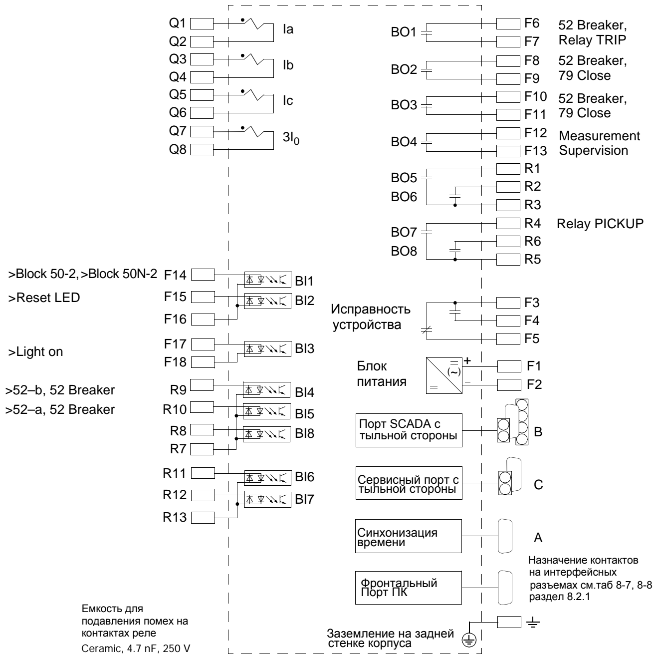
Рисунок А-2 Общая схема 7SJ611*-*D/E (Для встраивания в панель или установки в ячейку)
