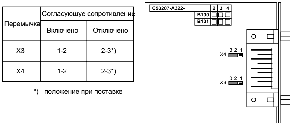
Рисунок 8-9 Расположение переключателей для установки согласующего сопротивления Profibus интерфейса.
