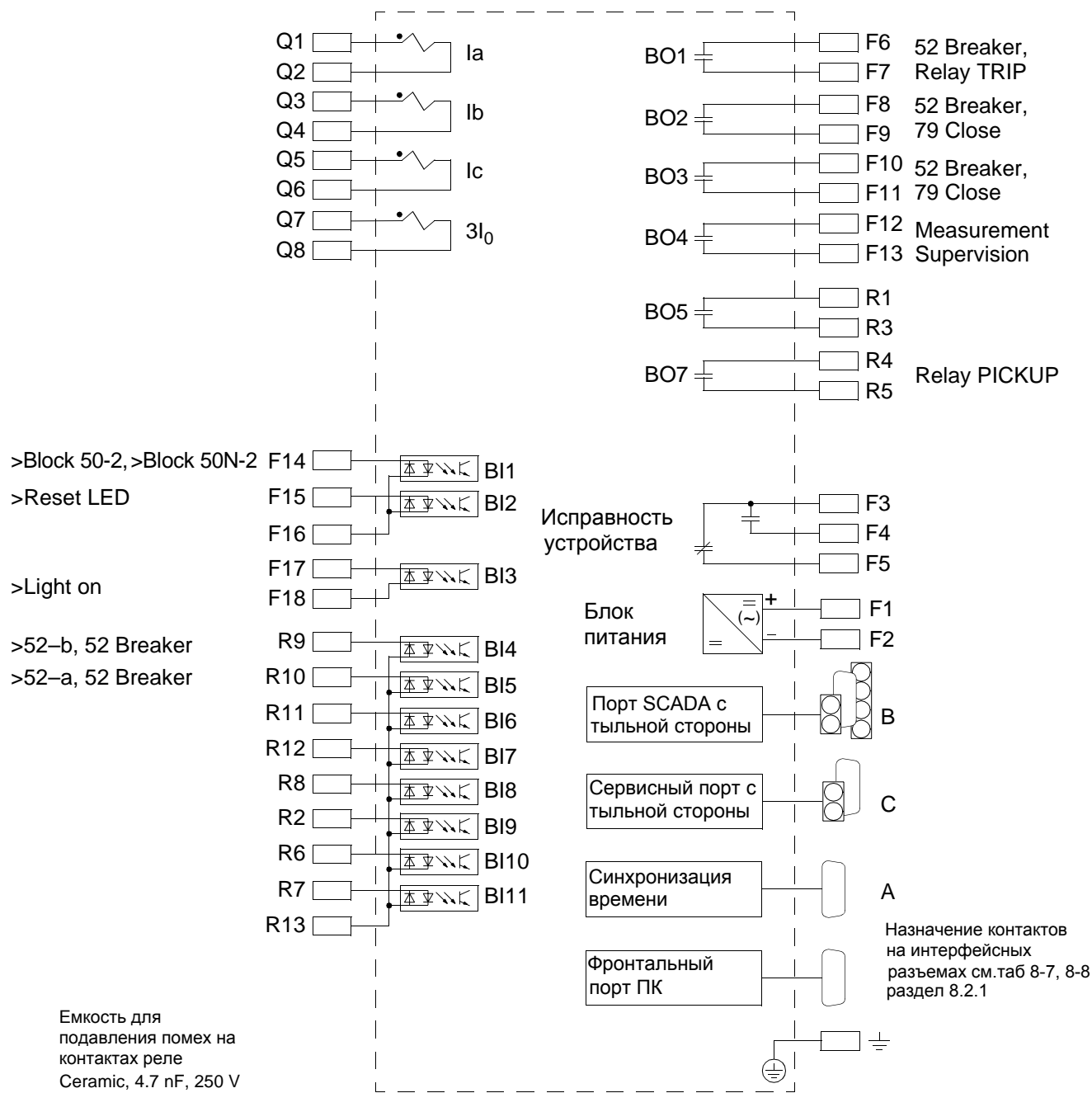
Рисунок А-3 Общая схема 7SJ612*-*D/E (Для встраивания в панель или установки в ячейку)
