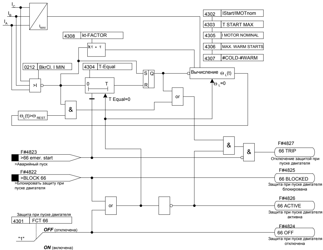
Рисунок 6-32 Схема логики блокировки от многократного включения двигателей
