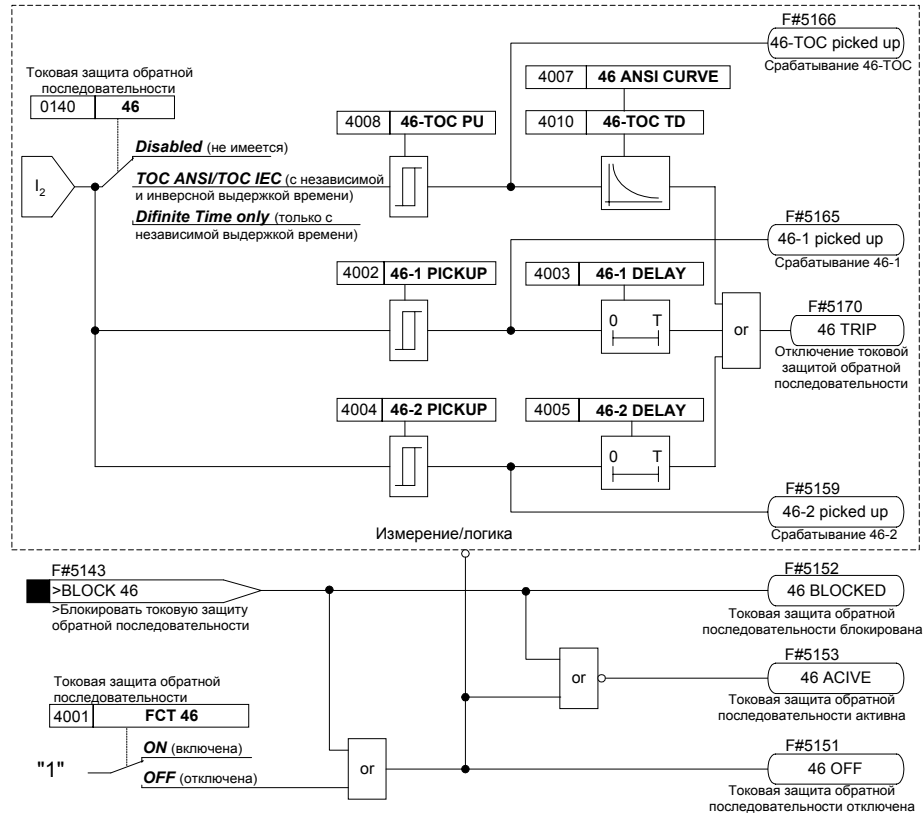
Рисунок 6-27 Схема логики токовой защиты обратной последовательности
