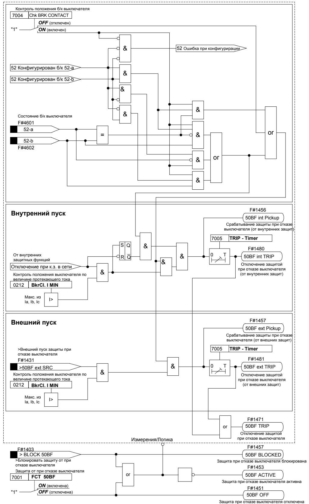
Рисунок 6-34 Схема логики защиты при отказе выключателя
