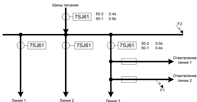
Рисунок 6-38 Пример применения чередования зон и защиты расположенных со стороны нагрузки предохранителей
