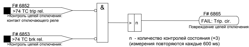
Рисунок 6-44 Схема логики контроля цепей отключения с помощью двух дискретных входов
