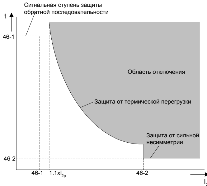
Рисунок 6-26 Инверсная временная характеристика для токовой защиты обратной последовательности
