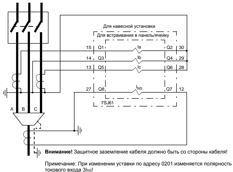
Рисунок А – 9. Токовые цепи с двумя трансформаторами тока и трансформатором тока с компенсированным магнитным сердечником в нейтрали, для высокочувствительного определения повреждения на землю – только для сетей с незаземленной или компенсированной нейтралью
