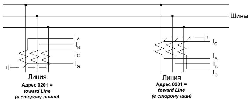
Рисунок 6-8 Варианты подключения трансформатора тока
