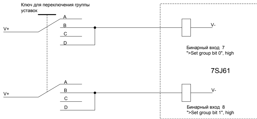
Рисунок 8-3 Схема переключения групп уставок через бинарные входы. Пример.
