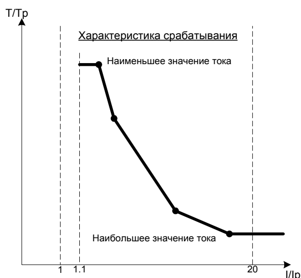
Рисунок 6-24 Применение определяемой пользователем кривой
