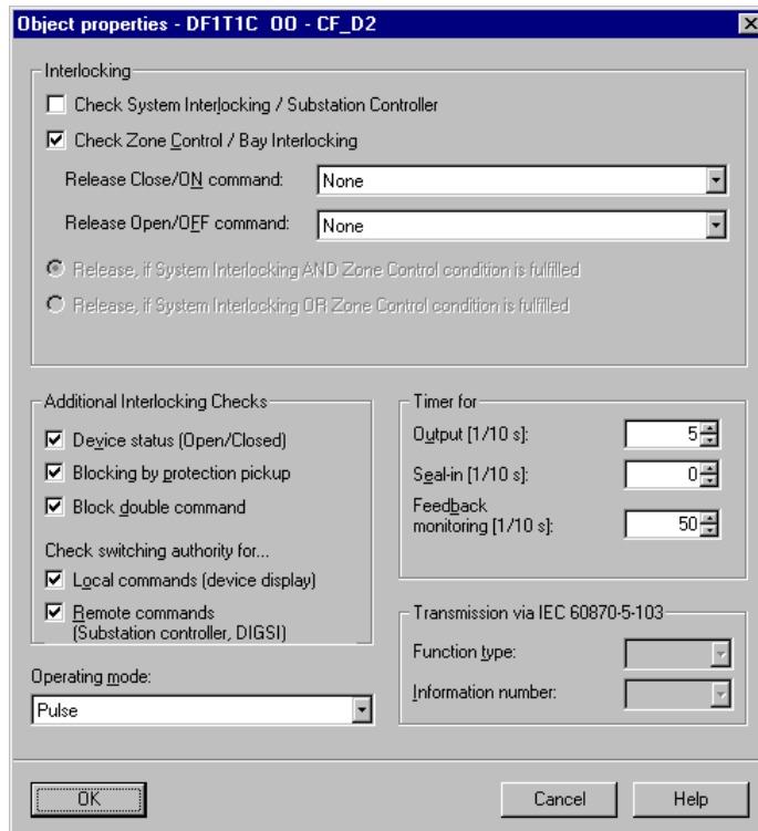
Рисунок 5-25 Окно диалога – Свойства объекта для команды с обратной связью (Пример: Двойная команда с одним отключающим выходом и двумя включающими выходами, CF_D12)
