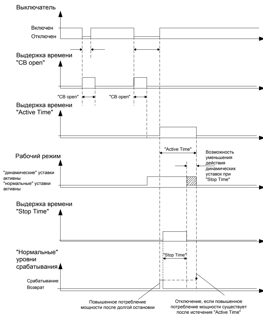
Рисунок 6-19 Временная диаграмма функции загрузления токовых защит при включении
