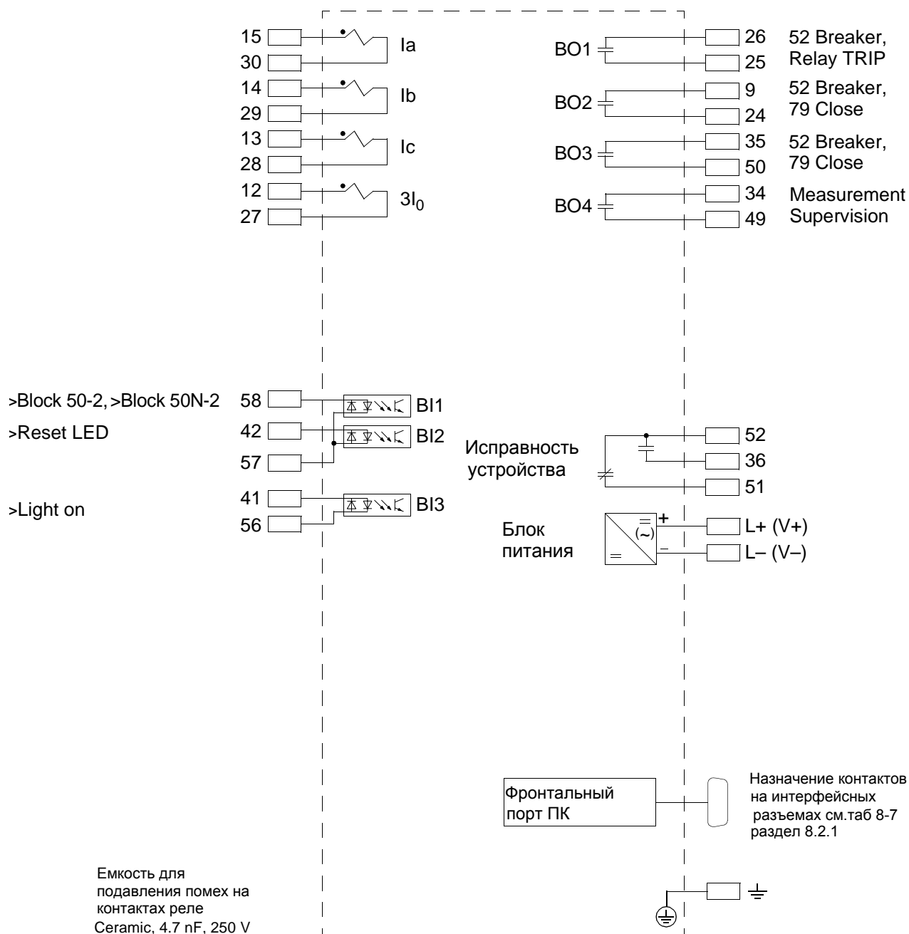
Рисунок А-4 Общая схема 7SJ610*-*B (Установка на панели)
