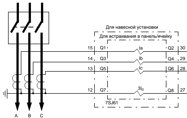
Рисунок А-8 Токовые цепи с тремя трансформаторами тока соединенных в звезду с заземленной нейтралью. Используется для всех типов сетей.
