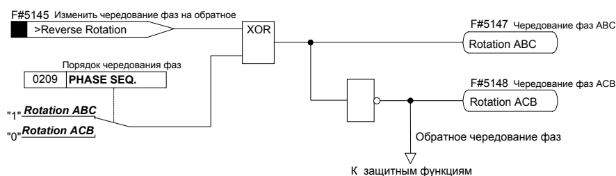
Рисунок 6-40 Схема логики переключения направления чередования фаз
