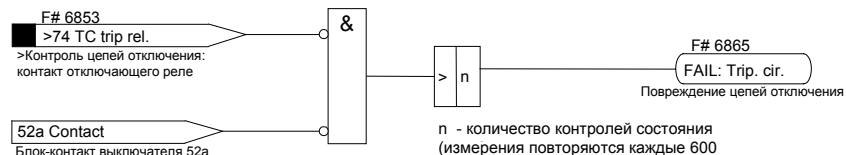
Рисунок 6-45 Схема логики контроля цепей отключения с помощью одного двоичного входа
