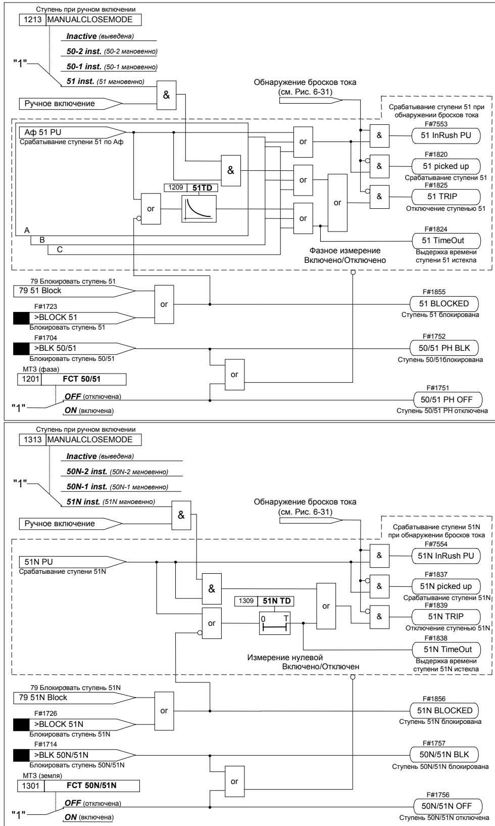
Рисунок 6-13 Схема логики защитных ступеней 51 и 51N
