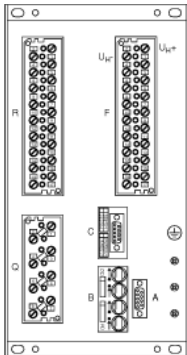
Рисунок 2-2 Задний вид устройства 7SJ61, с винтовыми клеммами (только для примера).
