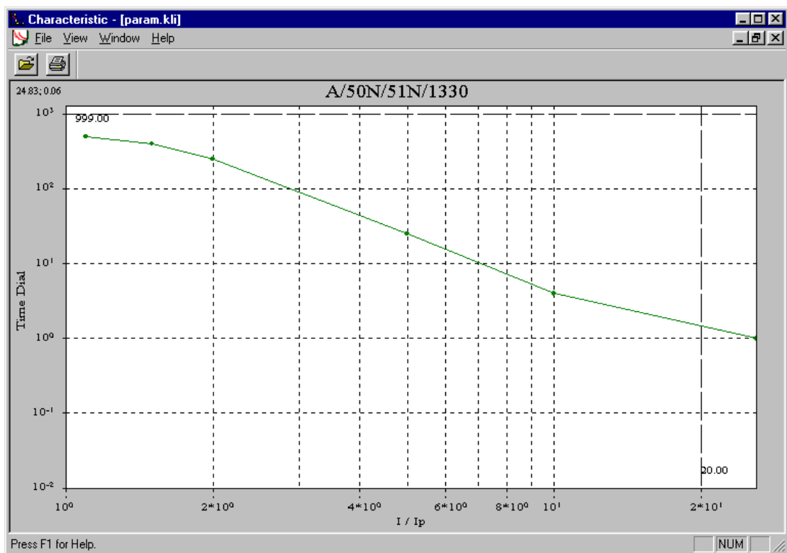
Рисунок 6-17 Графическое представление определяемой пользователем кривой в DIGSI®4
