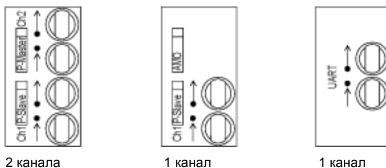
Рисунок 2-12 Оптические коммуникационные интерфейсы с защитными наконечниками
