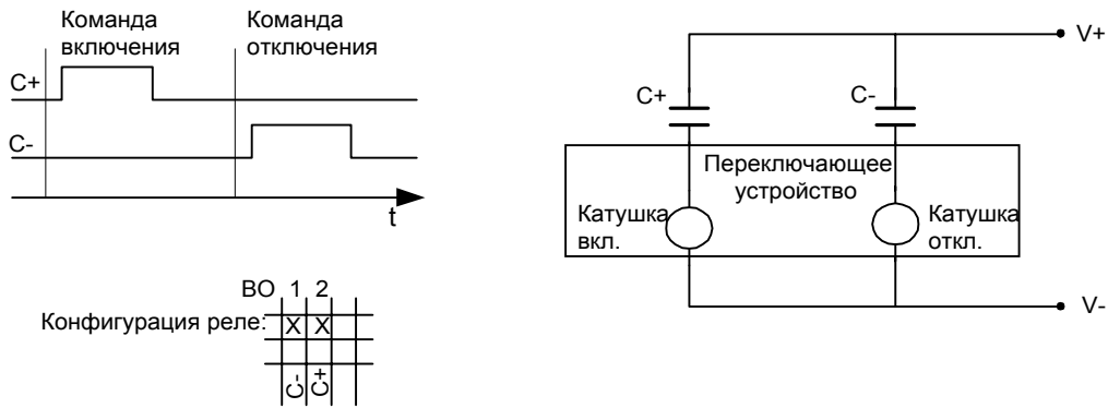
Рисунок 5-5 Двойная команда с одиночными контактами
