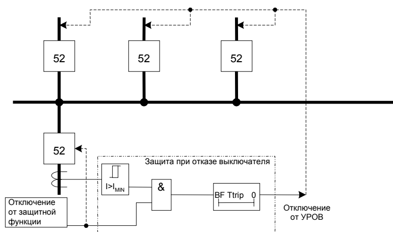
Рисунок 6-33 Принцип действия защиты при отказе выключателя
