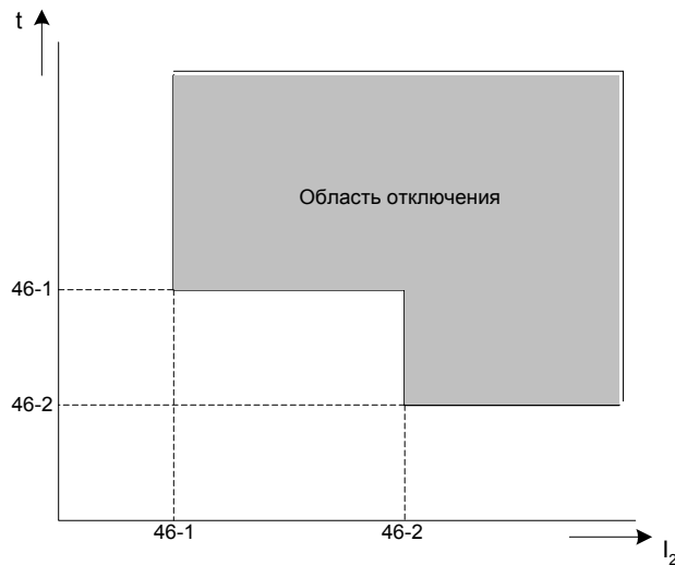
Рисунок 6-25 Независимая временная характеристика для токовой защиты обратной последовательности
