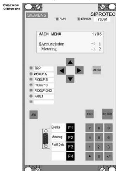
Рисунок 8-1 Установка на панель 7SJ61
