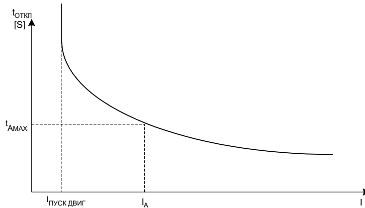
Рисунок 6-28 Инверсная временная характеристическая кривая отключения для пускового тока двигателя
