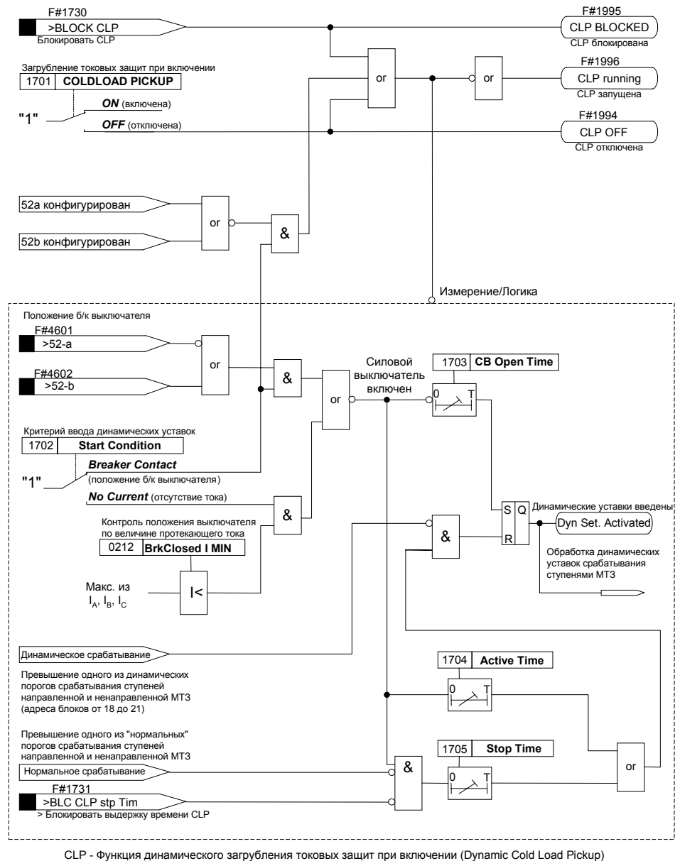
Рисунок 6-20 Схема логики функции загрубления токовых защит при включении
