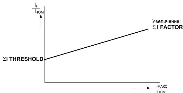
Рисунок 6-41 Контроль суммы токов
