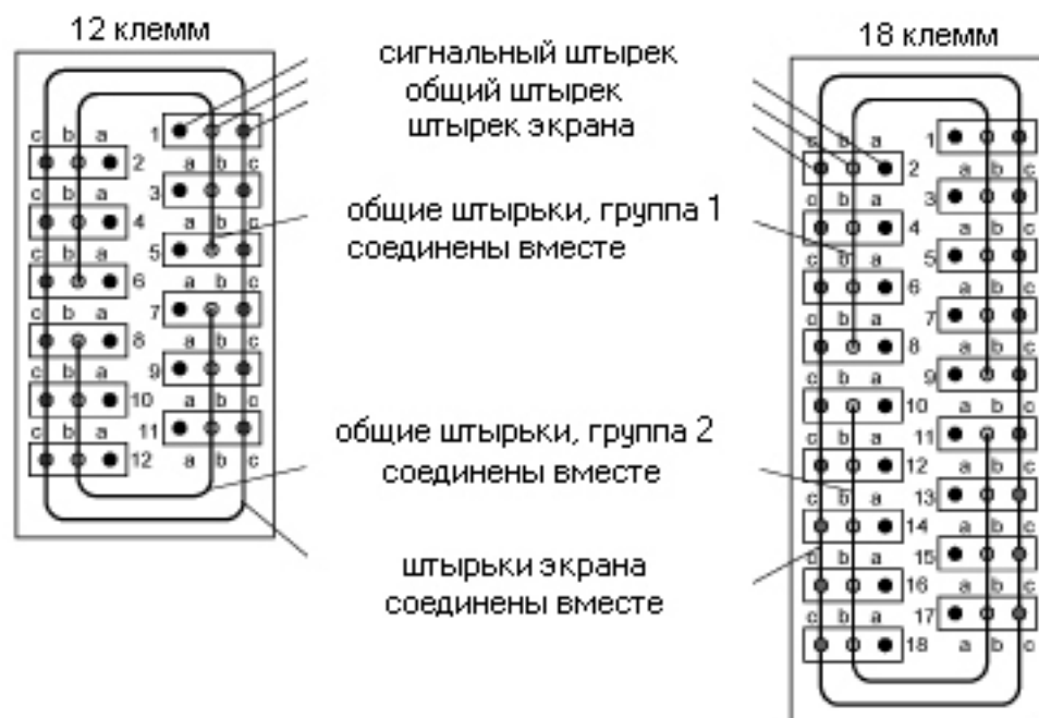
Рисунок 2-10 Схематический рисунок блоков с plug-in клеммами
