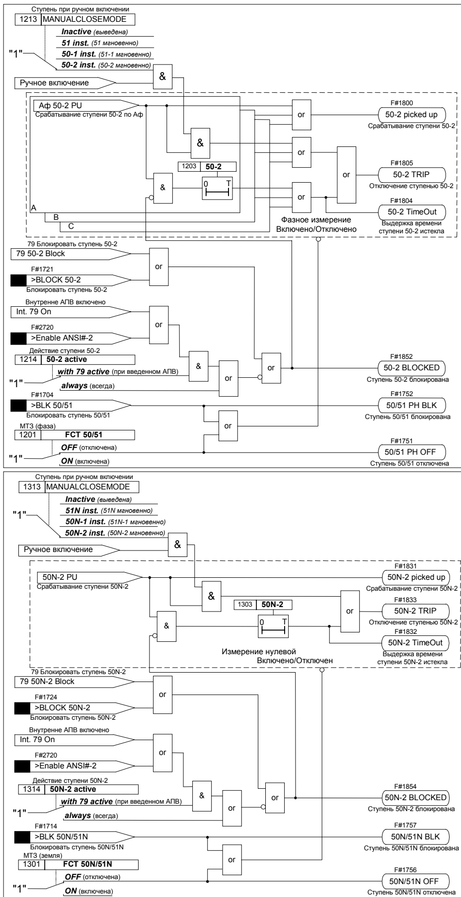
Рисунок 6-11 Схема логики защитных ступеней 50-2 и 50N-2
