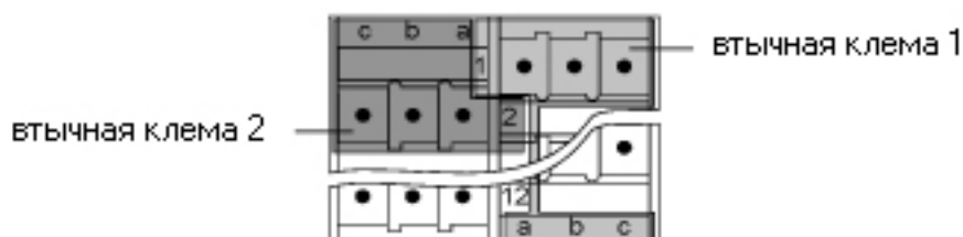
Рисунок 2-9 Соотношение (взаимосвязь) между plug-in клеммами и номерами /буквами подключениям
