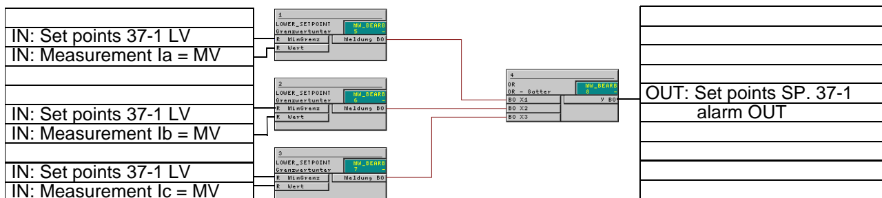
Рисунок A-14 Минимально токовый контроль 37-1
