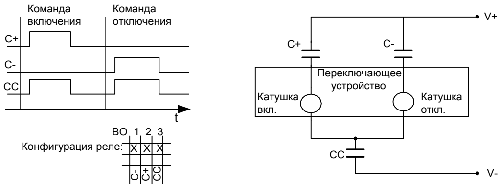
Рисунок 5-6 Двойная команда с одиночными контактами плюс общий контакт
