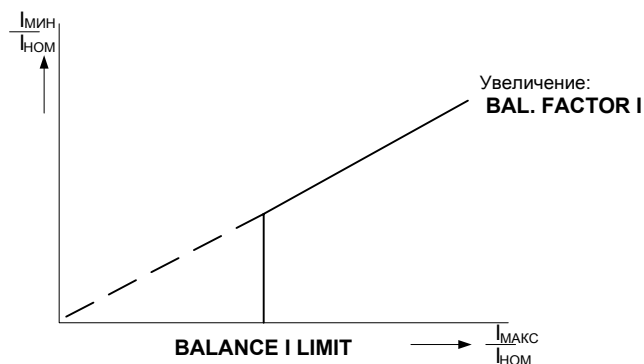
Рисунок 6-42 Контроль симметрии токов
