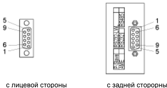
Рисунок 2-13 9-ти штырьковый миниатюрный разъем
