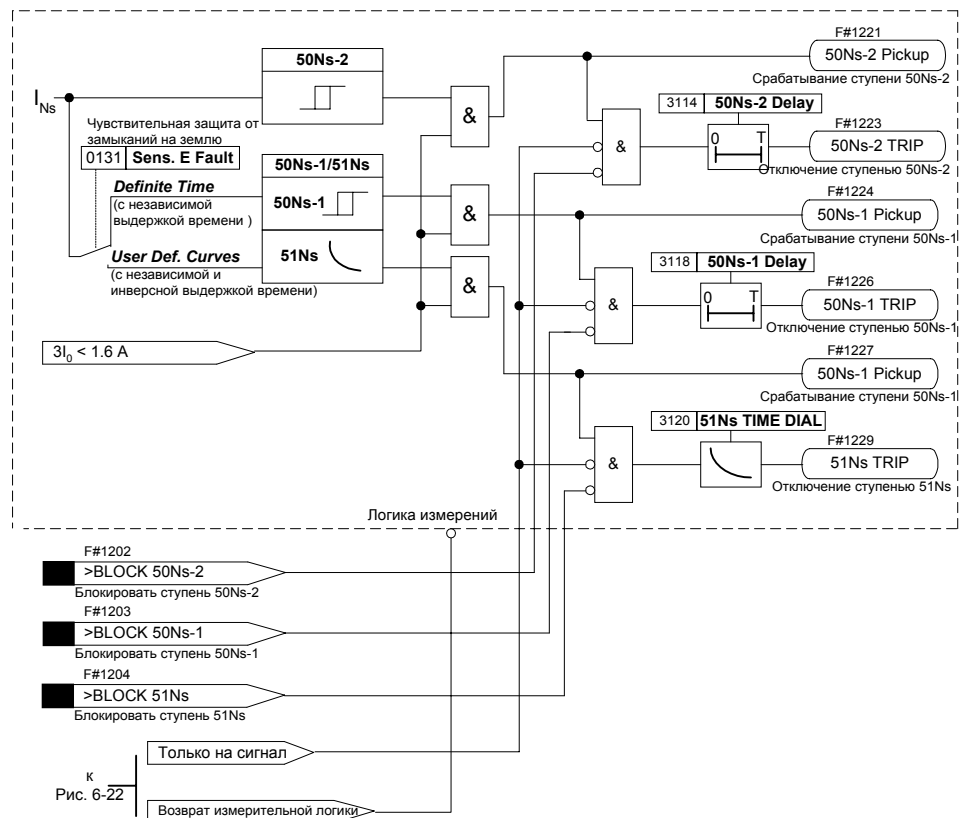
Рисунок 6-23 Схема логики чувствительной защиты от замыканий на землю
