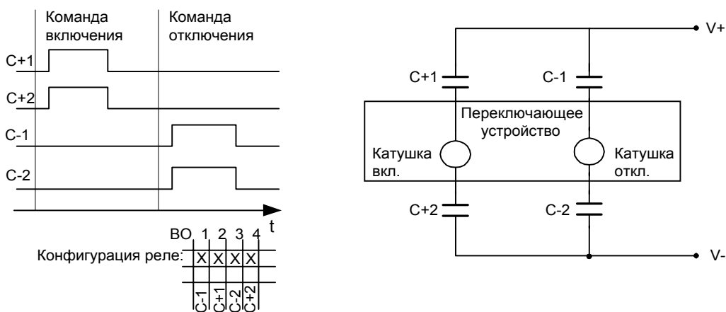
Рисунок 5-8 Двойная команда с двойными контактами (4 реле)
