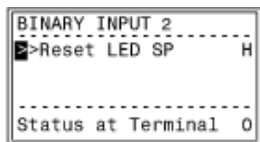
Рисунок 5-27 Выбор бинарного входа 2
