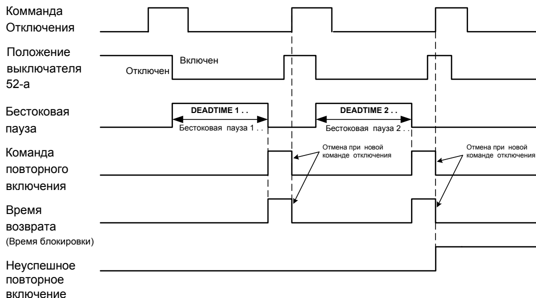
Рисунок 6-37 Временная диаграмма неуспешного двукратного повторного включения
