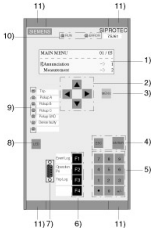
Рисунок 2-1 Передний вид устройства 7SJ61 для установки в шкафу/на панели.
