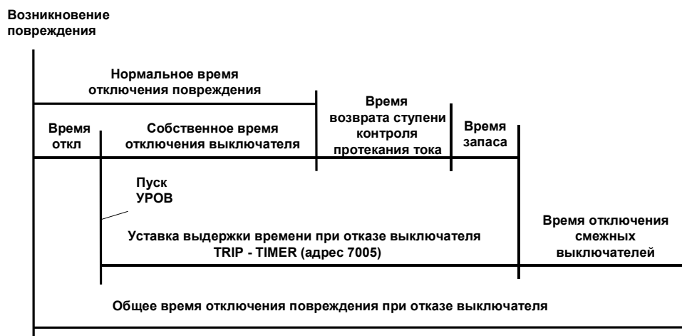
Рисунок 6-35 Временная диаграмма работы защиты при отказе выключателя
