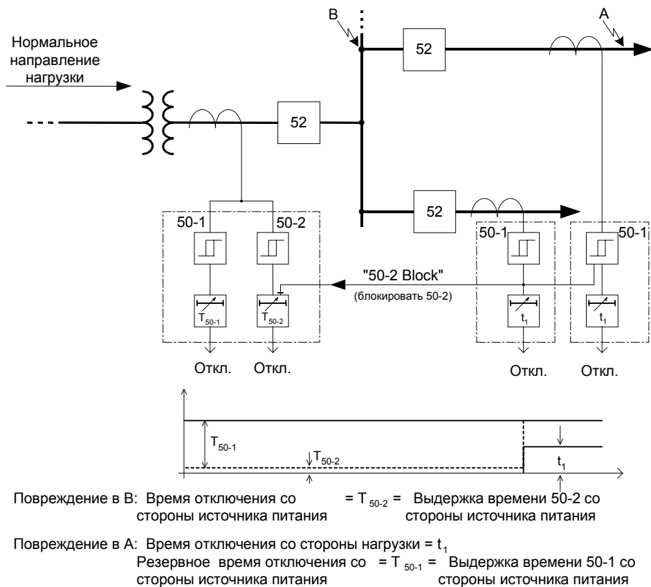
Рисунок 6-14 Схема защиты с обратной блокировкой
