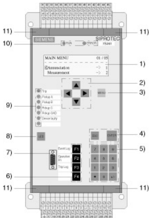
Рисунок 2-14 Передний вид устройства 7SJ61, для навесной установки на панели без оптических интерфейсов
