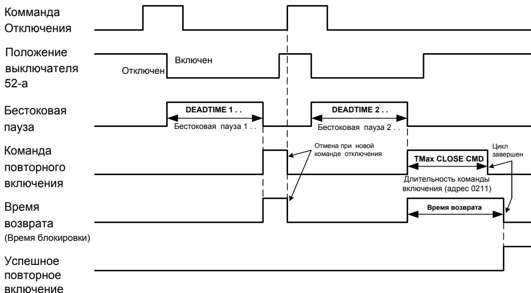
Рисунок 6-36 Временная диаграмма успешного двукратного повторного включения
