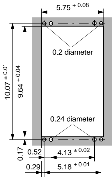
Посадочные размеры
