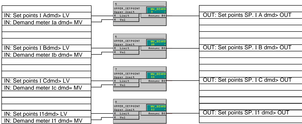
Рисунок А-15 Максимально токовый контроль
