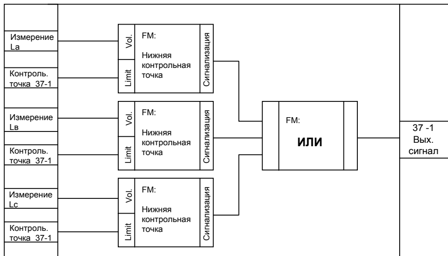
Рисунок 5-38 Контроль понижения тока как пример обработки измерений, определенной пользователем.
