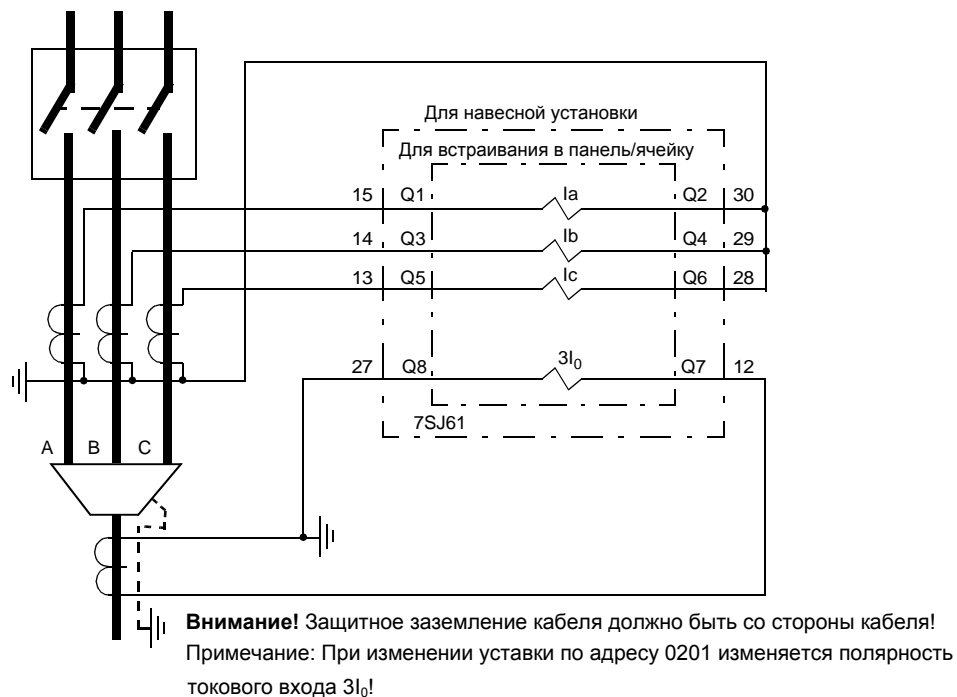
Рисунок А-10. Токовые цепи с тремя трансформаторами тока и трансформатором тока с компенсированным магнитным сердечником в нейтрали для земляного тока. Преимущественно для сетей с эффективным и низкоомным заземлением
