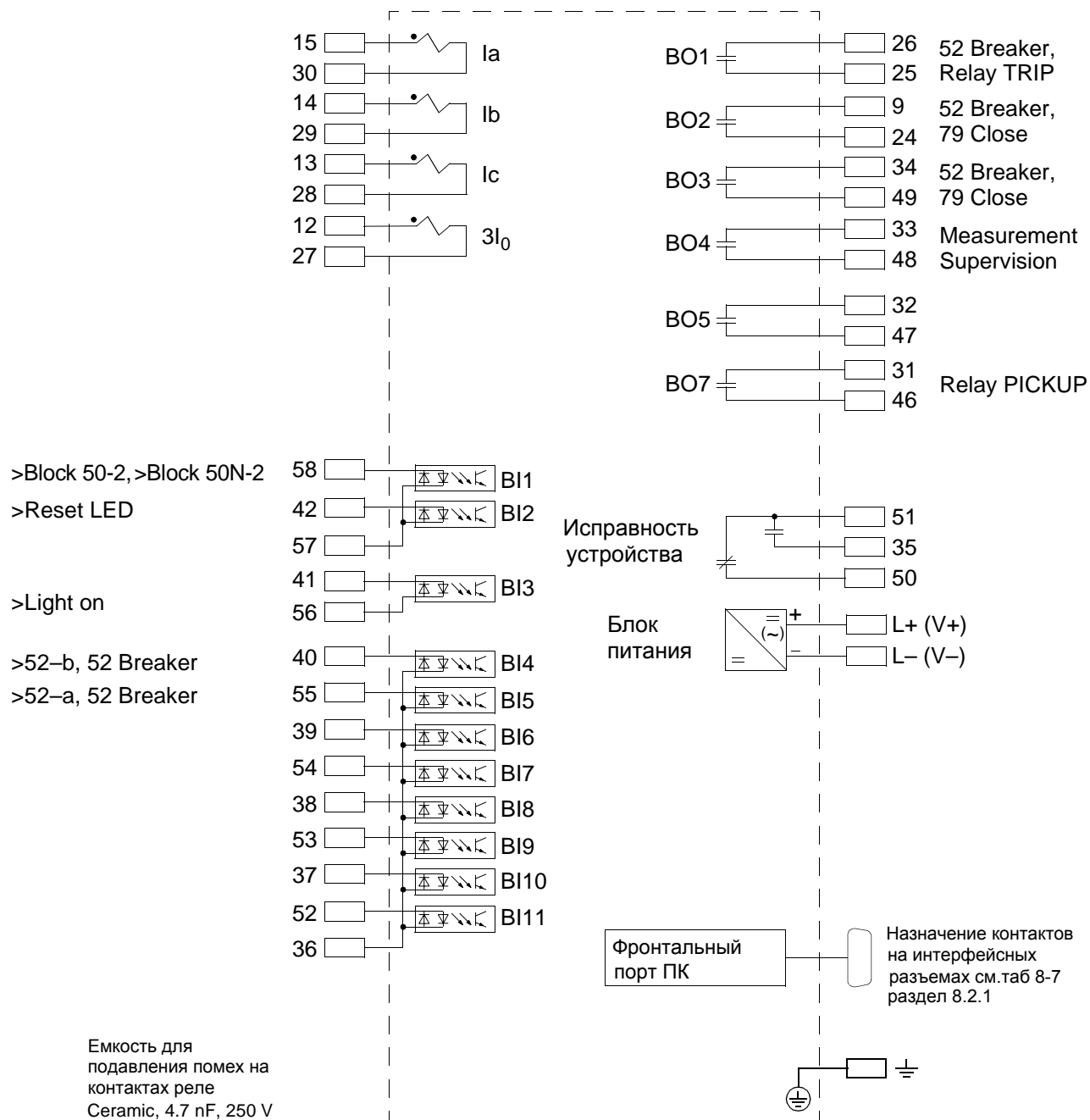
Рисунок А-6 Общая схема 7SJ612*-*B (Установка на панели)
