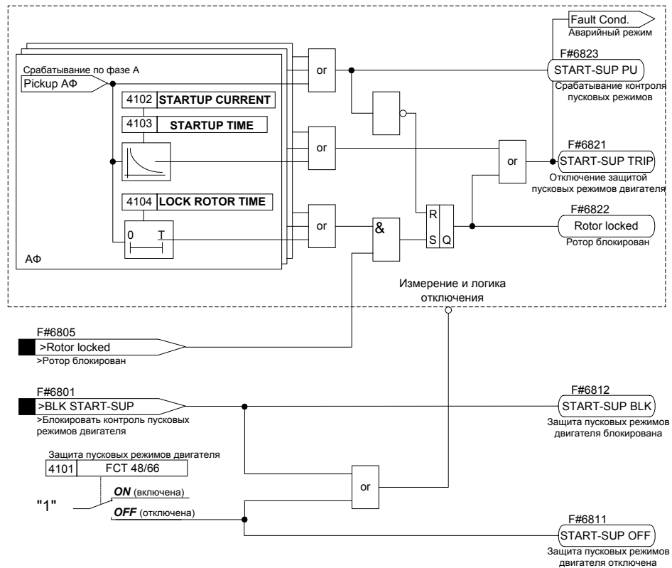
Рисунок 6-29 Схема логики защиты пусковых режимов двигателя
