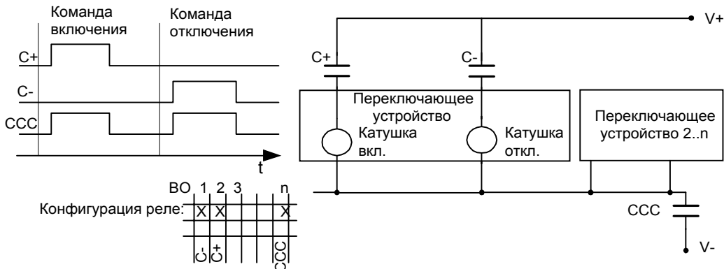
Рисунок 5-7 Двойная команда на общей шине с одиночными контактами и общим контактом
