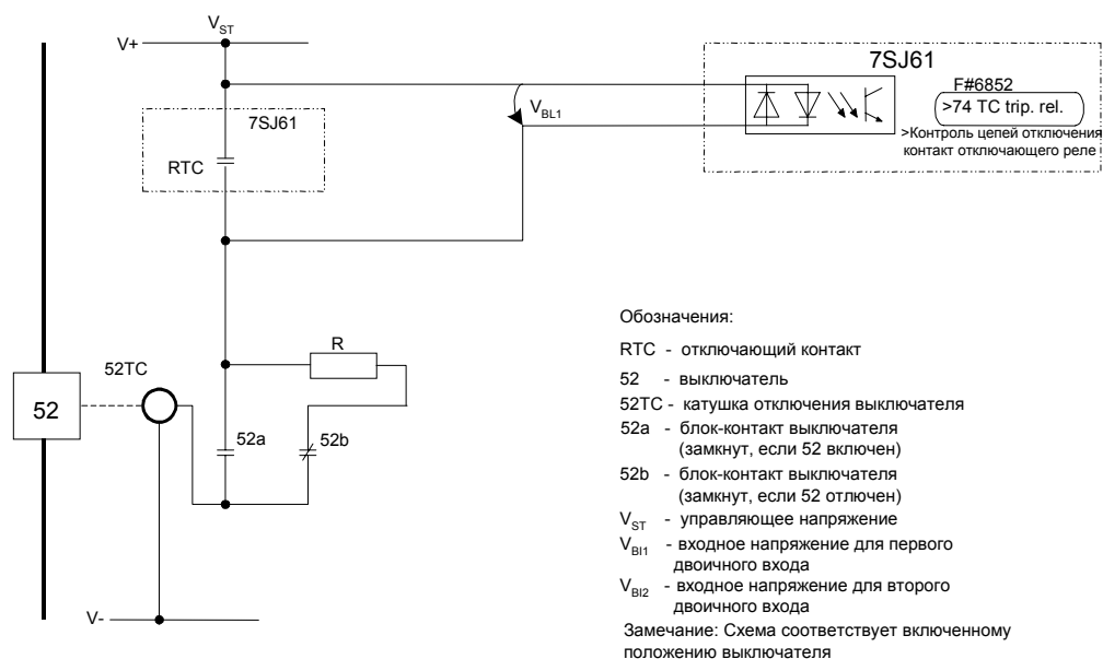
Рисунок 6-45 Контроль цепей отключения с помощью одного двоичного входа
