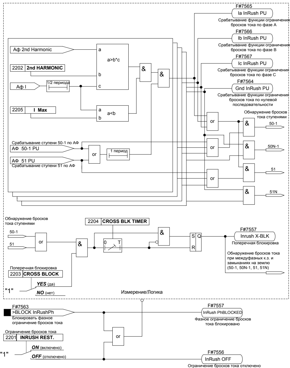
Рисунок 6-21 Схема логики функции ограничения бросков тока
