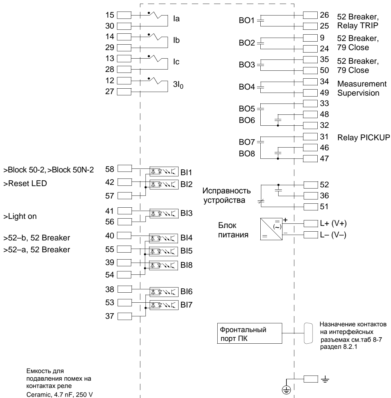
Рисунок А-5 Общая схема 7SJ611*-*B (Установка на панели)
