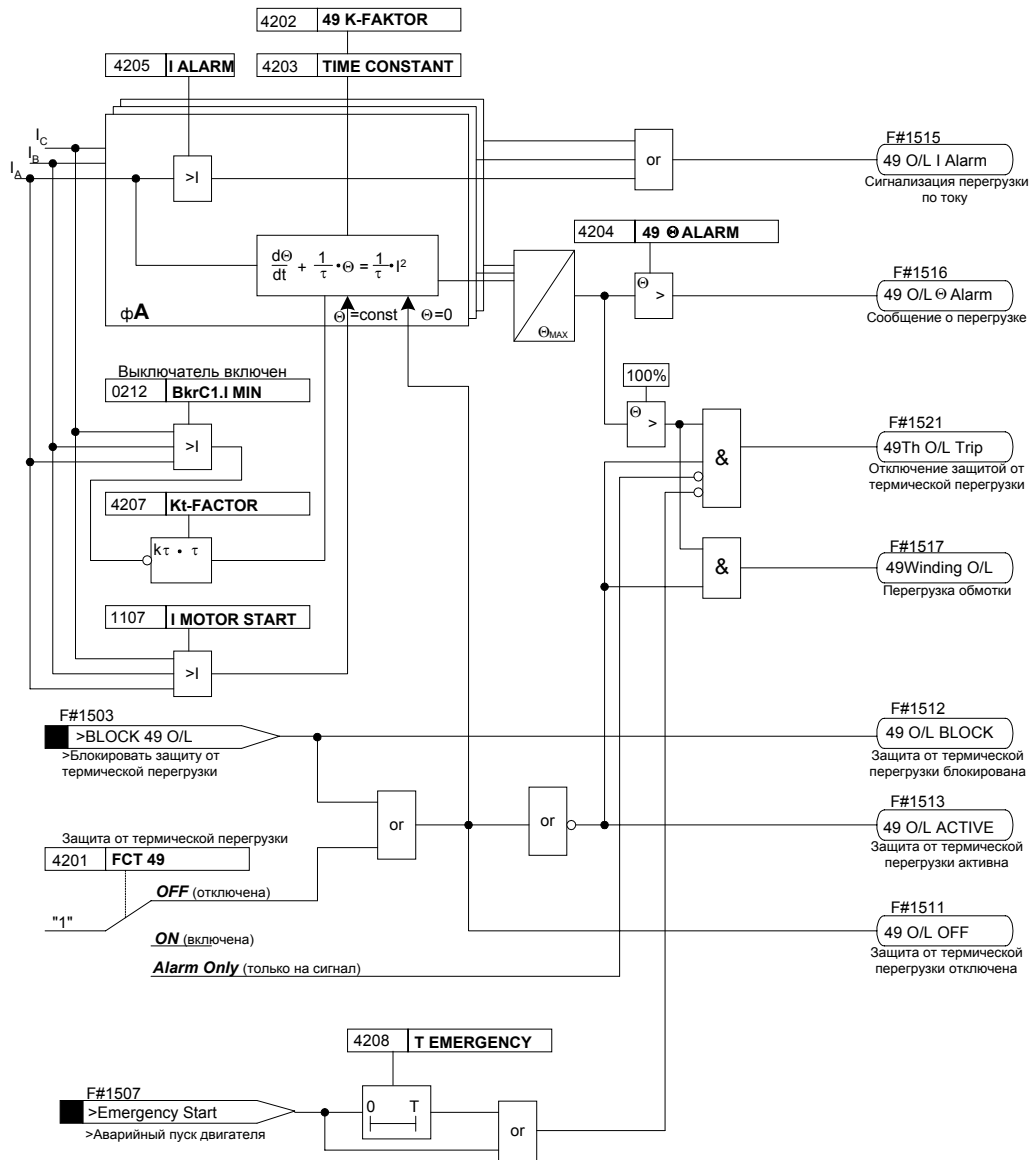
Рисунок 6-30 Схема логики защиты от термической перегрузки.
