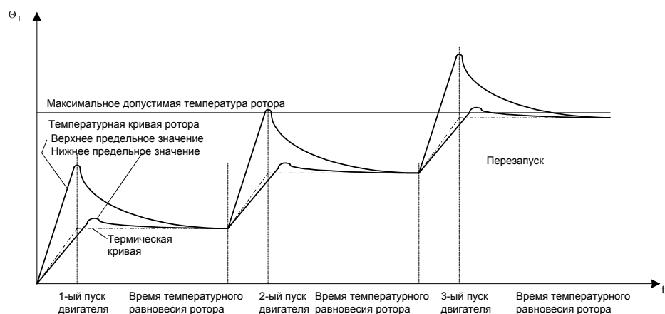
Рисунок 6-31 Термическая модель и температурная кривая ротора при многократных пусках двигателя
