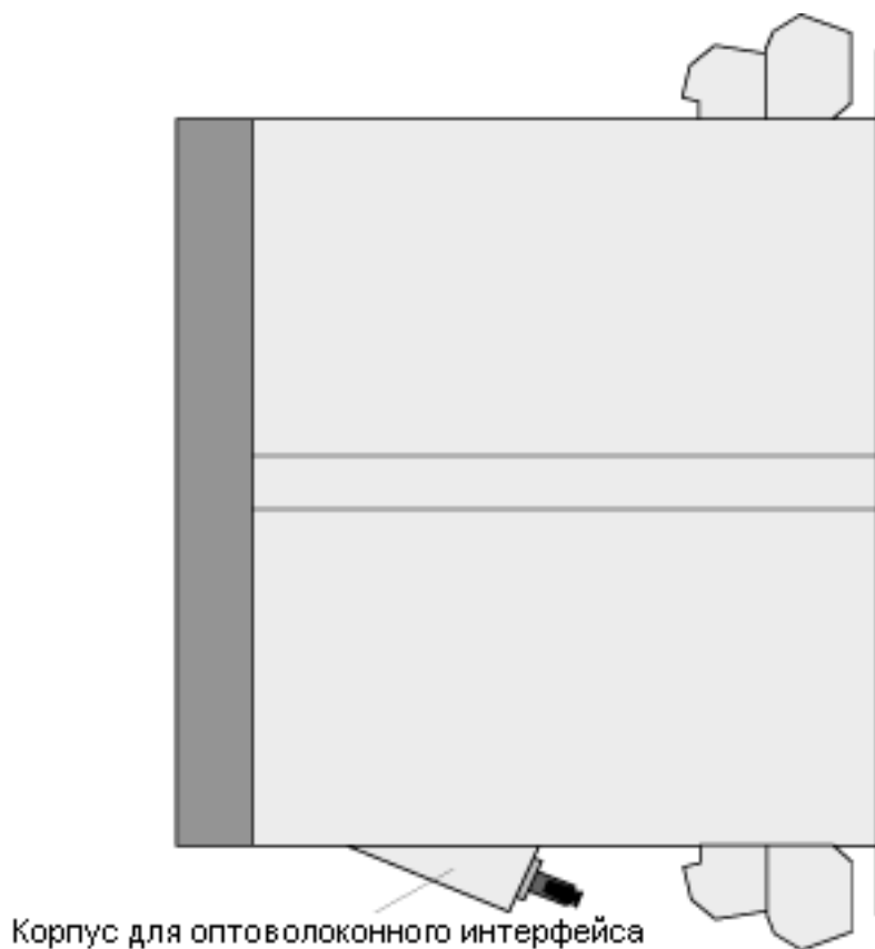
Рисунок 2-15 Вид сбоку устройства 7SJ61 для навесной установки на панели с оптическими интерфейсами
