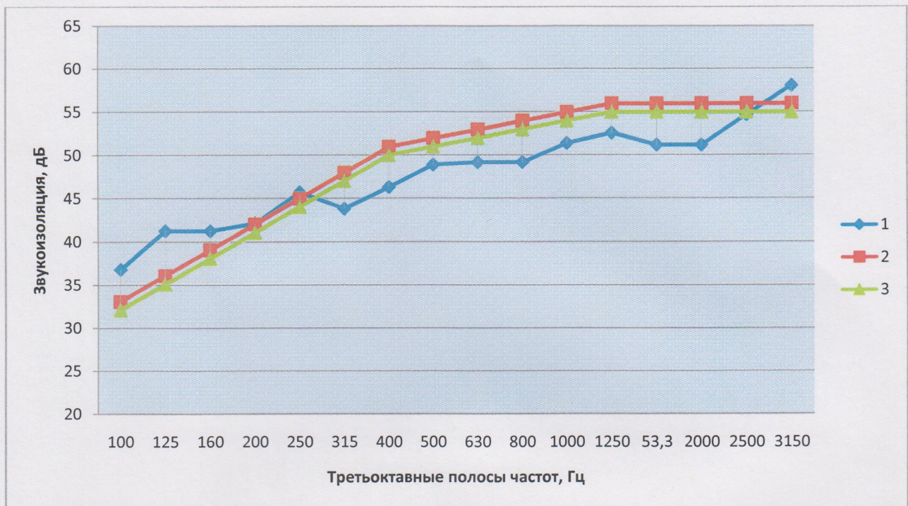
Рисунок 1. Частотная характеристика звукоизоляции 1 - изоляция воздушного шума многослойной конструкции, 2 - нормативная частотная характеристика изоляции воздушного шума, 3 – смещенная нормативная частотная характеристика изоляции воздушного шума на -1 дБ.
