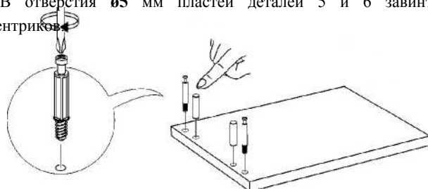
Рис. 3 - Установка шкантов и штоков эксцентриков.
