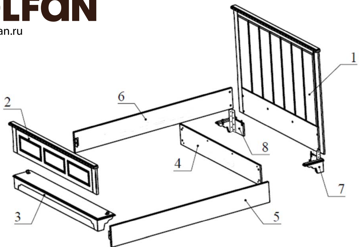
Рис. 2 - Схема сборки.
