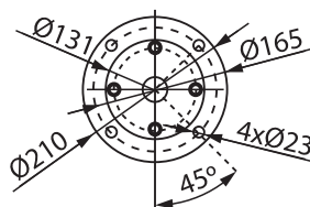
В DN350, 400 ISO 5210 - F16
