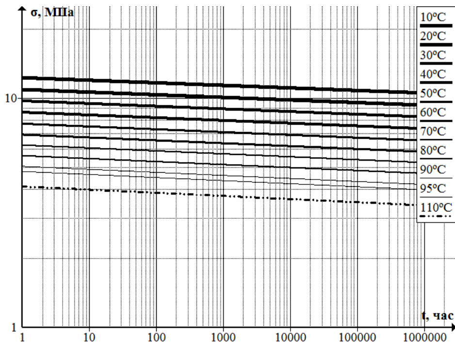
Рисунок 1 – Графики длительной прочности труб PRADO PE-Xa при различных температурах теплоносителя ( \sigma – кольцевые напряжения; t – время работы до разрушения трубы)
