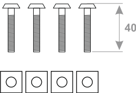
M6x40
