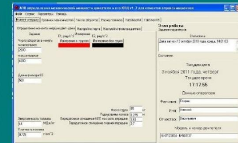
Интерфейс программной части аппаратно-программного комплекса контроля параметров колесных машин, оснащенных ДВС с искровым зажиганием
