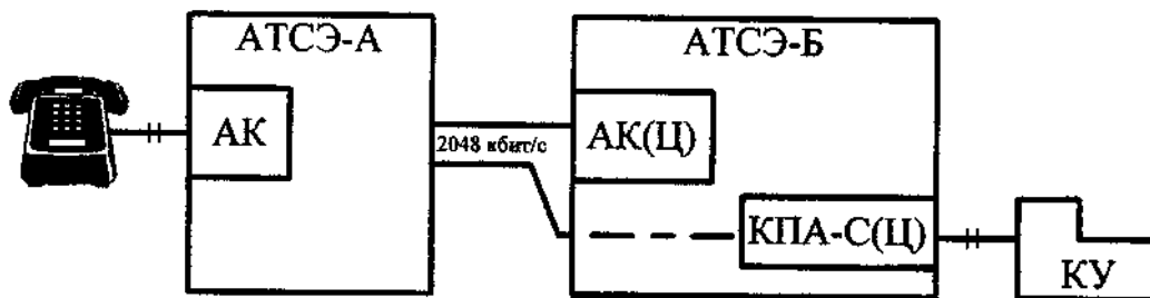
Рис. 6.5. Реализация на АТСЭ-Б цифрового абонентского комплекта для подключения прямого абонента
