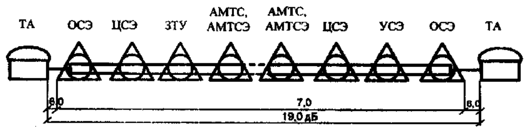
Рисунок Б.11 - Распределение норм затухания при междугородной связи для абонентов СТС
