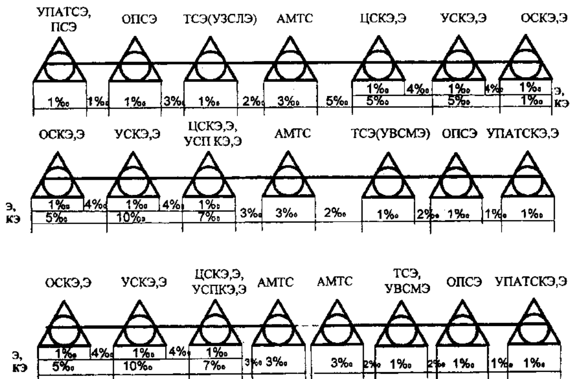
Рисунок А.3 - Максимально допустимые потери при внутризональной связи ГТС с СТС
