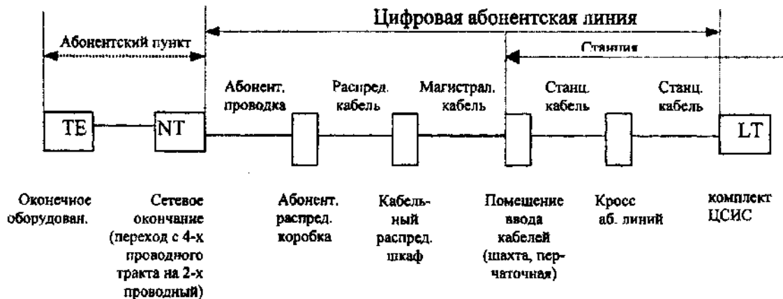
Рисунок 9.1 - Структура цифровой абонентской линии с ЦСИС (АЛЦ) 2В+D.
