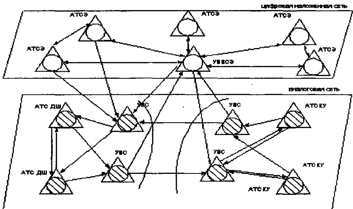
Рисунок 6.2 - Структура аналого-цифровой сети с узлами входящих сообщений
