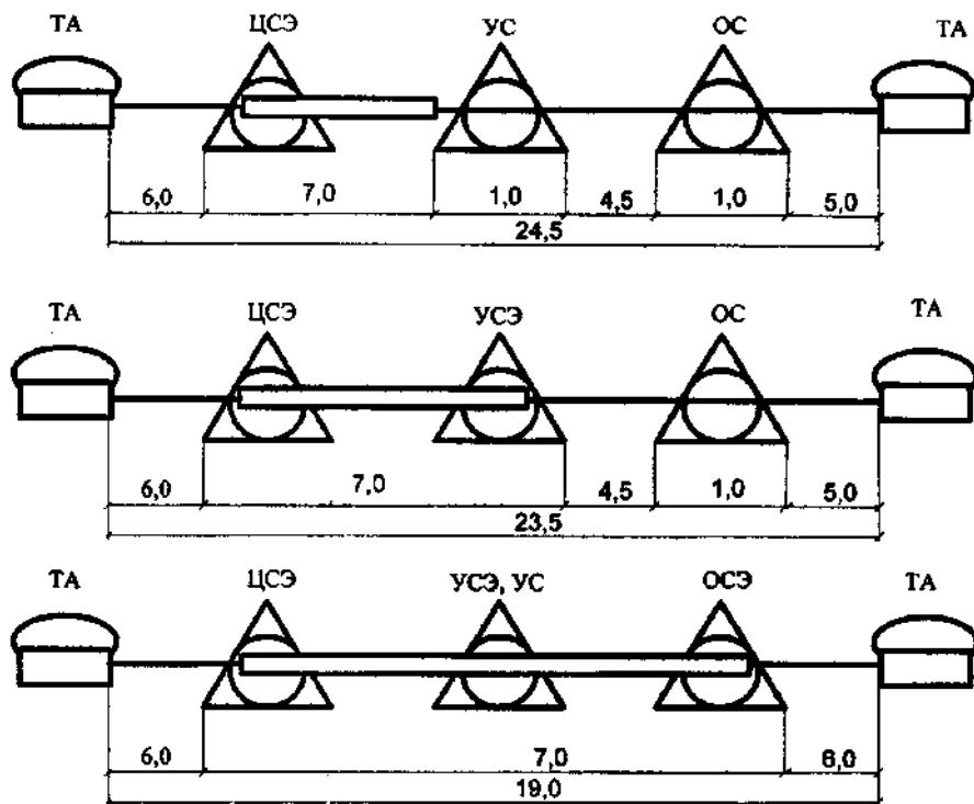
Рисунок Б.10 - Распределение норм затухания на СТС при двухступенчатом радиально-узловом построении, лист 1
