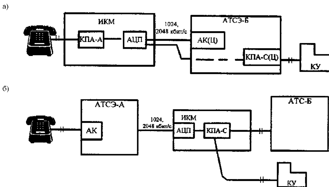
Рисунок 6.6. Реализации на АТСЭ абонентского (КПА-А) и стационарного (КПА-С) окончаний для подключений прямого абонента
