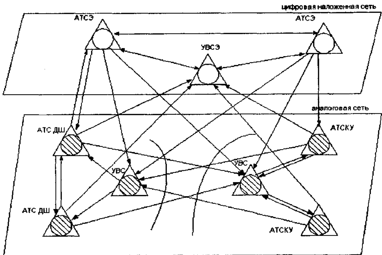
Рисунок 6.2 - Структура аналого-цифровой сети с узлами входящих сообщений
