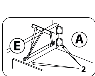
Крепление подъемного механизма к боковым царгам (газлифт крепится к подъемному механизму цилиндром вверх как на схеме)
