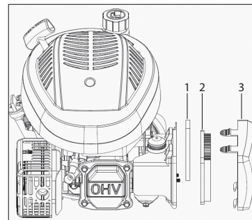
Рис.9. Воздушный фильтр:
