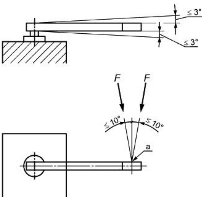
Рисунок 2 - Ключ в горизонтальном положении
