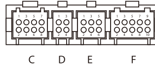
Схема разъемов подключения.
