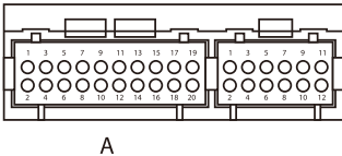
Схема разъемов подключения.
