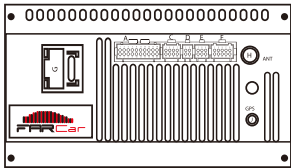
Схема распиновки разъемов устройства.
