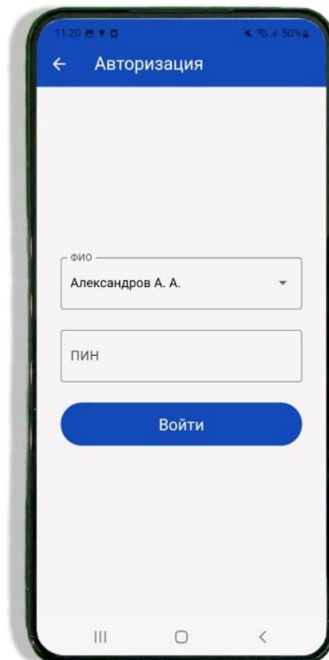
Рис. 5. Окно авторизации
