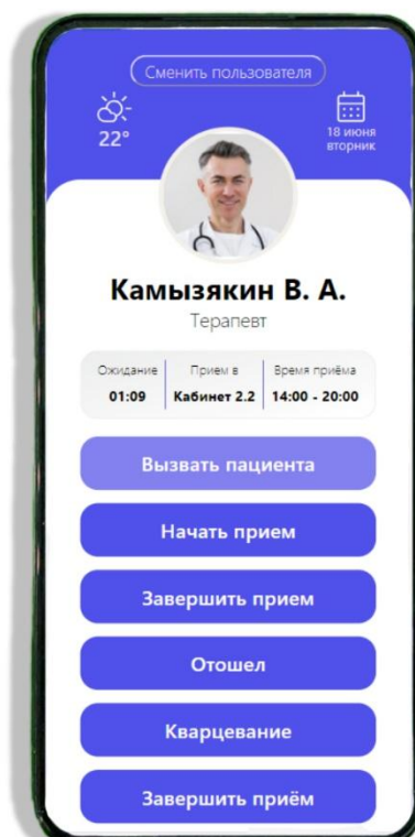
Рис. 6. Главная страница
