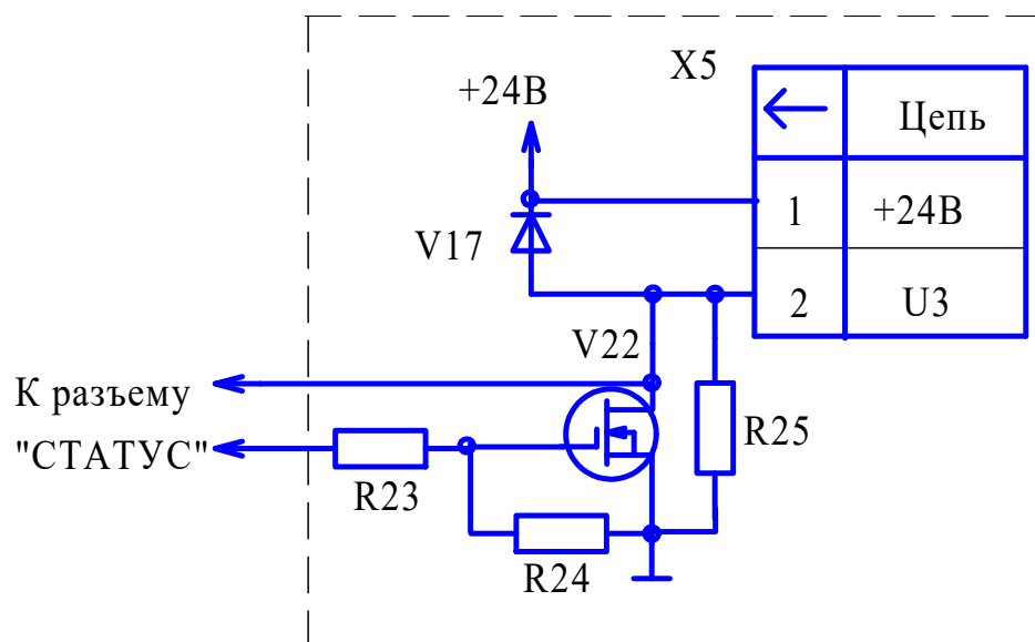
Рисунок 1.2 - Схема электрическая принципиальная формирователя сигнала СТАТУС
