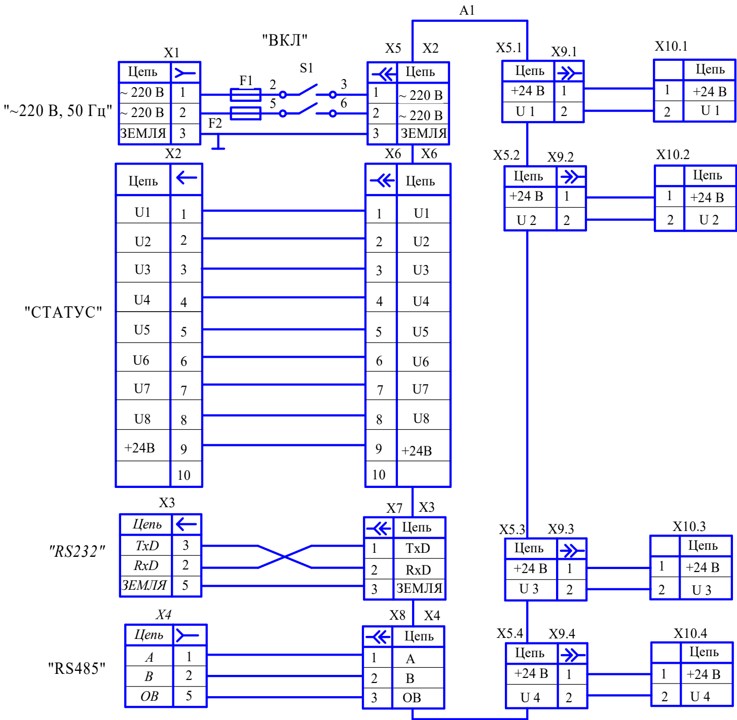
Распределитель газовый РГМ-4. Схема электрическая соединений
