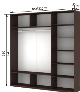
Внутренняя компоновка 3-х дверного шкафа Габаритные размеры указаны с учетом фасадов
