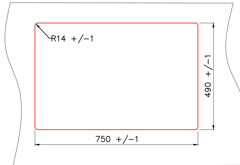
Врезной монтаж мойки (I)
