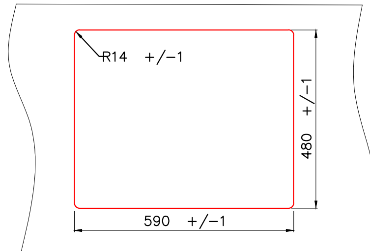
Врезной монтаж мойки (I)
