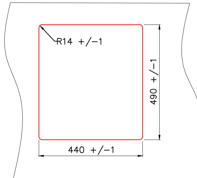
Врезной монтаж мойки (I)
