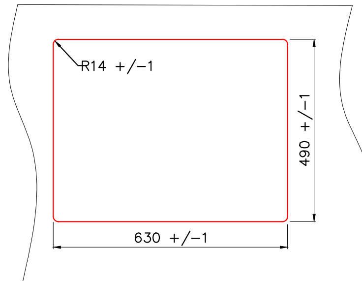
Врезной монтаж мойки (I)
