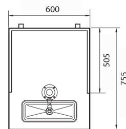
ВИД СВЕРХУ
