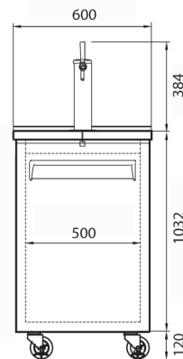
ВИД СПЕРЕДИ
