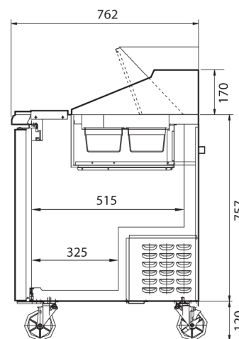
ВИД СБОКУ
