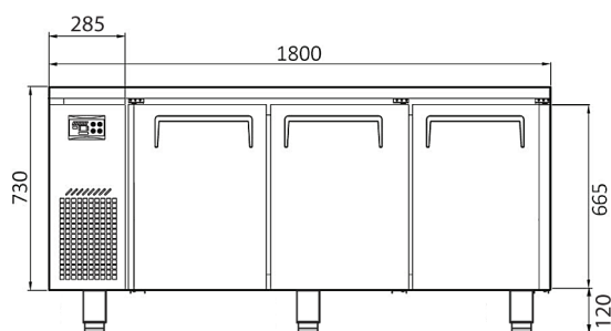
ВИД СПЕРЕДИ
