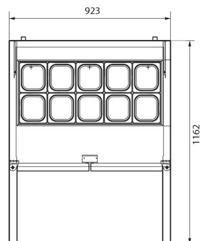
ВИД СВЕРХУ
