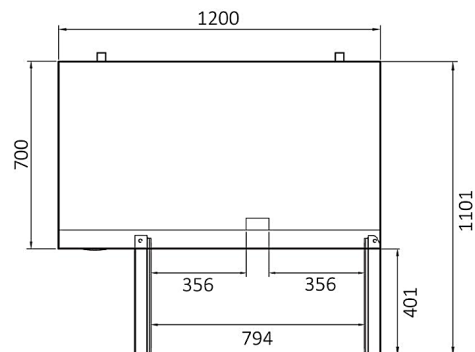
ВИД СВЕРХУ
