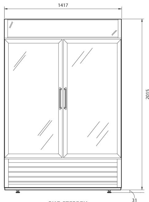
ВИД СПЕРЕДИ
