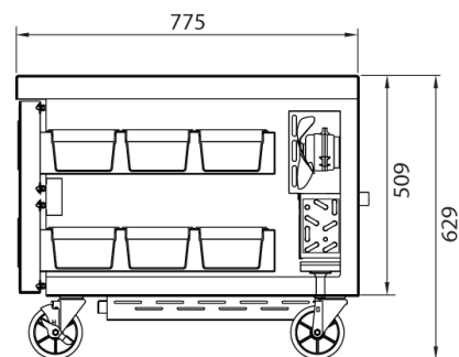
ВИД СБОКУ
