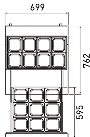
ВИД СВЕРХУ
