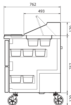
ВИД СБОКУ
