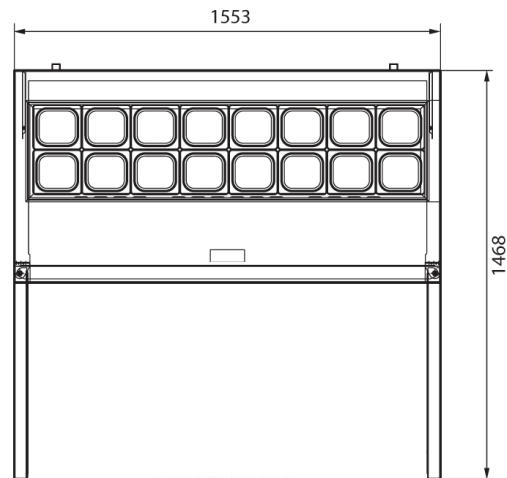
ВИД СВЕРХУ
