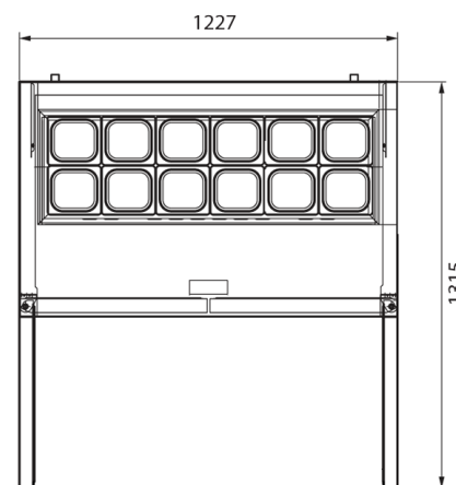
ВИД СВЕРХУ
