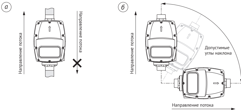
Рис. 4. Способы установки блока: а) относительно направления потока; б) относительно горизонтали
